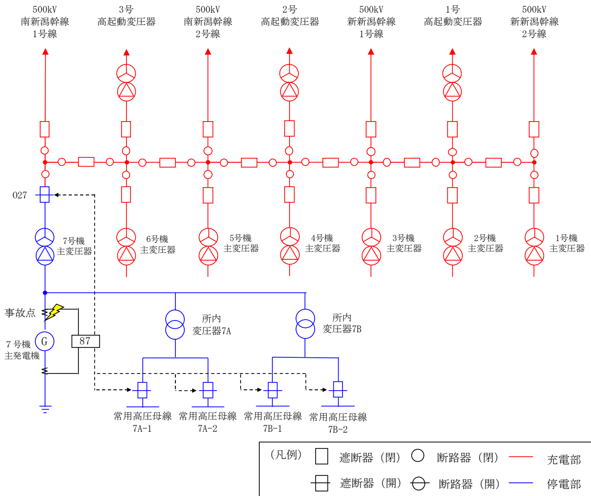
図 7 発電機保護
