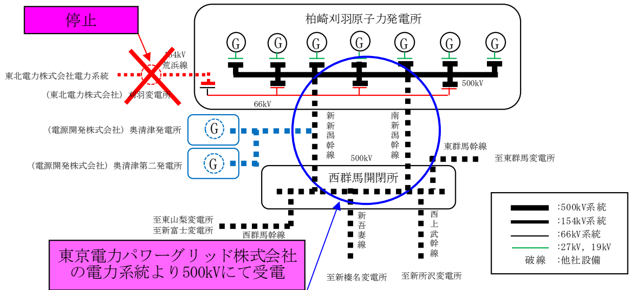
図3 刈羽変電所全停電時の供給系統
