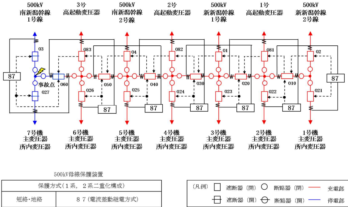
(a) 500kV 超高压開閉所 7号機が接続する母線故障時
