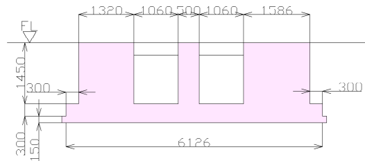
a-a' 断面
