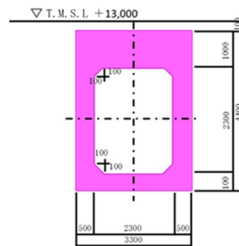
a-a' 断面
