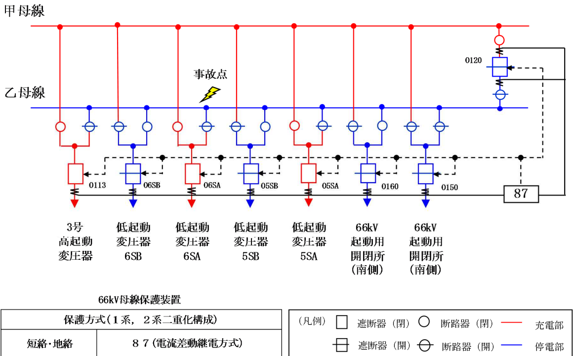
(b) 66kV 起動用開閉所 (北側) 乙母線故障時
