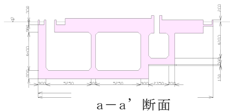
(a) 500kV 超高压開閉所基礎構造図
