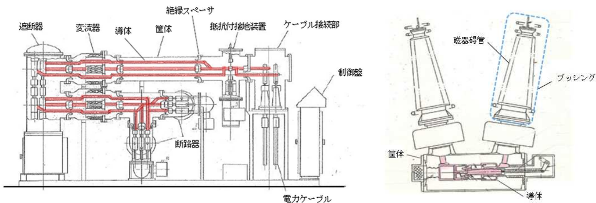
(a) 500kV ガス絶縁開閉装置
