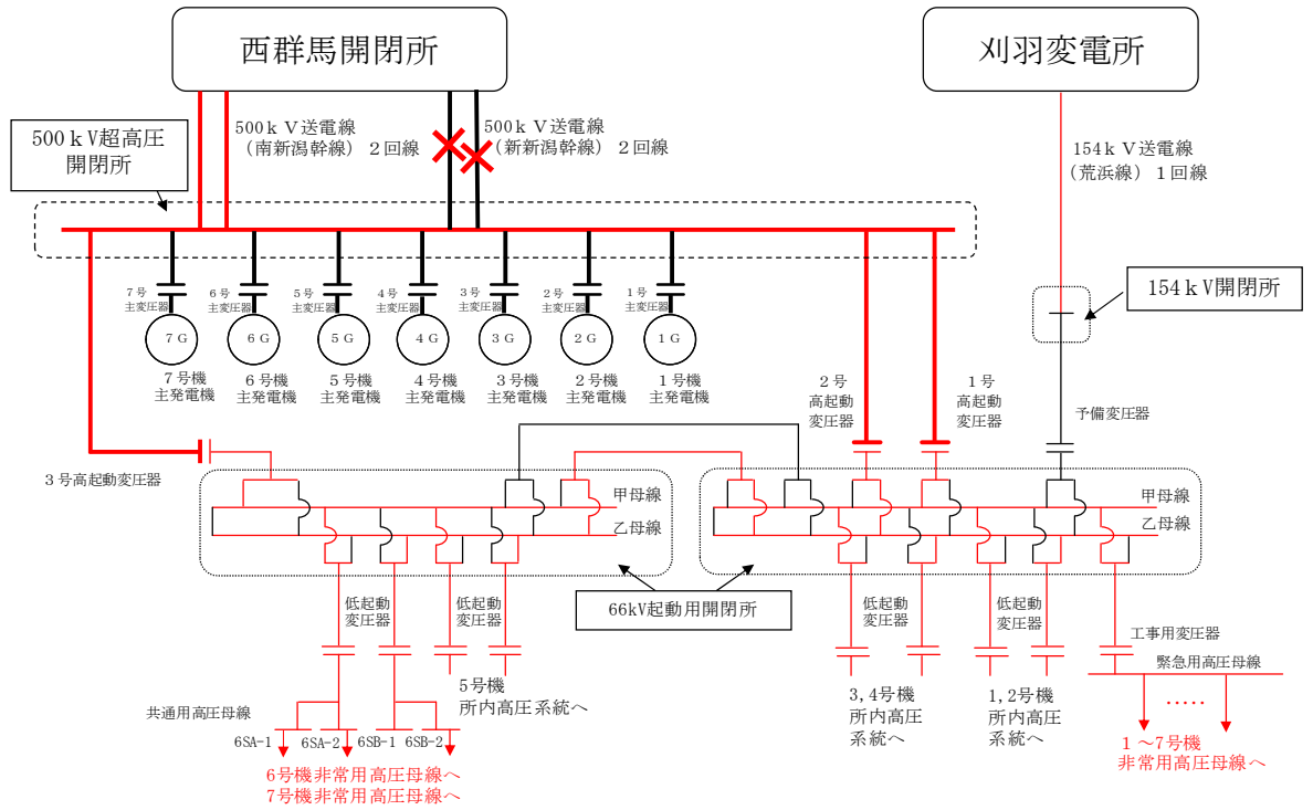
(a) 500kV 新新潟幹線 2 回線 停電時
