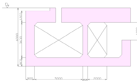
a-a' 断面
