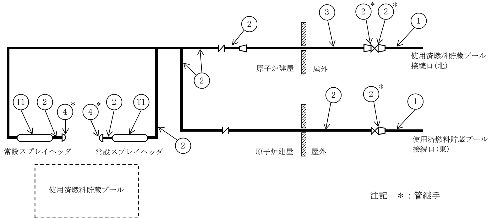
燃料プール代替注水系概略系統図 (その1)
