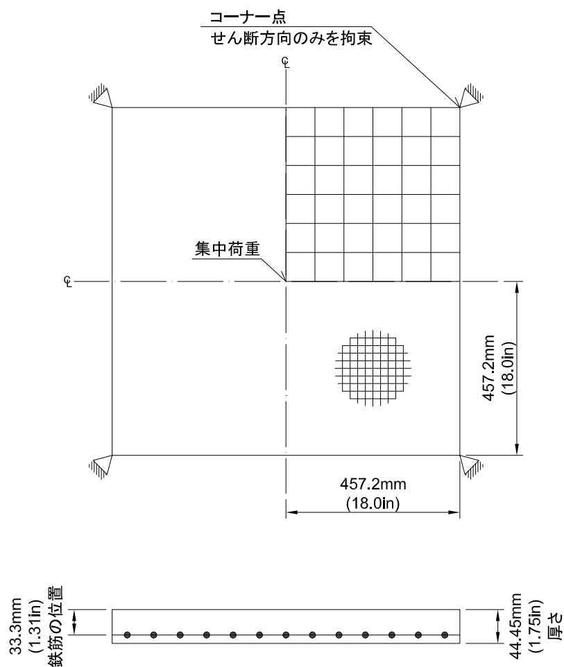
図 3-2 解析モデル
