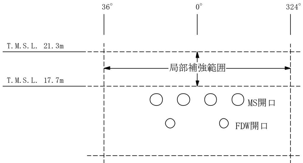
図 5-7 局部補強範囲
