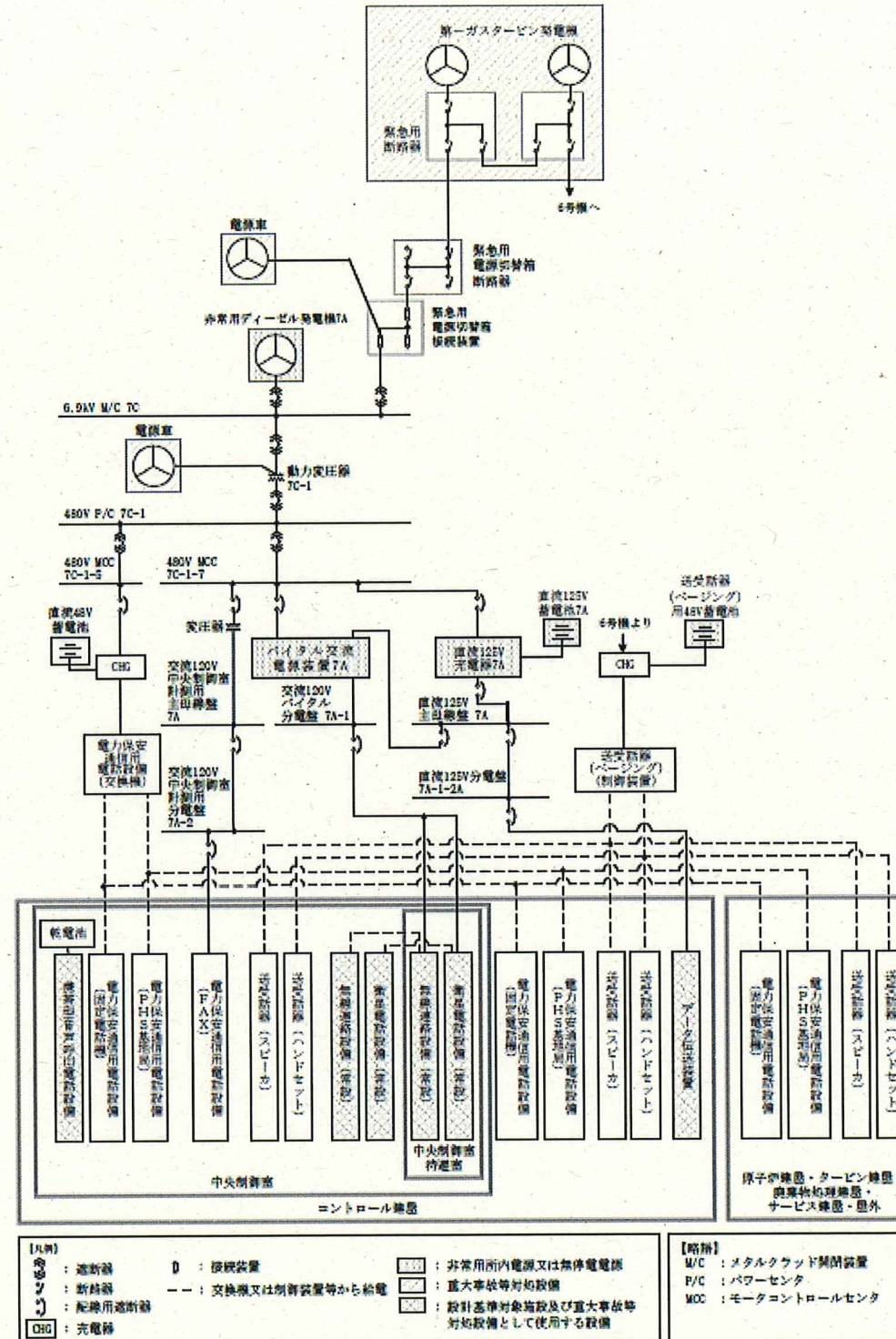
図1 通信連絡設備の電源概略構成図 (1/2)
