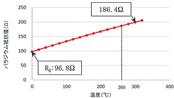
図5 パラジウム抵抗特性グラフ (水素濃度: 0vol%時)
