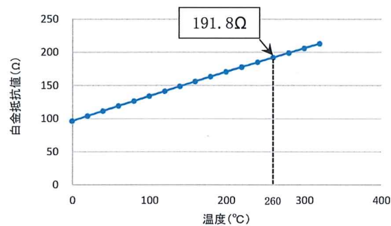
図4 白金抵抗特性グラフ (水素濃度: 0vol%時)
