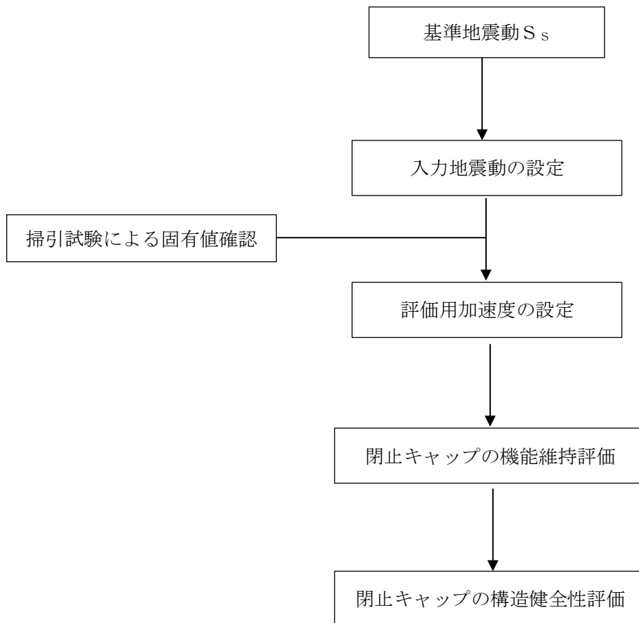
図2-3 耐震評価フロー
