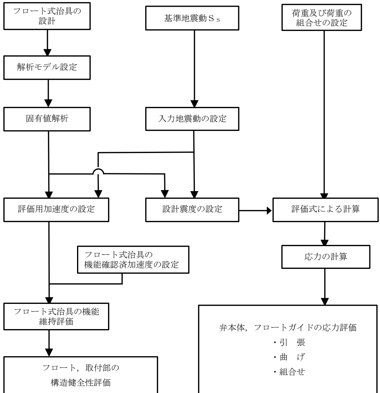
図2-1 耐震評価フロー
