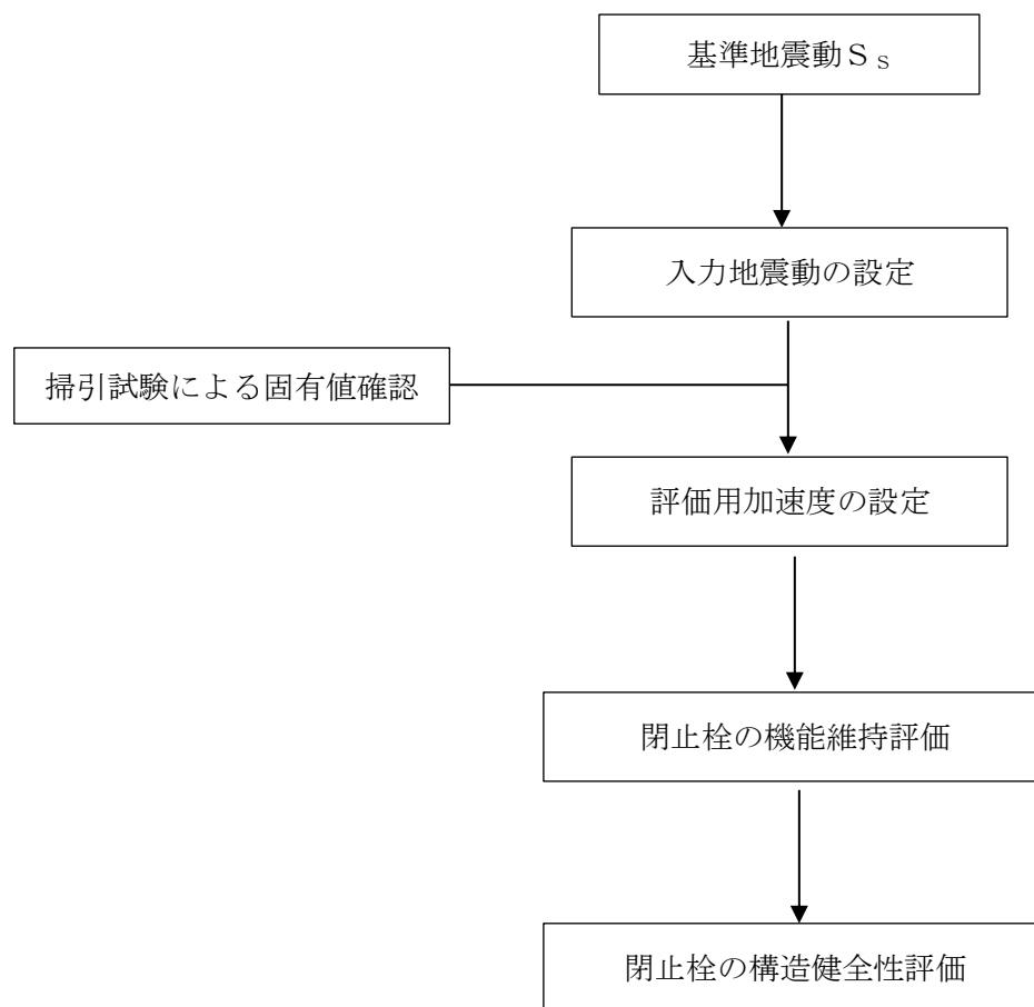
図2-4 耐震評価フロー
