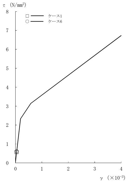
図2-123 τ - γ 関係と最大応答値 (Sd-8, EW方向, 4F) (2/8)
