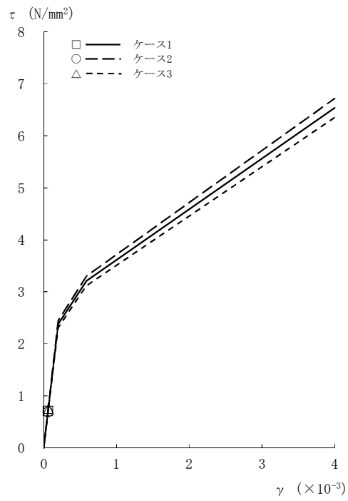
図2-39 τ - γ 関係と最大応答値 (Sd-3, NS方向, 4F) (2/8)
