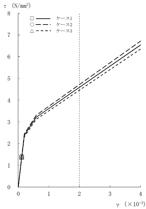
図2-19 \tau - \gamma 関係と最大応答値 (Ss-2, NS方向, 4F) (2/8)
