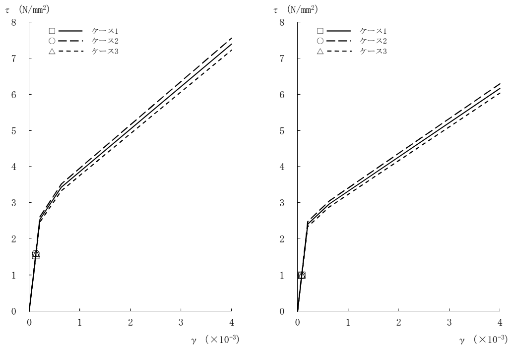
図2-41 τ - γ 関係と最大応答値 (Sd-1, EW方向, B1F) (6/8)
