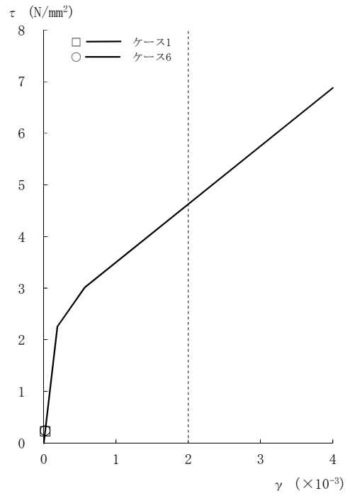
図2-102 \tau - \gamma 関係と最大応答値 (Ss-3, NS方向, 3F) (3/8)
