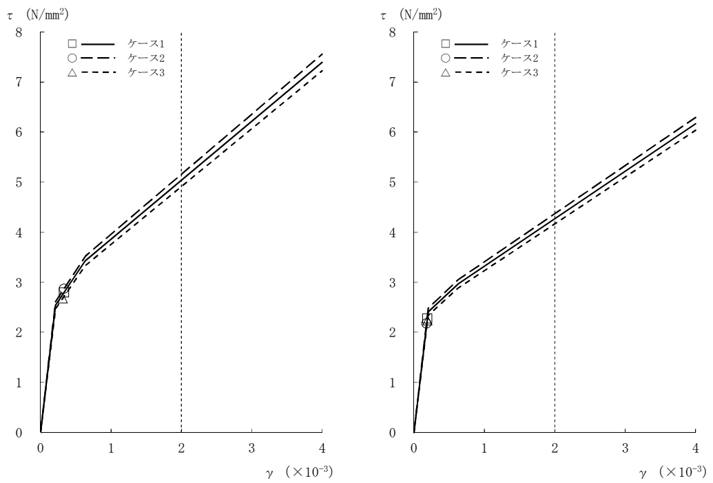
図2-22 τ - γ 関係と最大応答値 (Ss-1, EW方向, B1F) (6/8)
