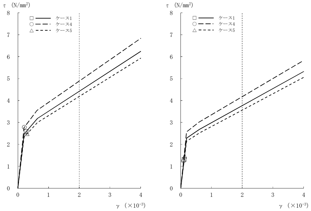
図2-64 τ - γ 関係と最大応答値 (Ss-2, EW方向, 1F) (5/8)
