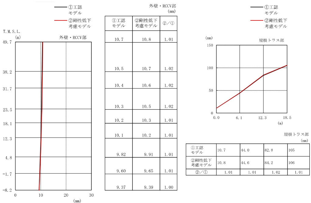
図 3-13 最大応答変位 (Ss-1, 鉛直方向)
