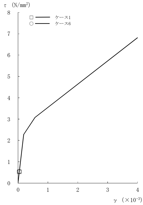
図2-117 τ - γ 関係と最大応答値 (Sd-2, NS方向, CRF) (1/8)
