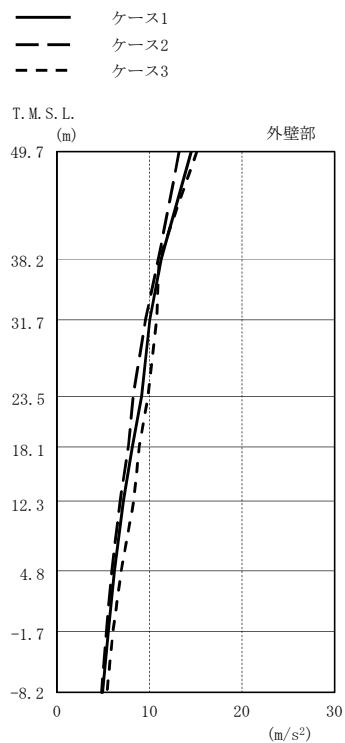
図2-1 最大応答加速度 (基準地震動 S s , NS方向) (2/2)
