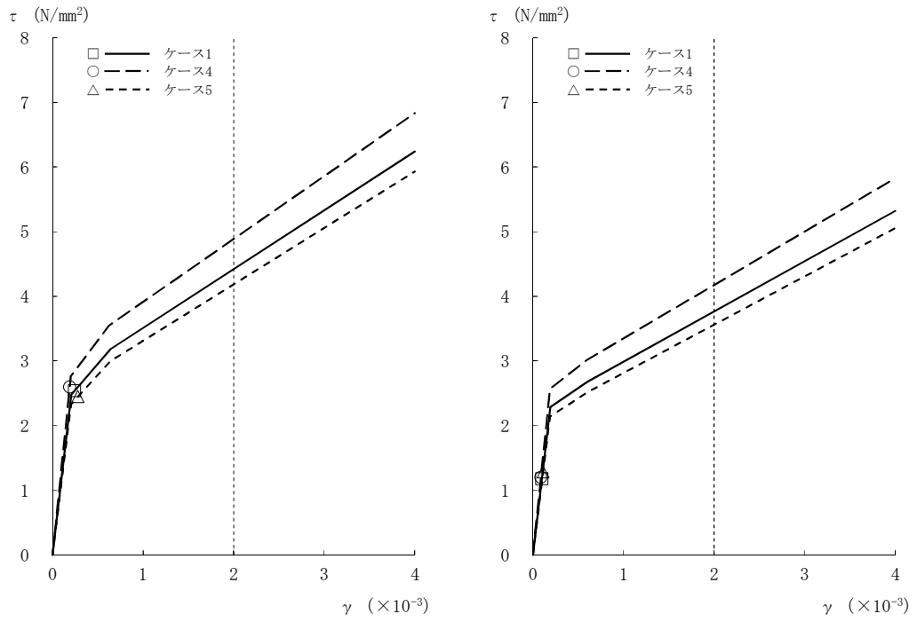
図2-63 \tau - \gamma 関係と最大応答値 (Ss-1, EW方向, 1F) (5/8)
