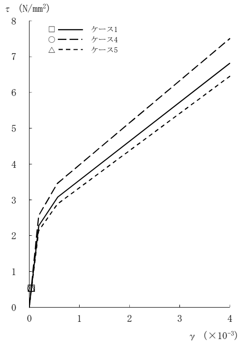
図2-79 τ - γ 関係と最大応答値 (Sd-2, NS方向, CRF) (1/8)
