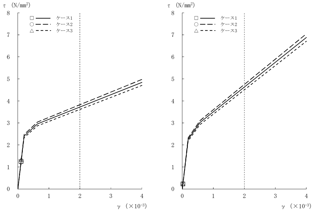
図2-20 τ - γ 関係と最大応答値 (Ss-3, NS方向, 3F) (3/8)
