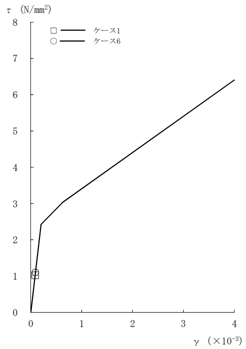
図2-116 τ - γ 関係と最大応答値 (Sd-1, NS方向, B1F) (6/8)
