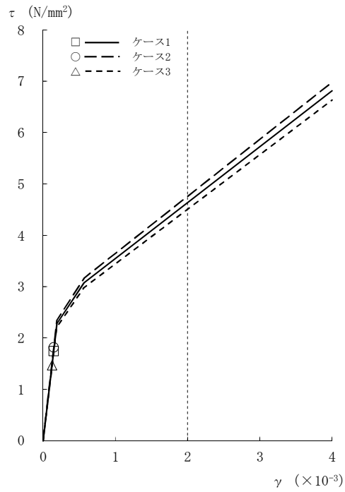
図2-18 τ - γ 関係と最大応答値 (Ss-1, NS方向, CRF) (1/8)
