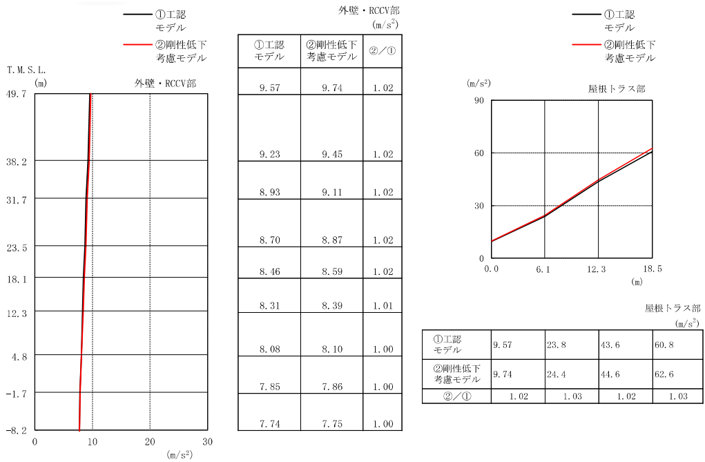
図 3-12 最大応答加速度 (Ss-1, 鉛直方向)
