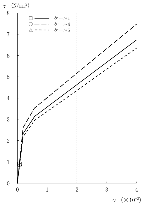
図2-65 τ - γ 関係と最大応答値 (Ss-3, EW方向, 4F) (2/8)
