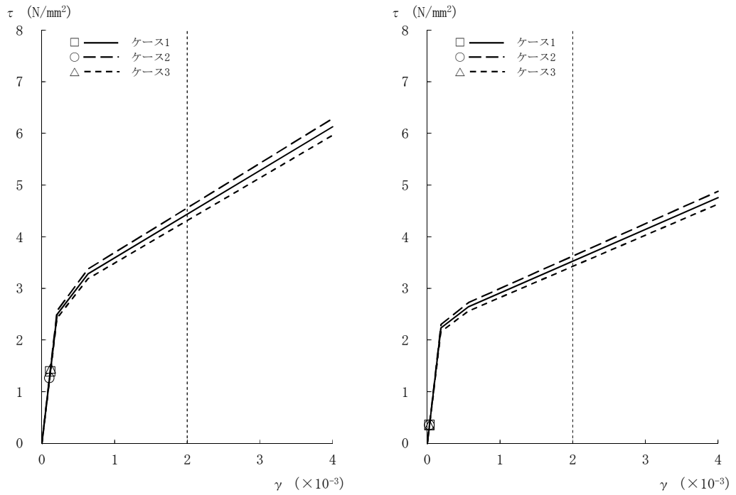
図2-25 \tau - \gamma 関係と最大応答値 (Ss-8, EW方向, 3F) (3/8)
