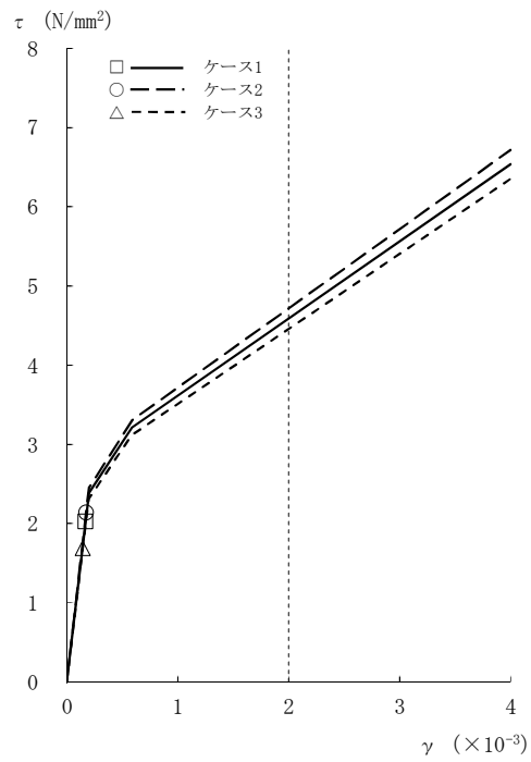
図2-18 τ - γ 関係と最大応答値 (Ss-1, NS方向, 4F) (2/8)
