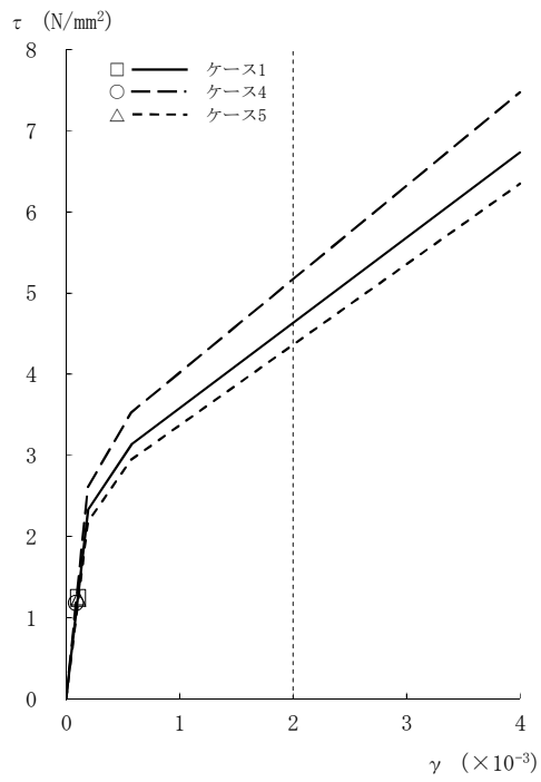
図2-64 τ - γ 関係と最大応答値 (Ss-2, EW方向, 4F) (2/8)
