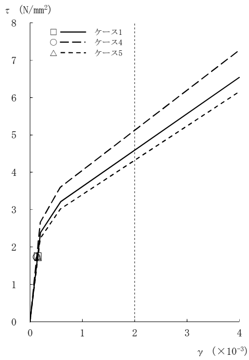
図2-62 τ - γ 関係と最大応答値 (S s -8, NS方向, 4F) (2/8)
