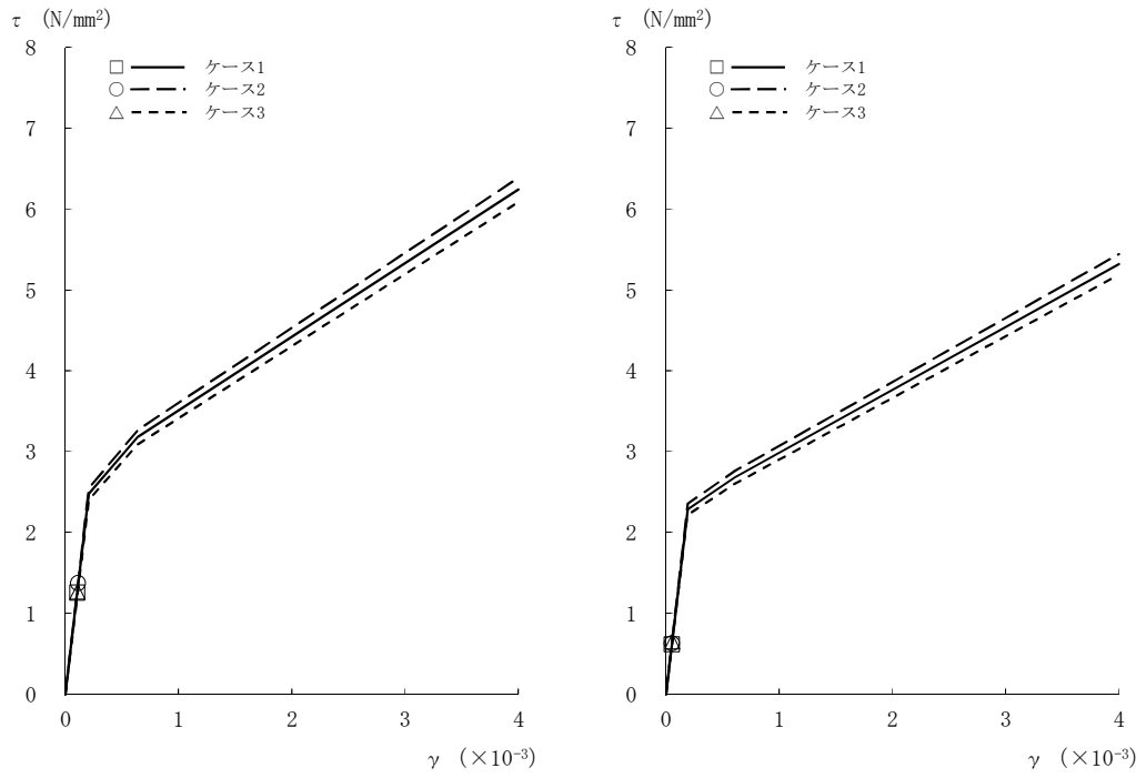
図2-41 τ - γ 関係と最大応答値 (Sd-1, EW方向, 1F) (5/8)
