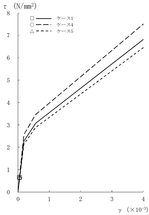
図2-81 τ - γ 関係と最大応答値 (Sd-8, NS方向, CRF) (1/8)
