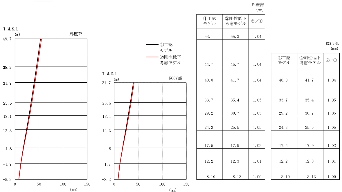
図 3-9 最大応答変位 (Ss-1, EW 方向)
