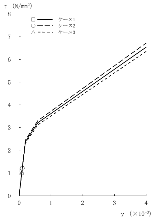
図2-37 \tau - \gamma 関係と最大応答値 (Sd-1, NS方向, 4F) (2/8)
