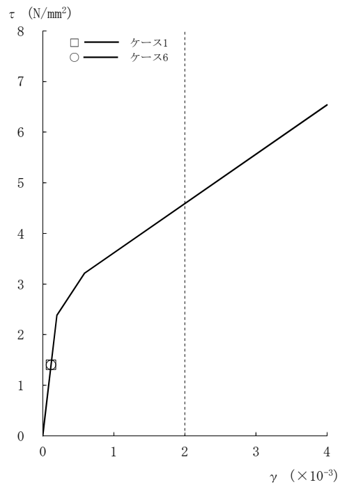
図2-102 \tau - \gamma 関係と最大応答値 (Ss-3, NS方向, 4F) (2/8)
