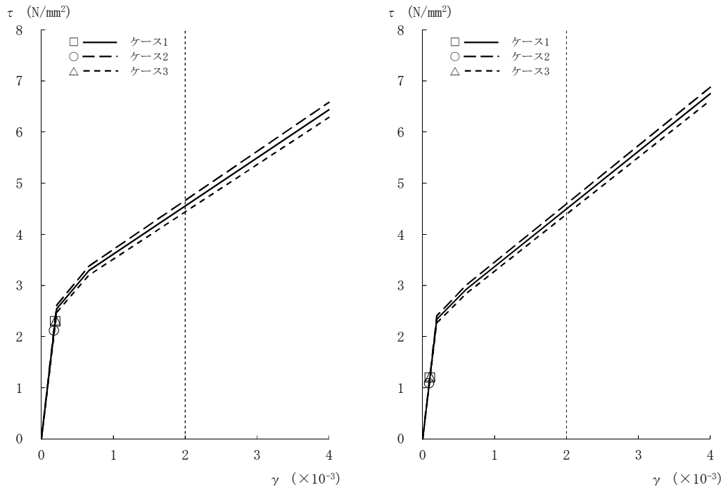
図2-19 \tau - \gamma 関係と最大応答値 (Ss-2, NS方向, 1F) (5/8)
