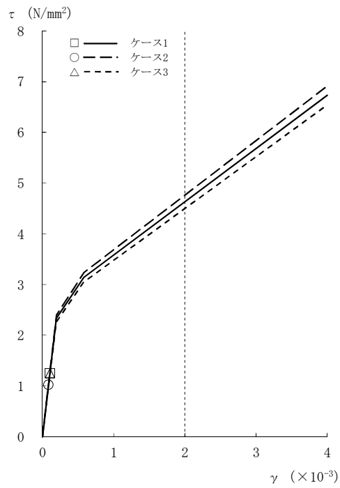
図2-23 τ - γ 関係と最大応答値 (Ss-2, EW方向, 4F) (2/8)
