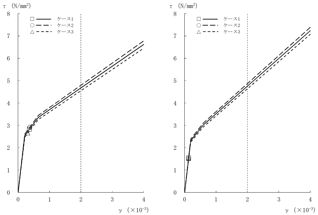
図2-18 τ - γ 関係と最大応答値 (Ss-1, NS方向, 2F) (4/8)
