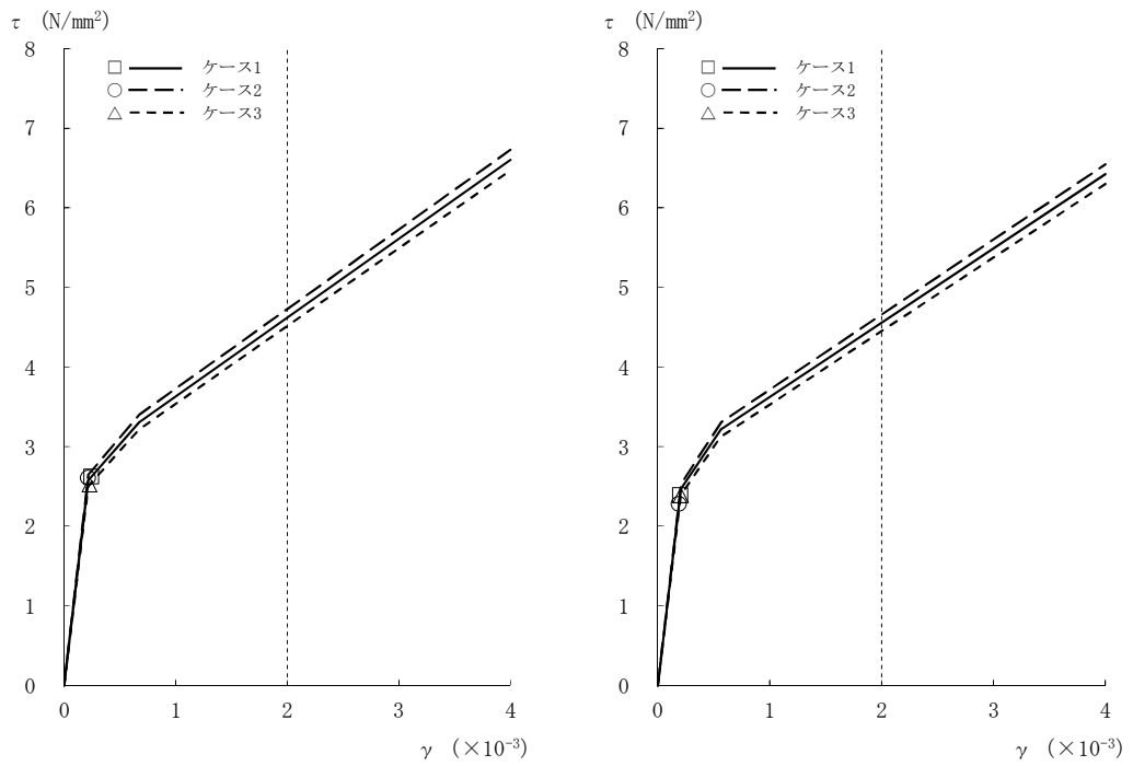
図2-22 τ - γ 関係と最大応答値 (S s -1, EW方向, B3F) (8/8)
