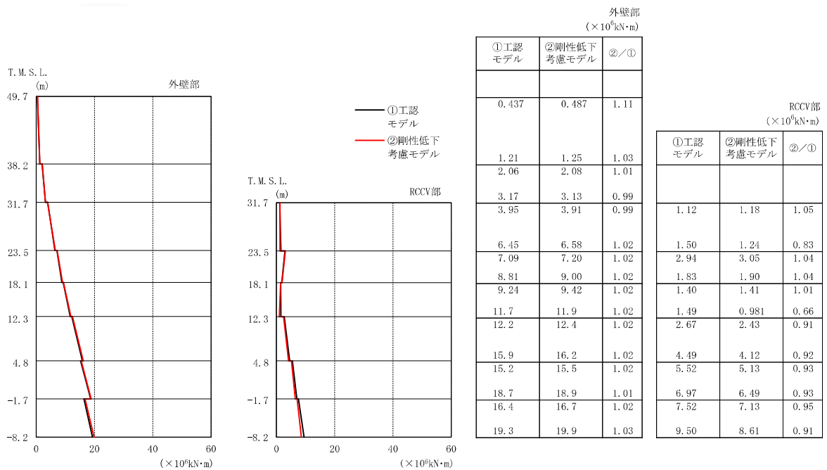
図 3-11 最大応答曲げモーメント (Ss-1, EW 方向)
