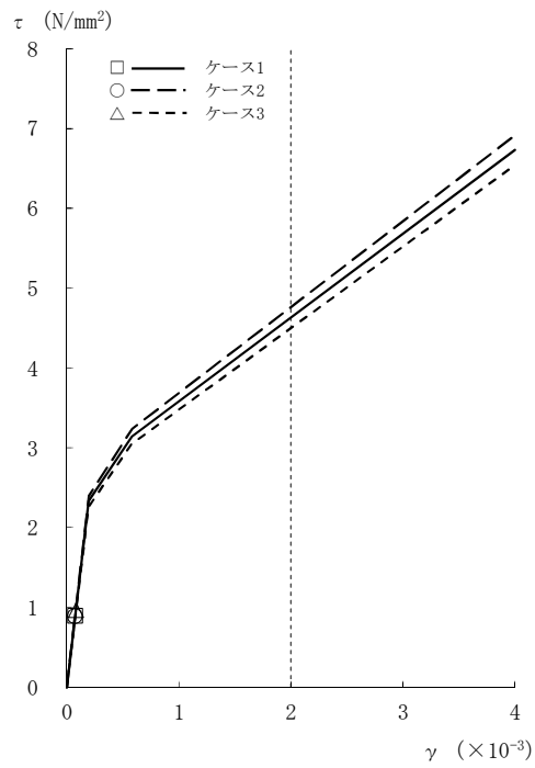
図2-24 \tau - \gamma 関係と最大応答値 (Ss-3, EW方向, 4F) (2/8)
