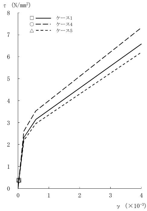
図2-84 τ - γ 関係と最大応答値 (Sd-3, EW方向, CRF) (1/8)
