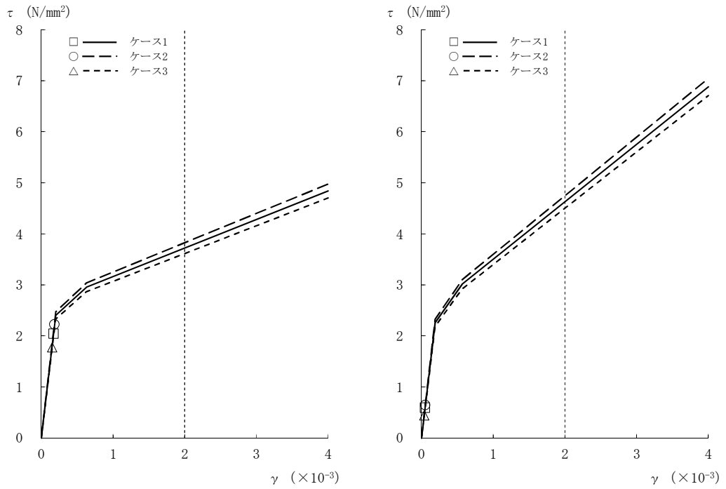
図2-18 τ - γ 関係と最大応答値 (Ss-1, NS方向, 3F) (3/8)
