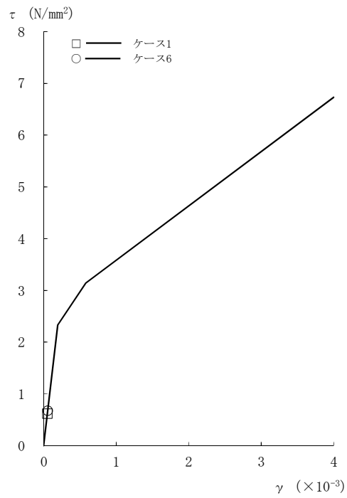
図2-121 τ - γ 関係と最大応答値 (Sd-2, EW方向, 4F) (2/8)
