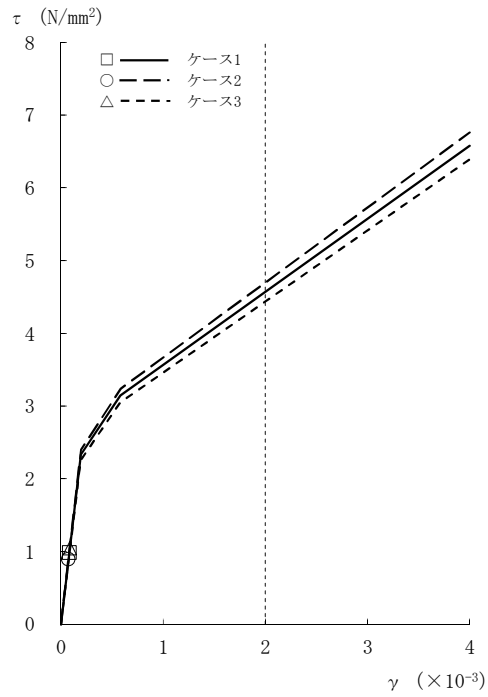
図2-25 τ - γ 関係と最大応答値 (S s -8, EW方向, CRF) (1/8)
