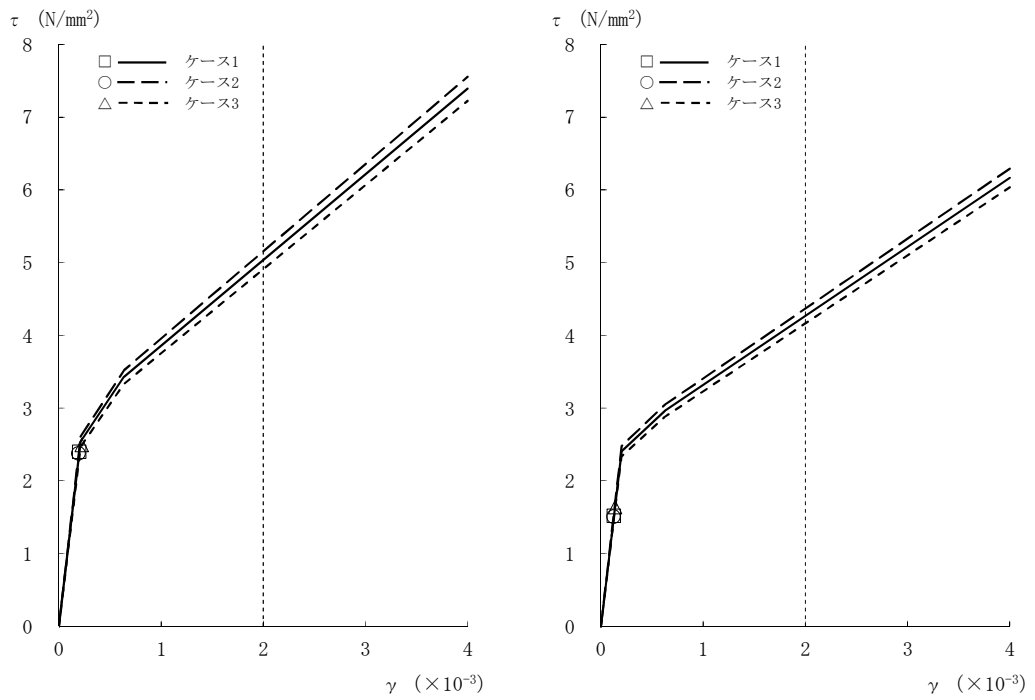
図2-24 τ - γ 関係と最大応答値 (Ss-3, EW方向, B1F) (6/8)
