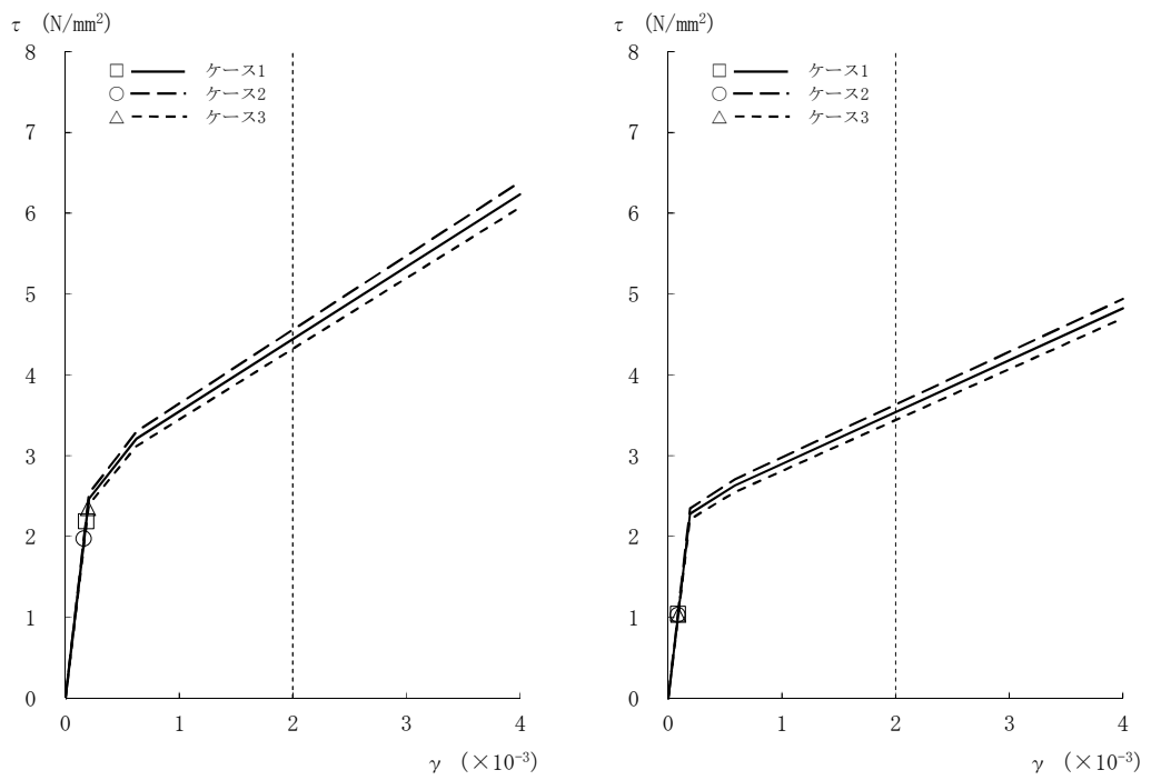
図2-25 \tau - \gamma 関係と最大応答値 (Ss-8, EW方向, 2F) (4/8)
