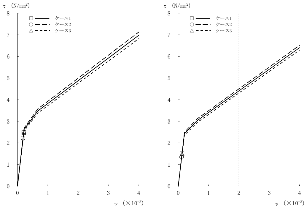
図2-19 \tau - \gamma 関係と最大応答値 (Ss-2, NS方向, B1F) (6/8)
