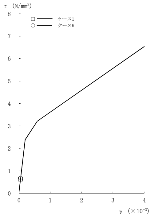
図2-117 τ - γ 関係と最大応答値 (Sd-2, NS方向, 4F) (2/8)
