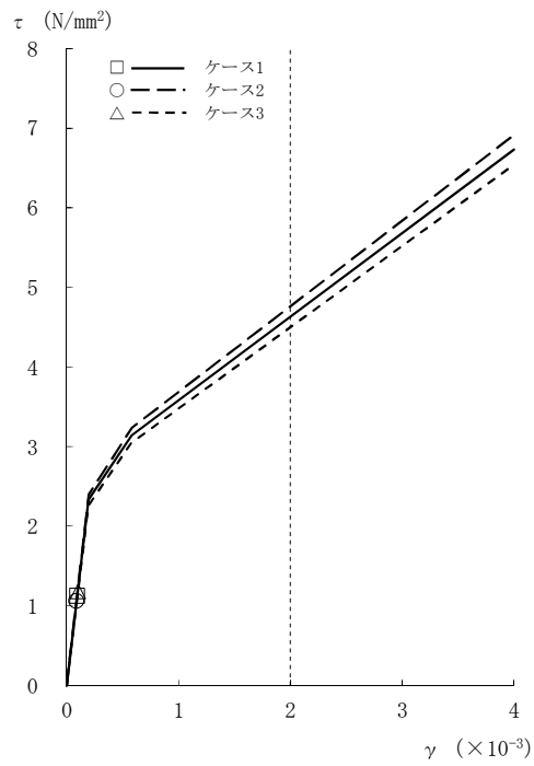
図2-25 τ - γ 関係と最大応答値 (S s -8, EW方向, 4F) (2/8)
