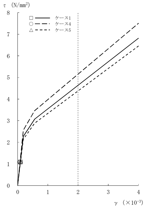
図2-60 τ - γ 関係と最大応答値 (S s -2, NS方向, CRF) (1/8)
