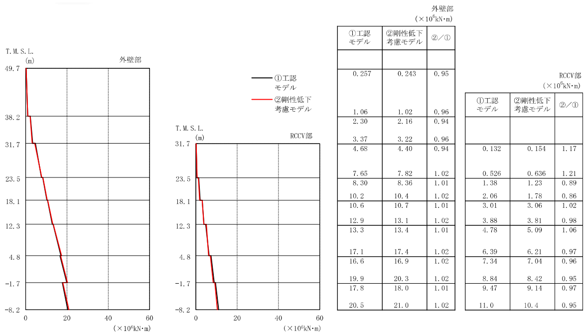
図 3-7 最大応答曲げモーメント (Ss-1, NS 方向)
