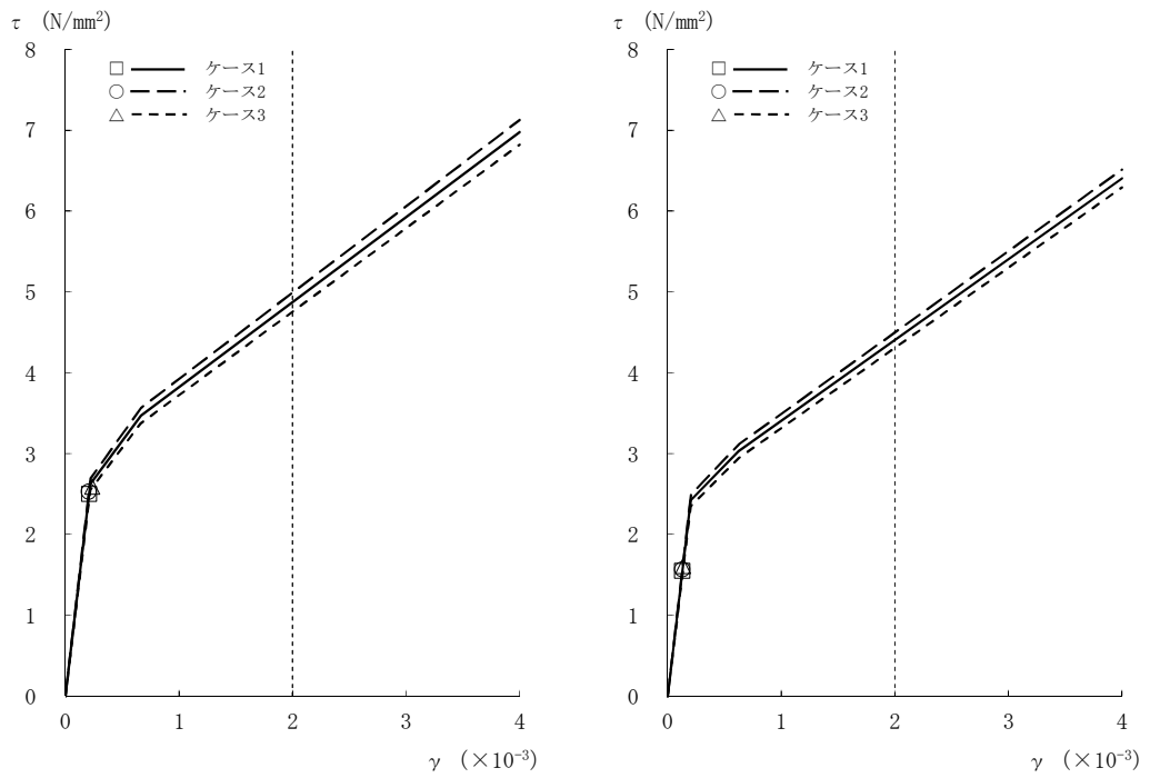
図2-20 τ - γ 関係と最大応答値 (Ss-3, NS方向, B1F) (6/8)
