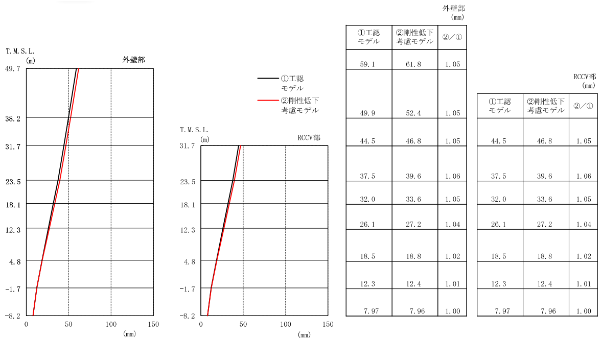
図 3-5 最大応答変位 (Ss-1, NS 方向)
