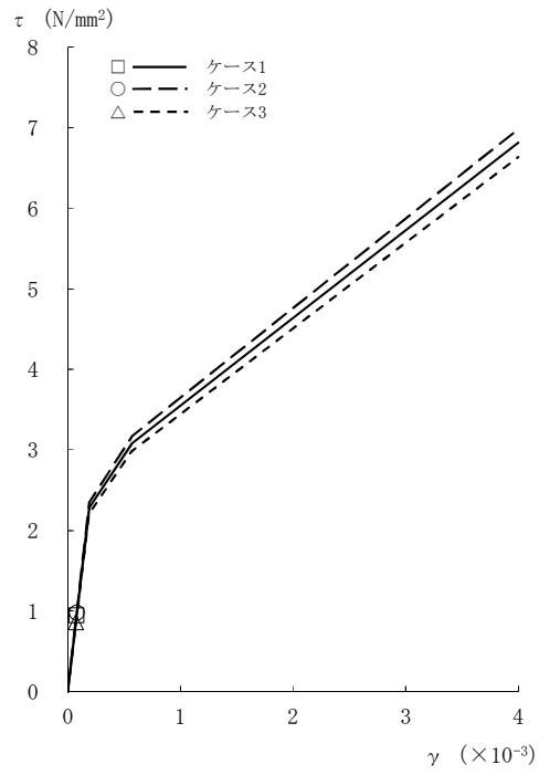
図2-37 \tau - \gamma 関係と最大応答値 (Sd-1, NS方向, CRF) (1/8)
