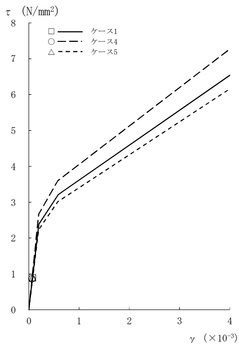
図2-81 τ - γ 関係と最大応答値 (Sd-8, NS方向, 4F) (2/8)
