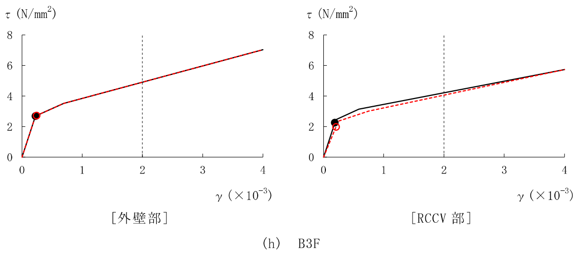
図 3-15 せん断スケルトン曲線上の最大応答値 (Ss-1, NS 方向) (3/3)
