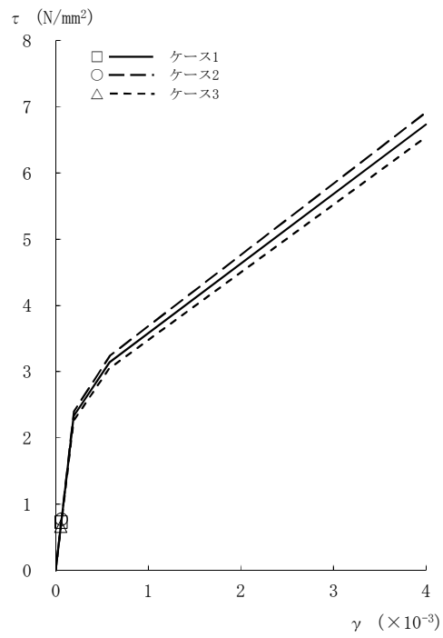
図2-41 τ - γ 関係と最大応答値 (Sd-1, EW方向, 4F) (2/8)
