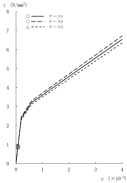
図2-40 τ - γ 関係と最大応答値 (Sd-8, NS方向, 4F) (2/8)
