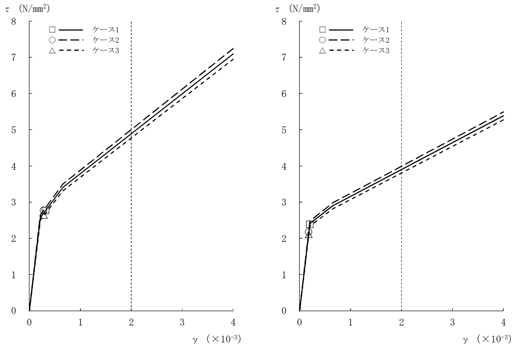
図2-22 τ - γ 関係と最大応答値 (S s -1, EW方向, B2F) (7/8)
