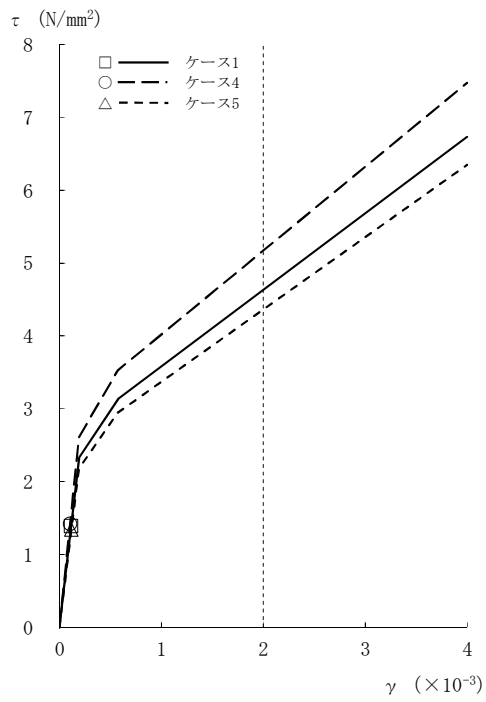
図2-63 τ - γ 関係と最大応答値 (Ss-1, EW方向, 4F) (2/8)
