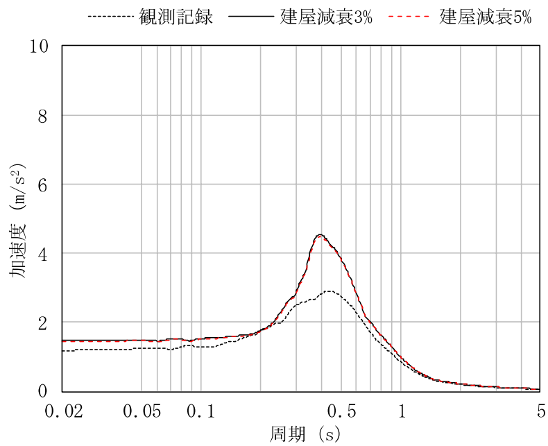
(b) EW 方向 4F (T. M. S. L. 31.7m, h = 5%)
