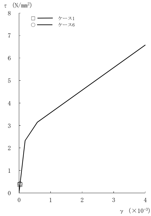
図2-122 τ - γ 関係と最大応答値 (Sd-3, EW方向, CRF) (1/8)
