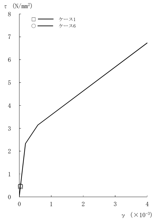
図2-122 τ - γ 関係と最大応答値 (Sd-3, EW方向, 4F) (2/8)
