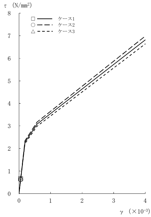
図2-40 τ - γ 関係と最大応答値 (Sd-8, NS方向, CRF) (1/8)
