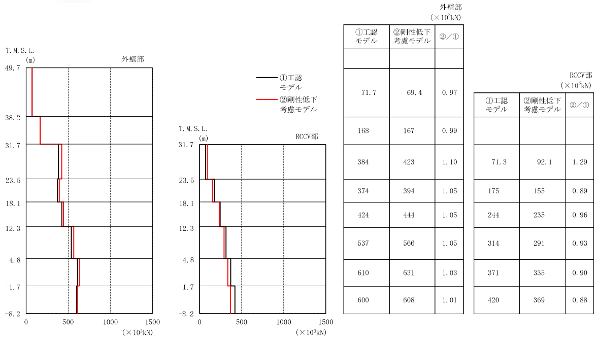
図 3-6 最大応答せん断力 (Ss-1, NS 方向)
