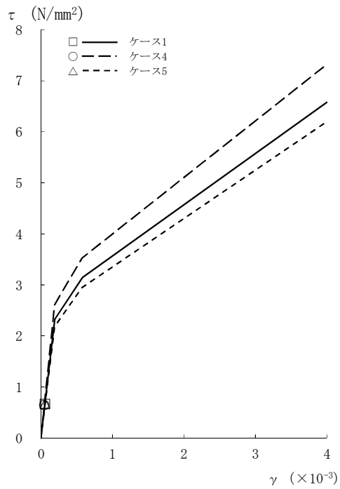
図2-82 \tau - \gamma 関係と最大応答値 (Sd-1, EW方向, CRF) (1/8)
