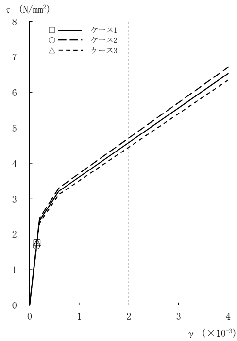
図2-21 \tau - \gamma 関係と最大応答値 (Ss-8, NS方向, 4F) (2/8)
