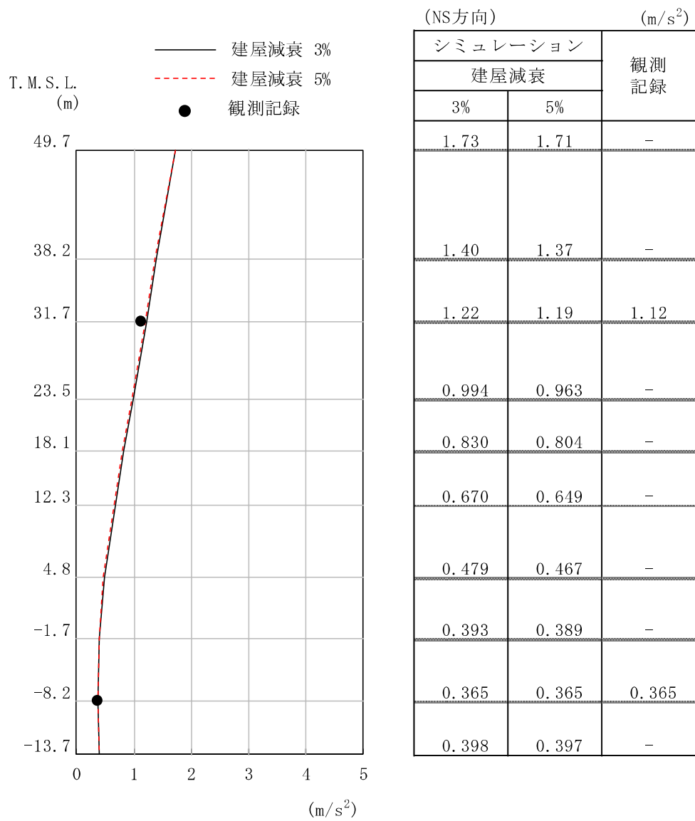
図 2-1 最大応答加速度分布の比較 (NS 方向) : 中越地震 (余震) 観測記録 (1/3)
