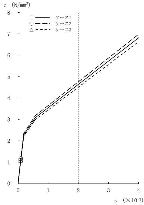
図2-19 \tau - \gamma 関係と最大応答値 (Ss-2, NS方向, CRF) (1/8)
