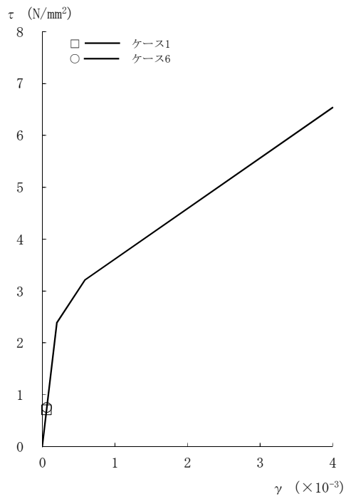
図2-118 τ - γ 関係と最大応答値 (Sd-3, NS方向, 4F) (2/8)
