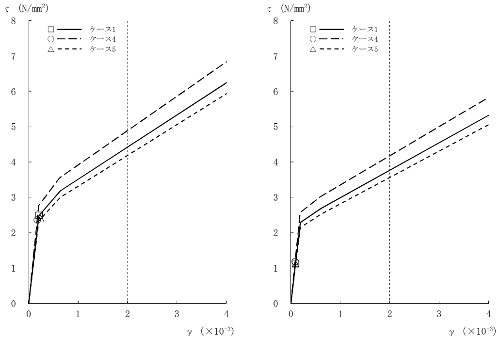
図2-66 τ - γ 関係と最大応答値 (Ss-8, EW方向, 1F) (5/8)
