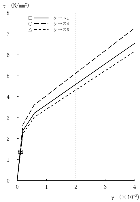
図2-60 τ - γ 関係と最大応答値 (S s -2, NS方向, 4F) (2/8)
