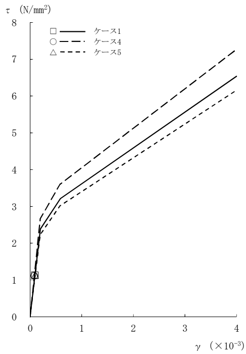
図2-78 τ - γ 関係と最大応答値 (Sd-1, NS方向, 4F) (2/8)
