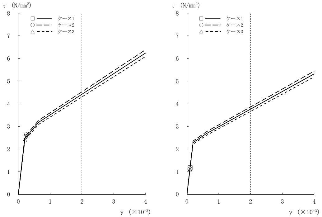
図2-22 τ - γ 関係と最大応答値 (Ss-1, EW方向, 1F) (5/8)
