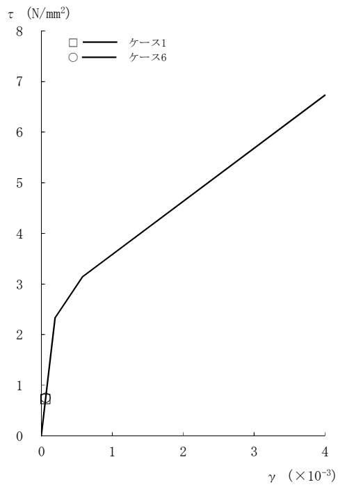
図2-120 τ - γ 関係と最大応答値 (Sd-1, EW方向, 4F) (2/8)
