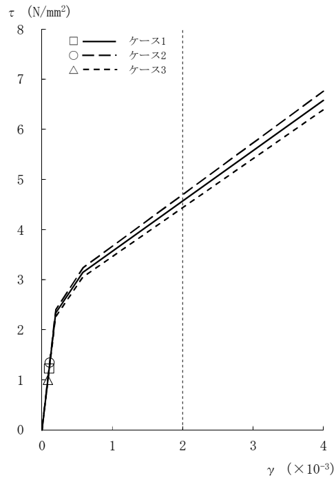
図2-22 τ - γ 関係と最大応答値 (Ss-1, EW方向, CRF) (1/8)
