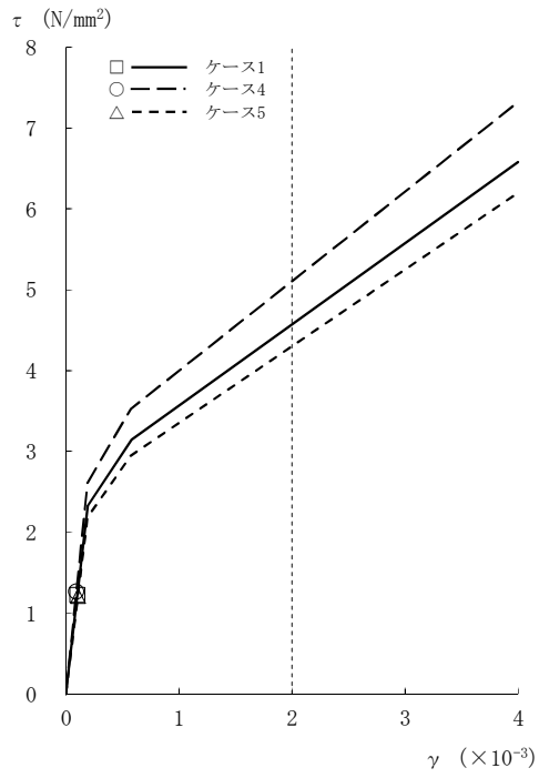
図2-63 τ - γ 関係と最大応答値 (Ss-1, EW方向, CRF) (1/8)
