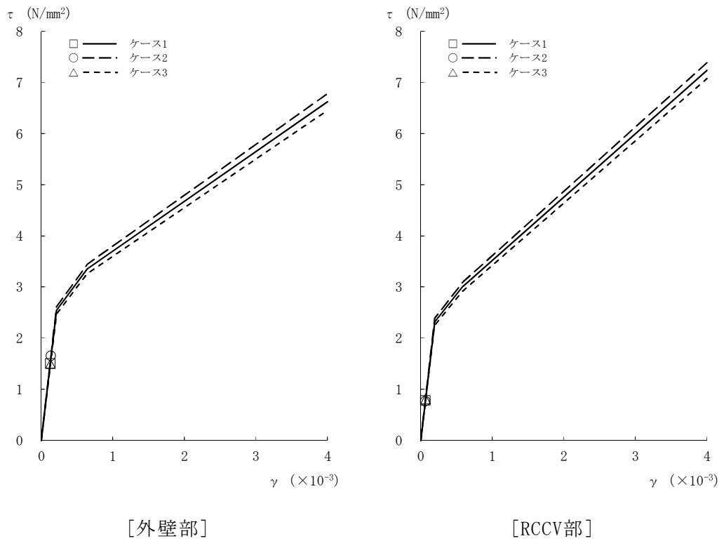
図2-37 \tau - \gamma 関係と最大応答値 (Sd-1, NS方向, 2F) (4/8)
