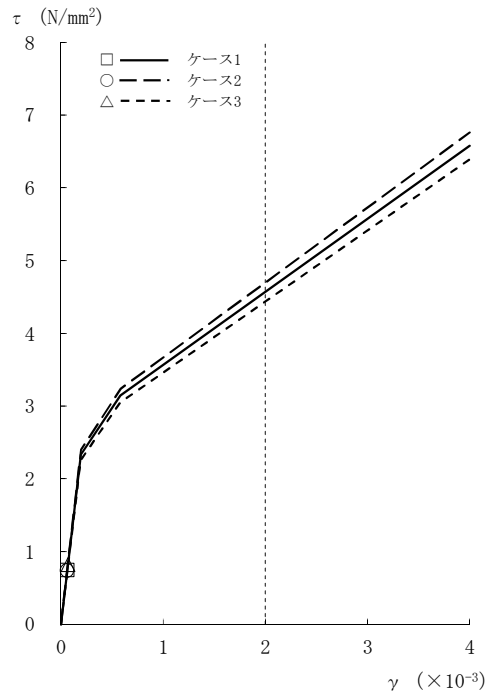
図2-24 \tau - \gamma 関係と最大応答値 (Ss-3, EW方向, CRF) (1/8)
