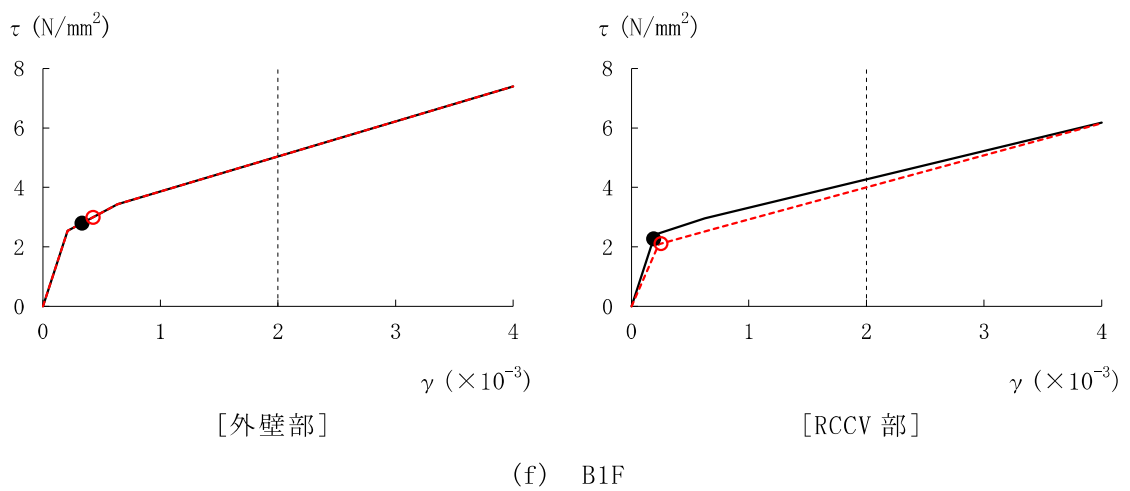
図 3-16 せん断スケルトン曲線上の最大応答値 (Ss-1, EW 方向) (2/3)
