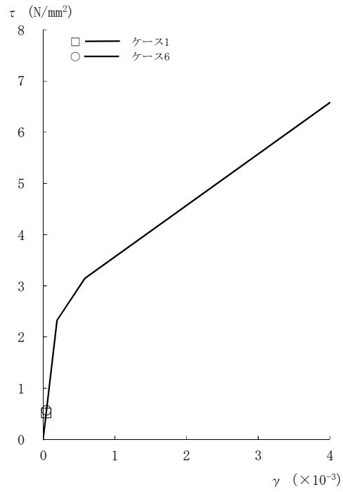
図2-121 τ - γ 関係と最大応答値 (Sd-2, EW方向, CRF) (1/8)
