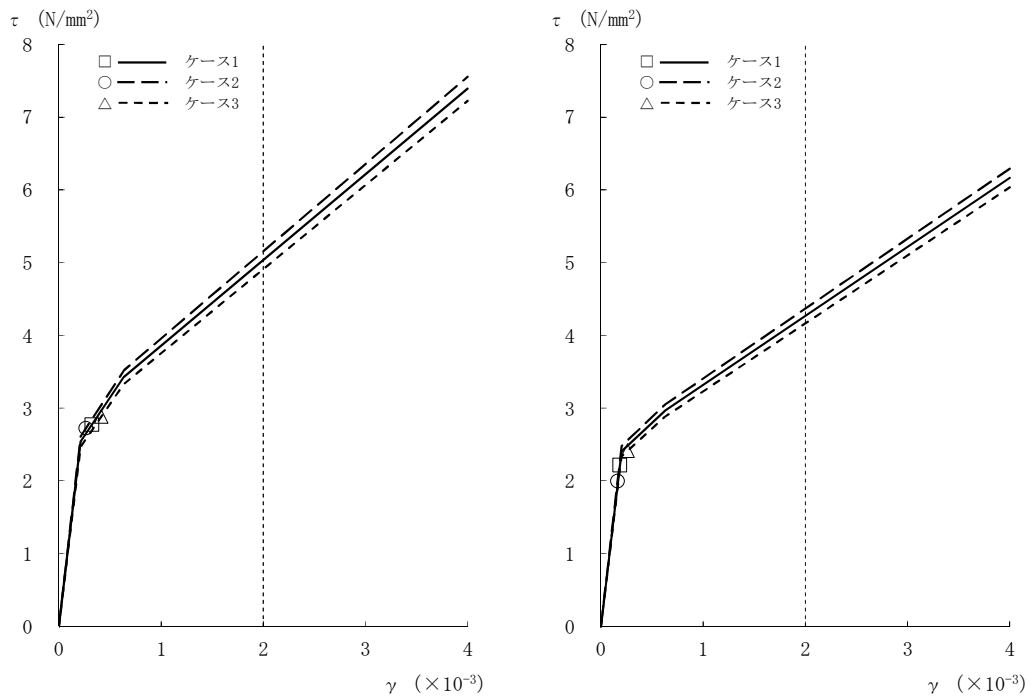
図2-25 τ - γ 関係と最大応答値 (Ss-8, EW方向, B1F) (6/8)
