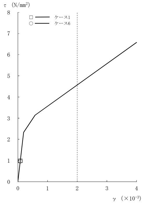
図2-107 τ - γ 関係と最大応答値 (Ss-8, EW方向, CRF) (1/8)
