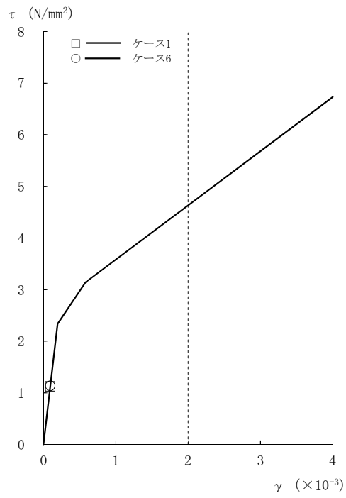
図2-107 τ - γ 関係と最大応答値 (Ss-8, EW方向, 4F) (2/8)
