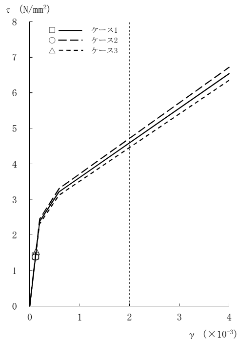
図2-20 \tau - \gamma 関係と最大応答値 (Ss-3, NS方向, 4F) (2/8)
