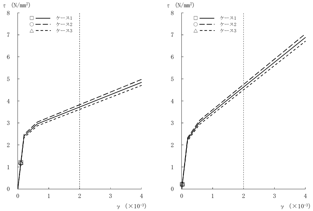
図2-19 τ - γ 関係と最大応答値 (Ss-2, NS方向, 3F) (3/8)
