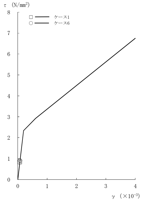
図2-116 τ - γ 関係と最大応答値 (Sd-1, NS方向, 1F) (5/8)
