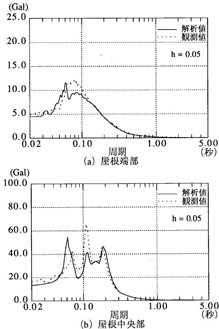
図3-7 中部電力（株）浜岡原子力発電所3号機原子炉建屋のシミュレーション解析結果 3.7)
