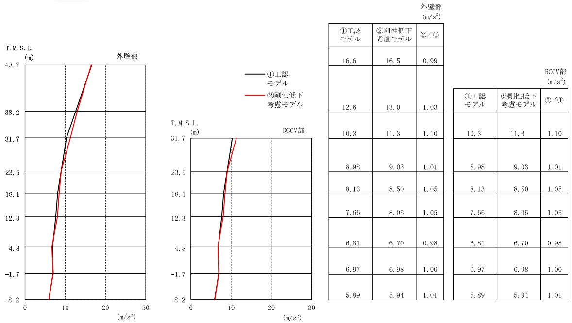
図 3-8 最大応答加速度 (Ss-1, EW 方向)
