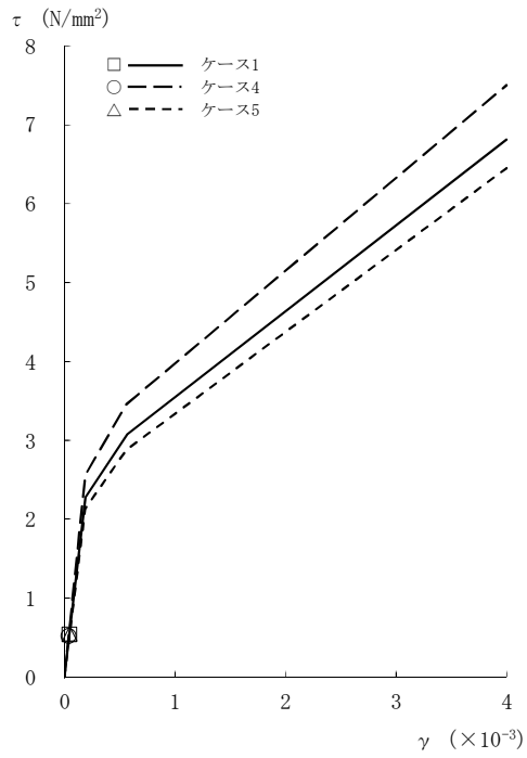
図2-80 τ - γ 関係と最大応答値 (Sd-3, NS方向, CRF) (1/8)
