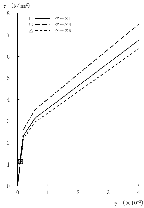
図2-66 τ - γ 関係と最大応答値 (Ss-8, EW方向, 4F) (2/8)
