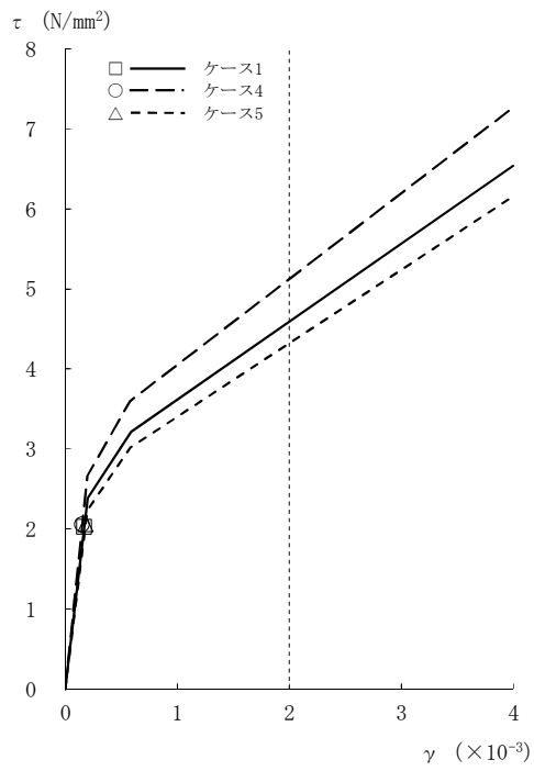
図2-59 \tau - \gamma 関係と最大応答値 (S s -1, NS方向, 4F) (2/8)
