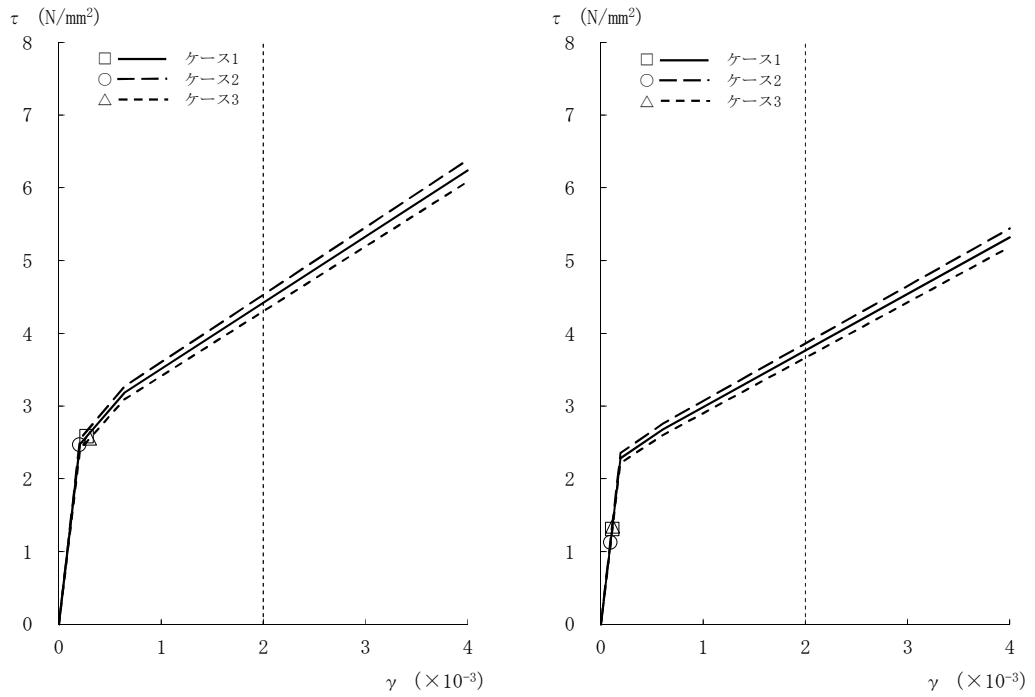
図2-23 τ - γ 関係と最大応答値 (Ss-2, EW方向, 1F) (5/8)
