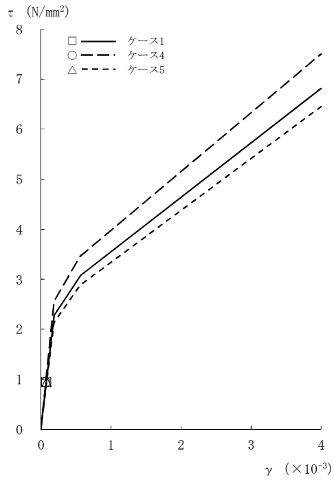
図2-78 τ - γ 関係と最大応答値 (Sd-1, NS方向, CRF) (1/8)
