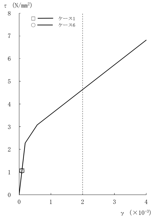
図2-102 \tau - \gamma 関係と最大応答値 (Ss-3, NS方向, CRF) (1/8)
