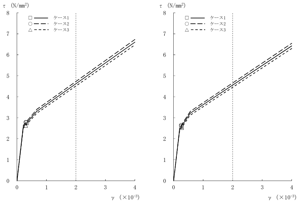
図2-23 \tau - \gamma 関係と最大応答値 (S s -2, EW方向, B3F) (8/8)
