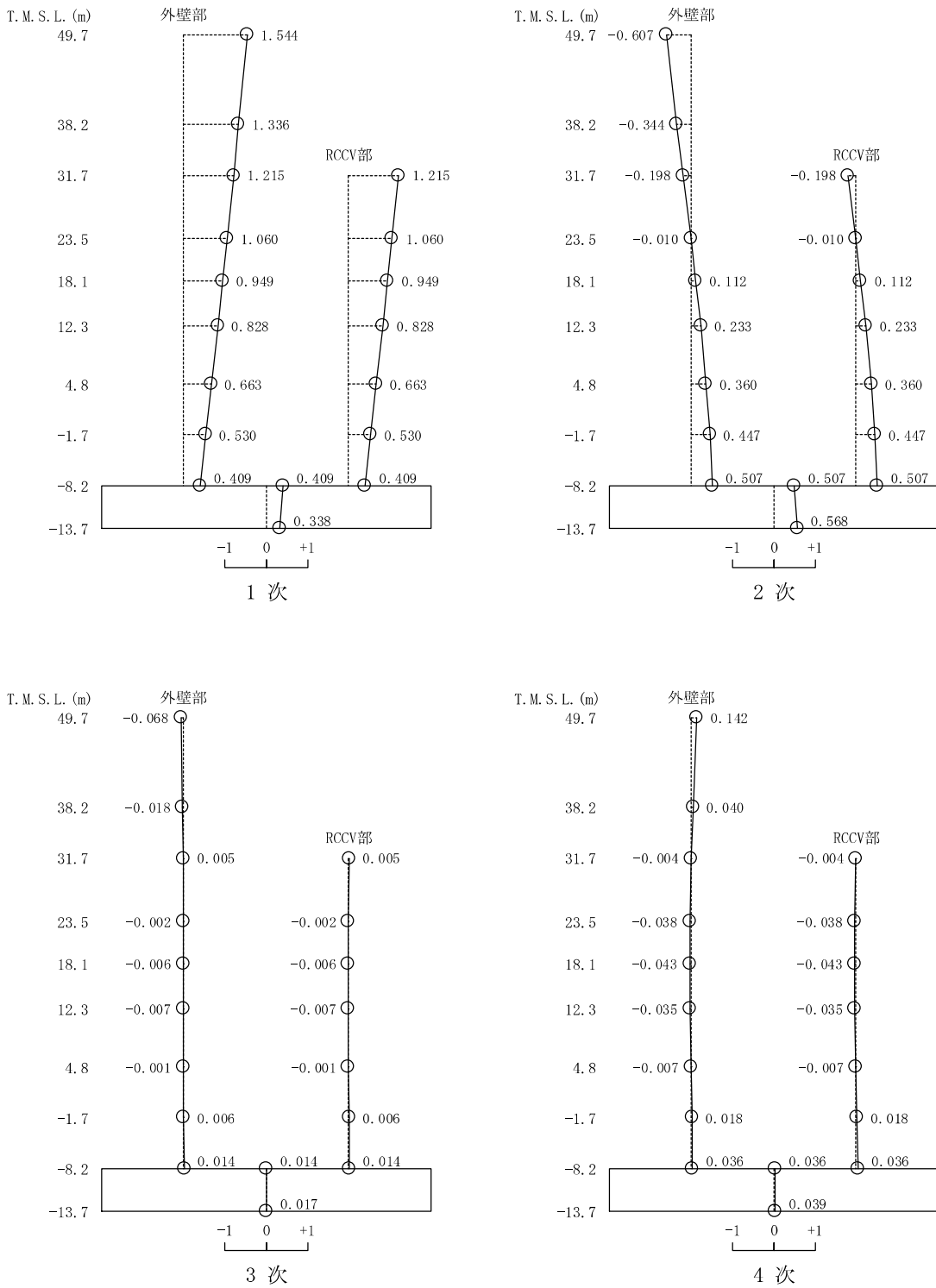
図 3-3 刺激関数図 (Ss-1, EW 方向, 剛性低下考慮モデル) (2/3)
