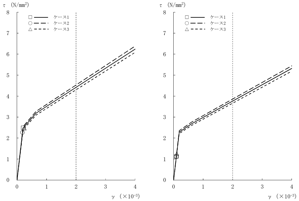
図2-25 τ - γ 関係と最大応答値 (Ss-8, EW方向, 1F) (5/8)
