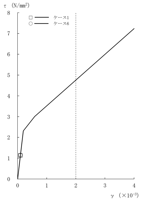
図2-102 \tau - \gamma 関係と最大応答値 (Ss-3, NS方向, 2F) (4/8)
