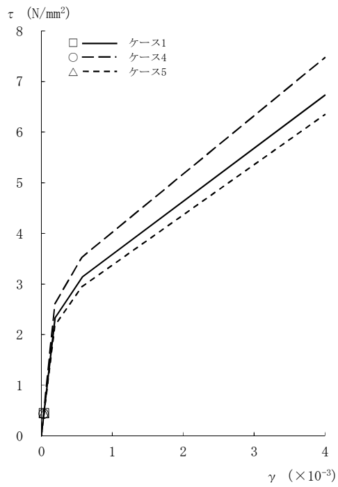
図2-84 τ - γ 関係と最大応答値 (Sd-3, EW方向, 4F) (2/8)
