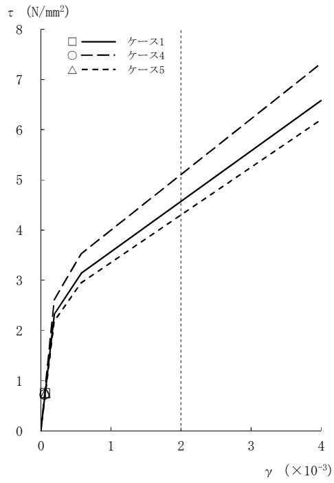
図2-65 τ - γ 関係と最大応答値 (Ss-3, EW方向, CRF) (1/8)
