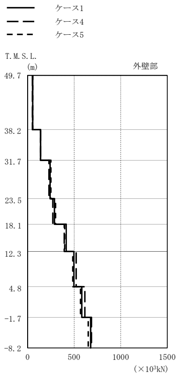
図2-51 最大応答せん断力(基準地震動 S s , EW方向)(2/2)
