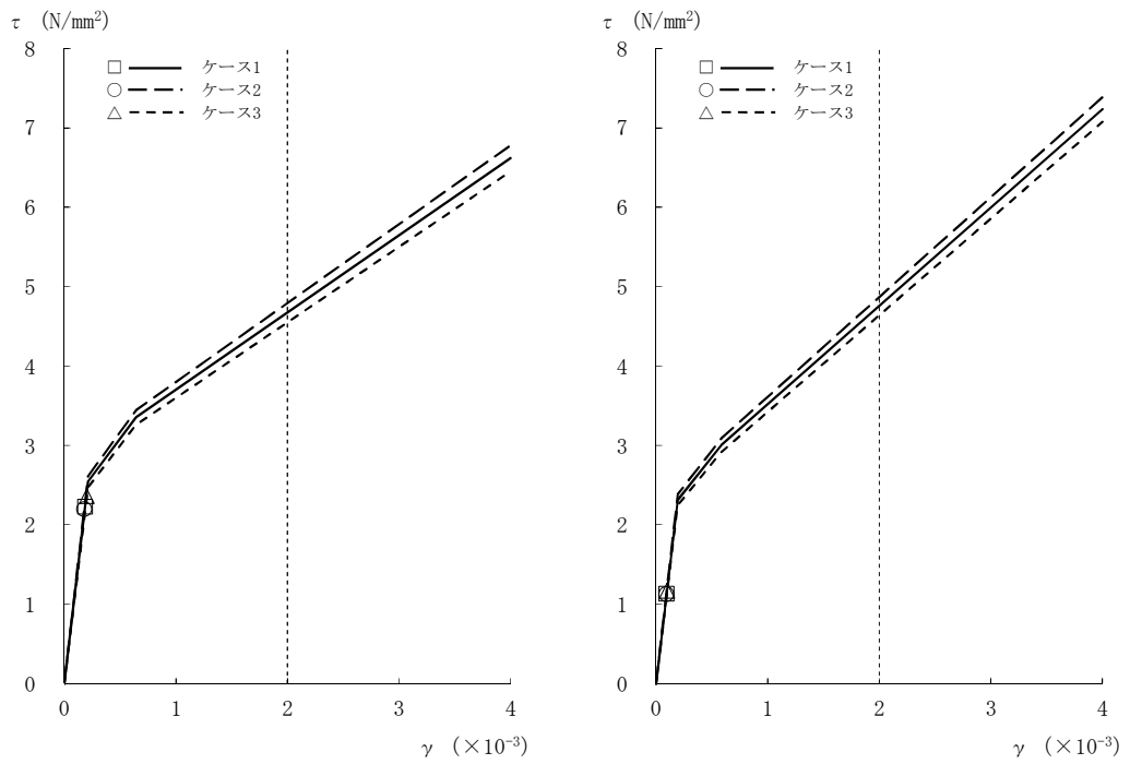
図2-20 τ - γ 関係と最大応答値 (Ss-3, NS方向, 2F) (4/8)
