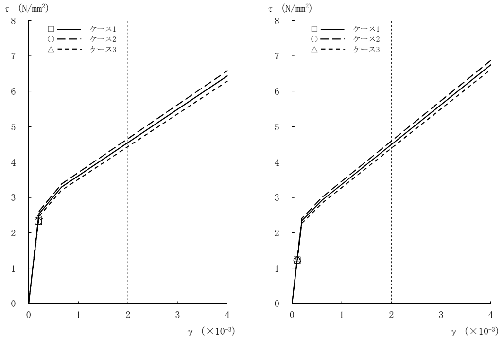
図2-20 τ - γ 関係と最大応答値 (Ss-3, NS方向, 1F) (5/8)
