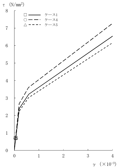
図2-80 τ - γ 関係と最大応答値 (Sd-3, NS方向, 4F) (2/8)
