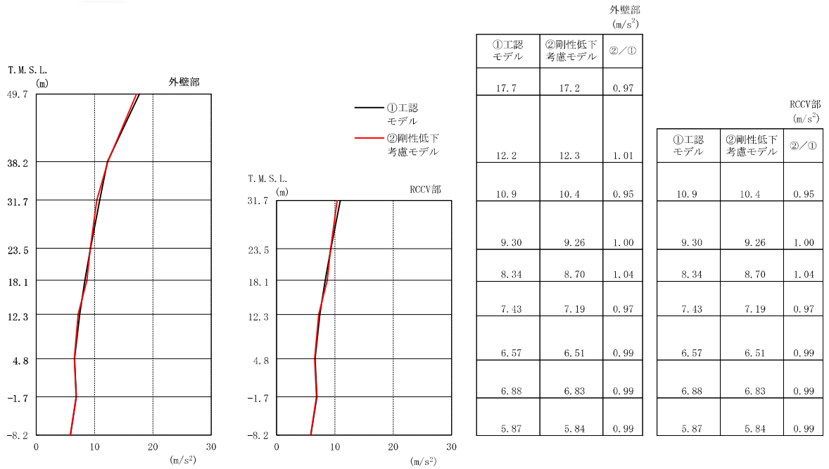
図 3-4 最大応答加速度 (Ss-1, NS 方向)
