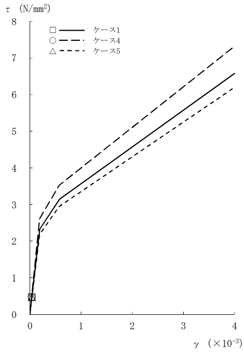
図2-85 τ - γ 関係と最大応答値 (Sd-8, EW方向, CRF) (1/8)
