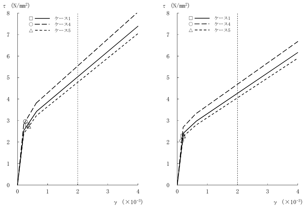
図2-63 \tau - \gamma 関係と最大応答値 (Ss-1, EW方向, B1F) (6/8)
