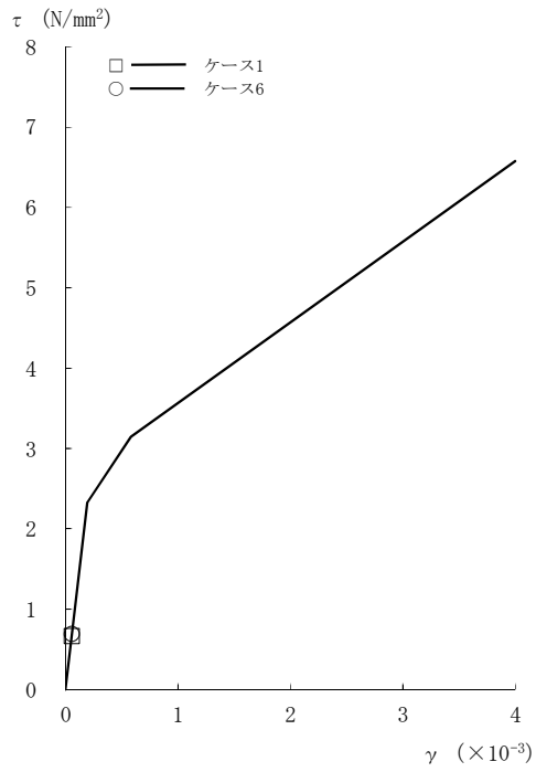
図2-120 τ - γ 関係と最大応答値 (Sd-1, EW方向, CRF) (1/8)
