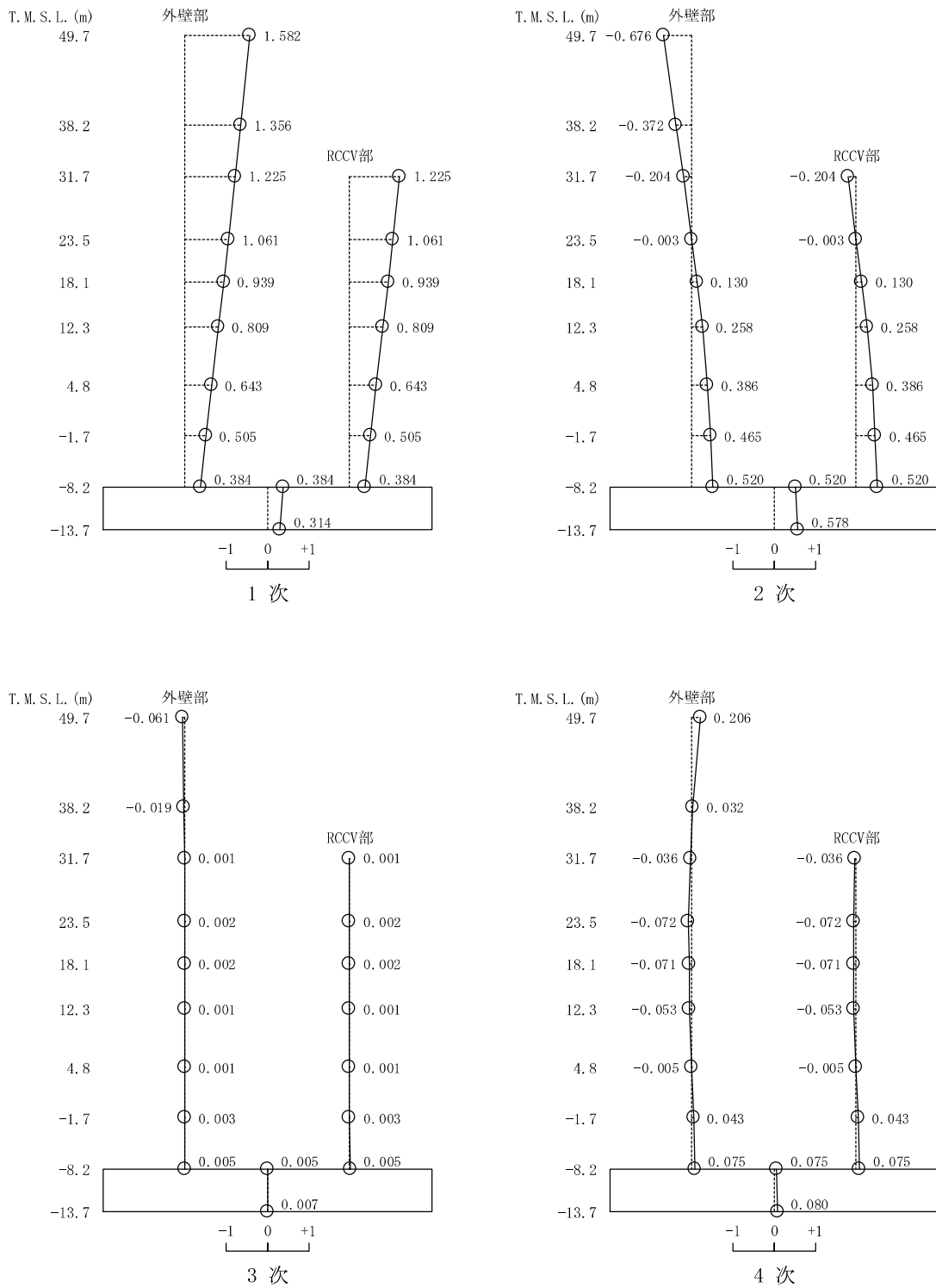
図 3-3 刺激関数図 (Ss-1, NS 方向, 剛性低下考慮モデル) (1/3)
