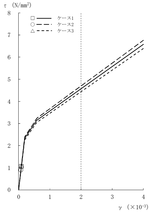
図2-23 τ - γ 関係と最大応答値 (Ss-2, EW方向, CRF) (1/8)
