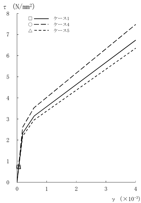
図2-82 \tau - \gamma 関係と最大応答値 (Sd-1, EW方向, 4F) (2/8)
