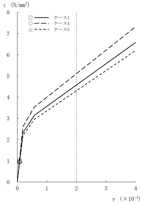
図2-66 τ - γ 関係と最大応答値 (Ss-8, EW方向, CRF) (1/8)
