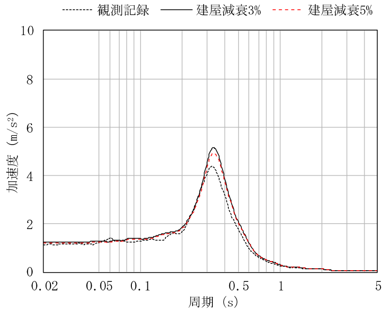
(a) NS 方向 4F (T. M. S. L. 31.7m, h = 5%)
