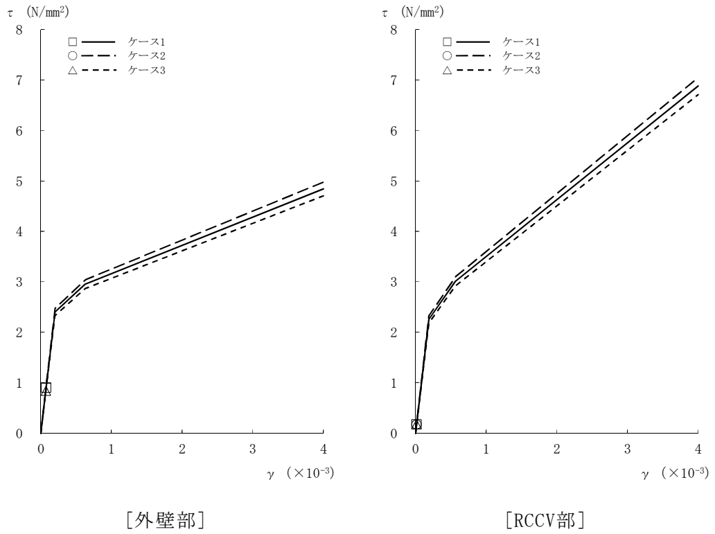
図2-37 \tau - \gamma 関係と最大応答値 (Sd-1, NS方向, 3F) (3/8)
