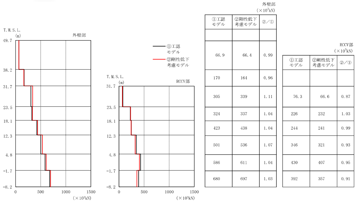
図 3-10 最大応答せん断力 (Ss-1, EW 方向)
