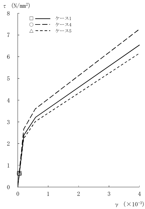
図2-79 τ - γ 関係と最大応答値 (Sd-2, NS方向, 4F) (2/8)
