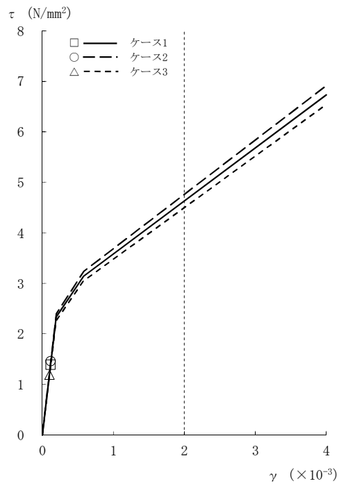
図2-22 τ - γ 関係と最大応答値 (Ss-1, EW方向, 4F) (2/8)
