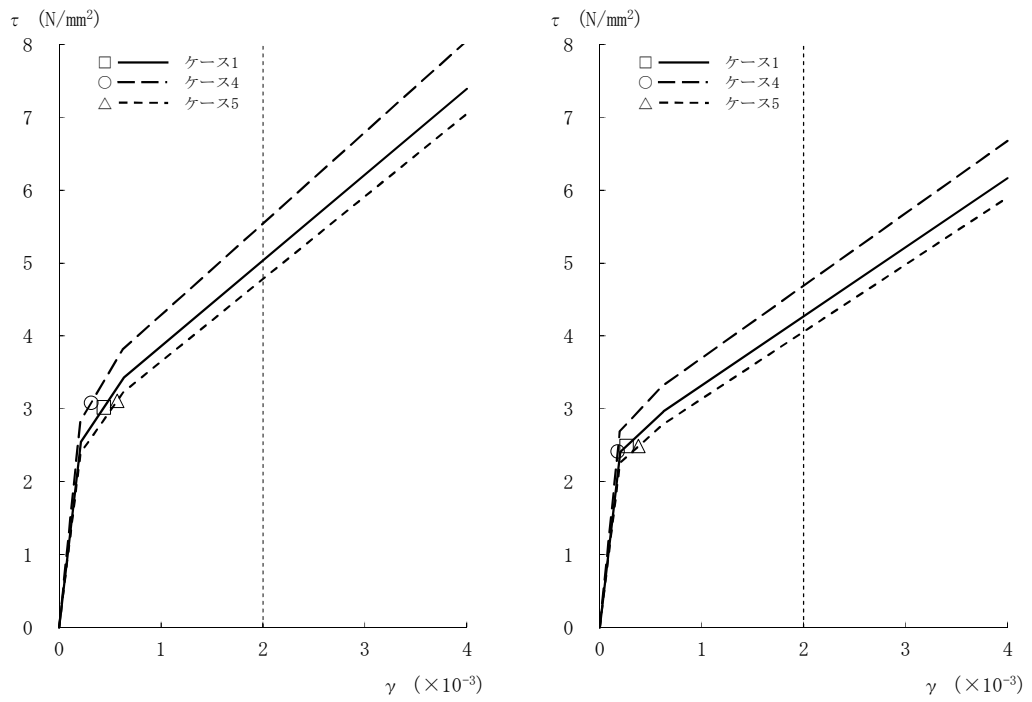
図2-64 τ - γ 関係と最大応答値 (Ss-2, EW方向, B1F) (6/8)
