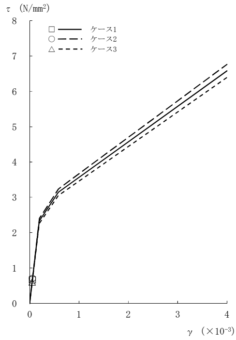
図2-41 τ - γ 関係と最大応答値 (Sd-1, EW方向, CRF) (1/8)
