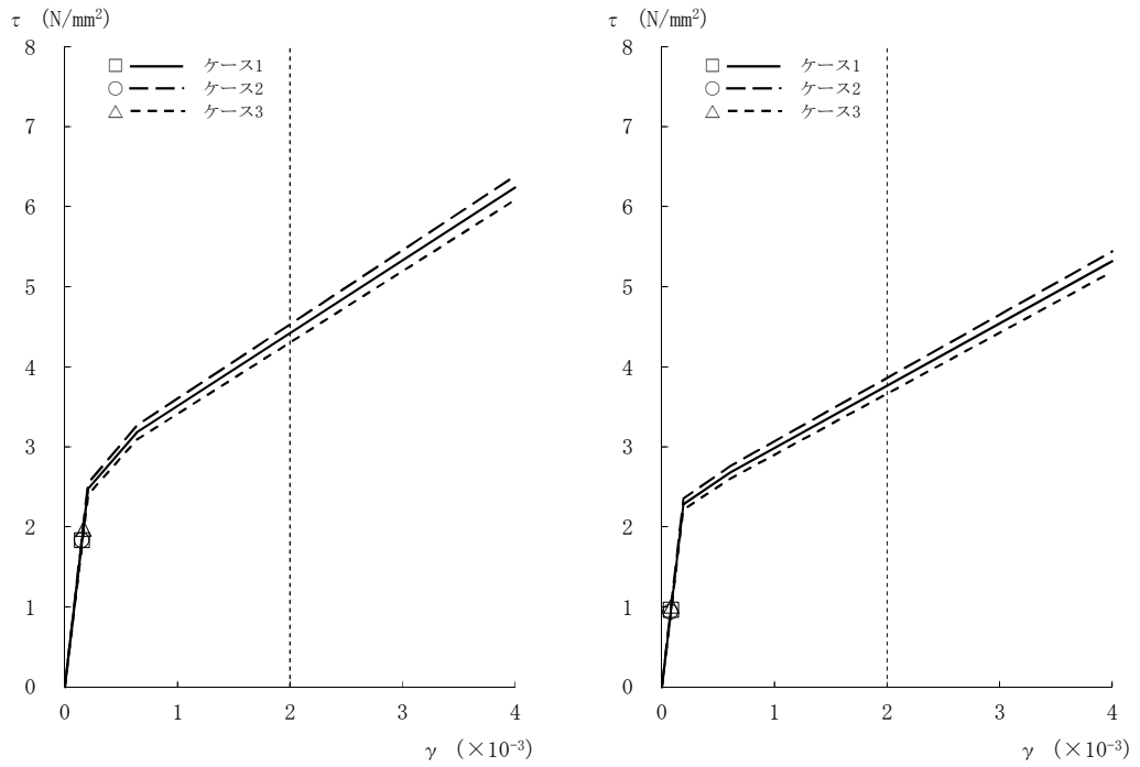
図2-24 τ - γ 関係と最大応答値 (Ss-3, EW方向, 1F) (5/8)
