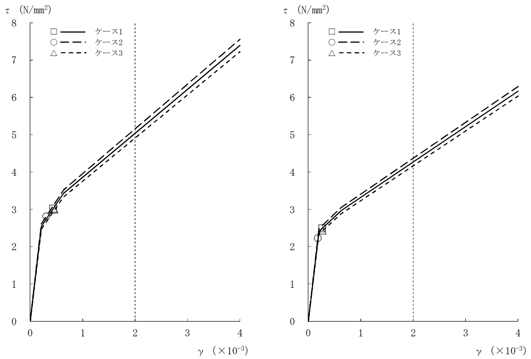
図2-23 τ - γ 関係と最大応答値 (Ss-2, EW方向, B1F) (6/8)
