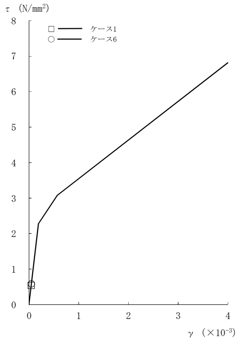
図2-118 τ - γ 関係と最大応答値 (Sd-3, NS方向, CRF) (1/8)
