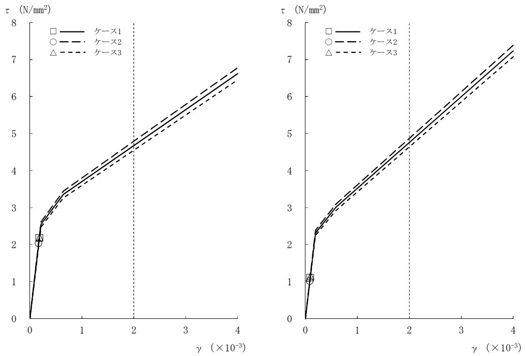
図2-19 τ - γ 関係と最大応答値 (Ss-2, NS方向, 2F) (4/8)
