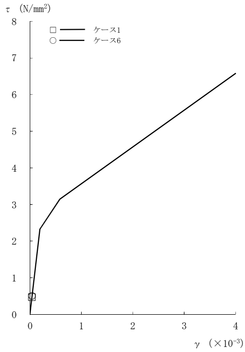
図2-123 τ - γ 関係と最大応答値 (Sd-8, EW方向, CRF) (1/8)
