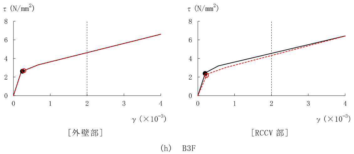
図 3-16 せん断スケルトン曲線上の最大応答値 (Ss-1, EW 方向) (3/3)
