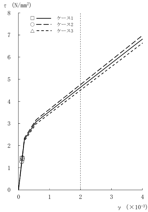
図2-21 \tau - \gamma 関係と最大応答値 (Ss-8, NS方向, CRF) (1/8)
