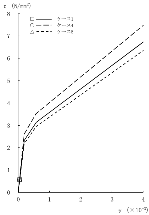
図2-85 τ - γ 関係と最大応答値 (Sd-8, EW方向, 4F) (2/8)
