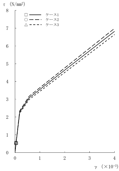
図2-39 τ - γ 関係と最大応答値 (Sd-3, NS方向, CRF) (1/8)
