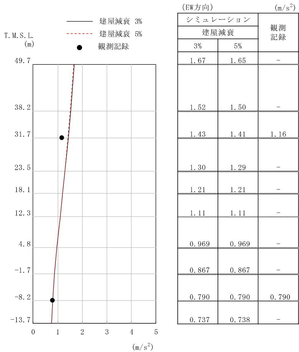
図 2-1 最大応答加速度分布の比較 (EW 方向) : 中越地震 (余震) 観測記録 (2/3)
