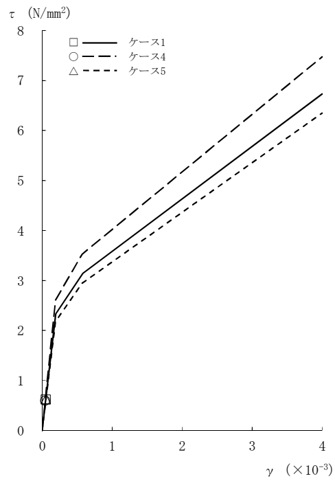
図2-83 τ - γ 関係と最大応答値 (Sd-2, EW方向, 4F) (2/8)
