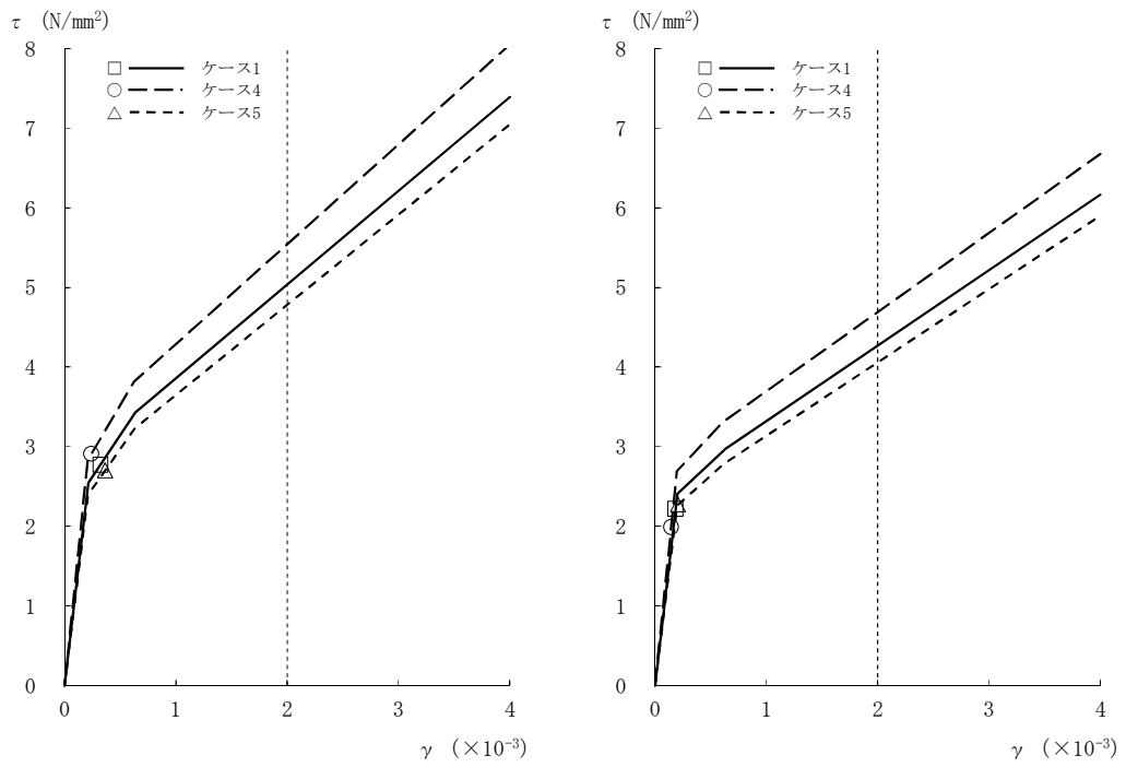
図2-66 τ - γ 関係と最大応答値 (Ss-8, EW方向, B1F) (6/8)
