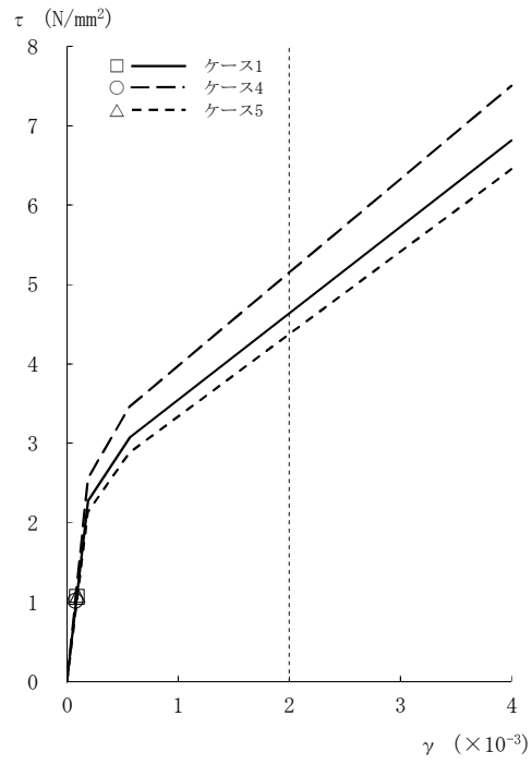
図2-61 τ - γ 関係と最大応答値 (Ss-3, NS方向, CRF) (1/8)
