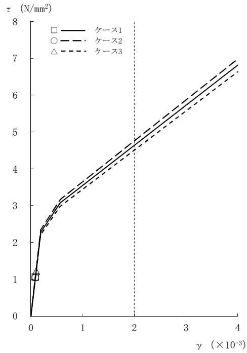
図2-20 \tau - \gamma 関係と最大応答値 (Ss-3, NS方向, CRF) (1/8)
