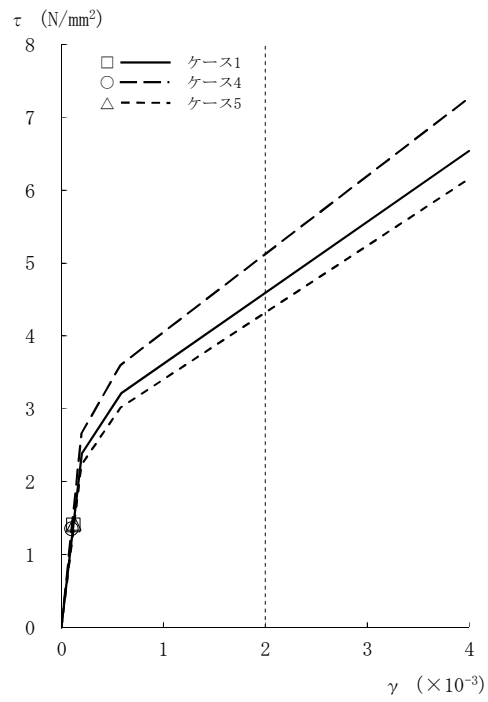
図2-61 τ - γ 関係と最大応答値 (Ss-3, NS方向, 4F) (2/8)
