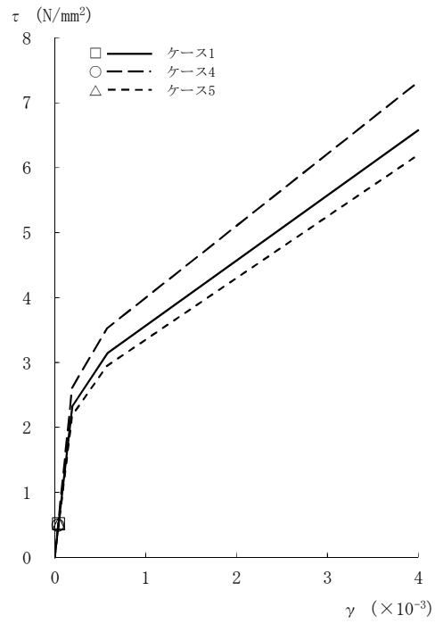
図2-83 τ - γ 関係と最大応答値 (Sd-2, EW方向, CRF) (1/8)
