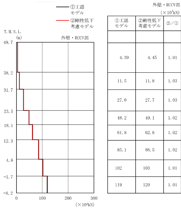
図 3-14 最大応答軸力 (Ss-1, 鉛直方向)
