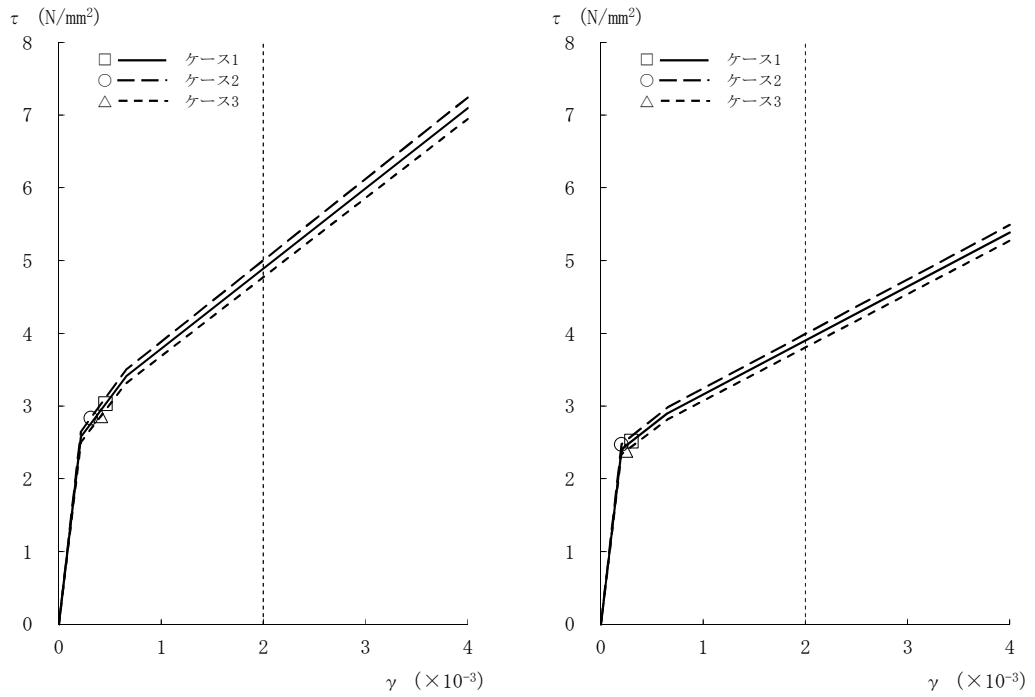
図2-23 \tau - \gamma 関係と最大応答値 (S s -2, EW方向, B2F) (7/8)
