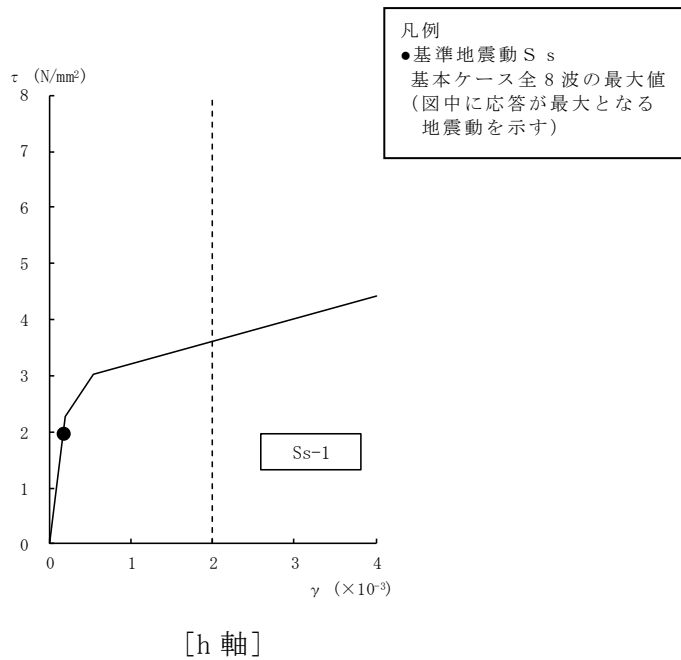
図 4-15 せん断スケルトン曲線上の最大応答値 (基準地震動 S s , EW 方向, 1F) (1/4)
