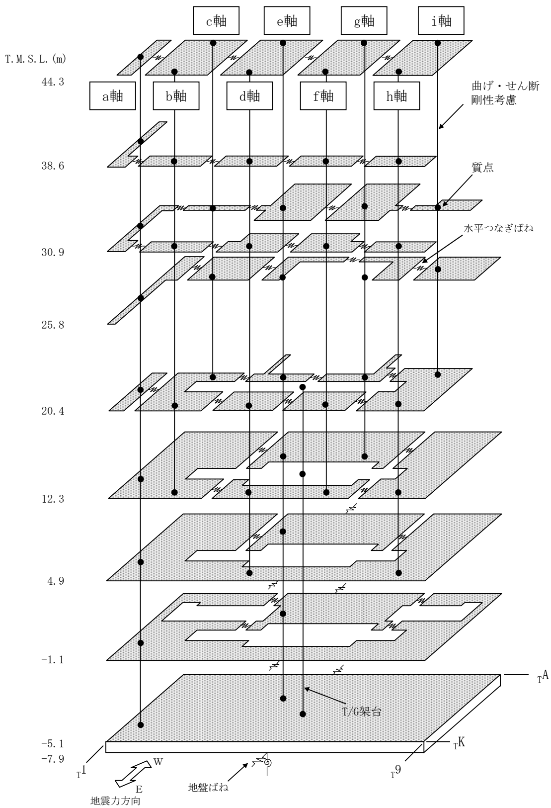
図 3-10 地震応答解析モデルの概念図 (EW 方向)
