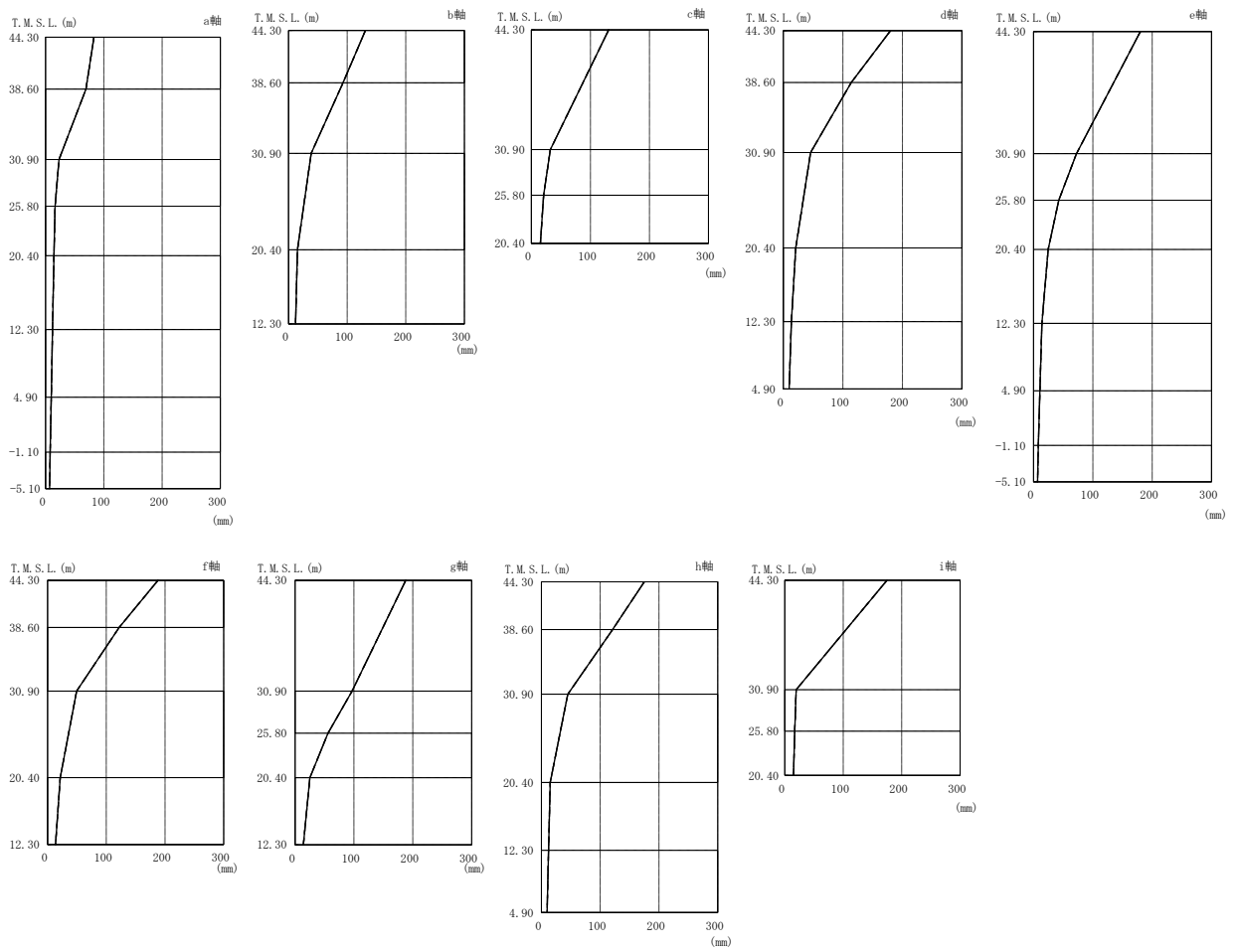
図 4-8 最大応答変位（基準地震動 S s，EW 方向）
