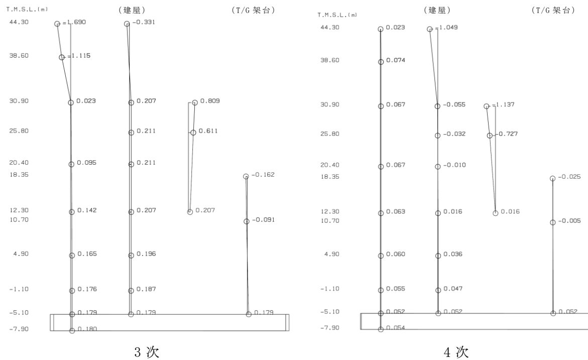
図 4-1 刺激関数図 (Ss-1, NS 方向) (1/4)
