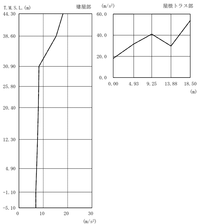
図 4-11 最大応答加速度（基準地震動 S s ，鉛直方向）
