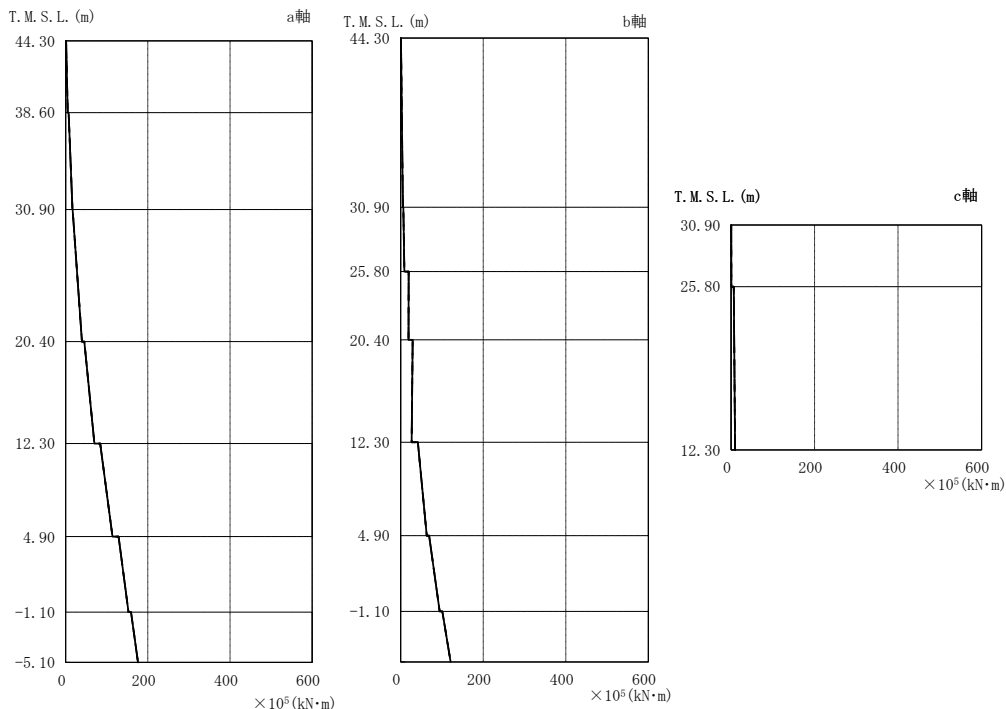
図 4-6 最大応答曲げモーメント（基準地震動 S s , NS 方向）
