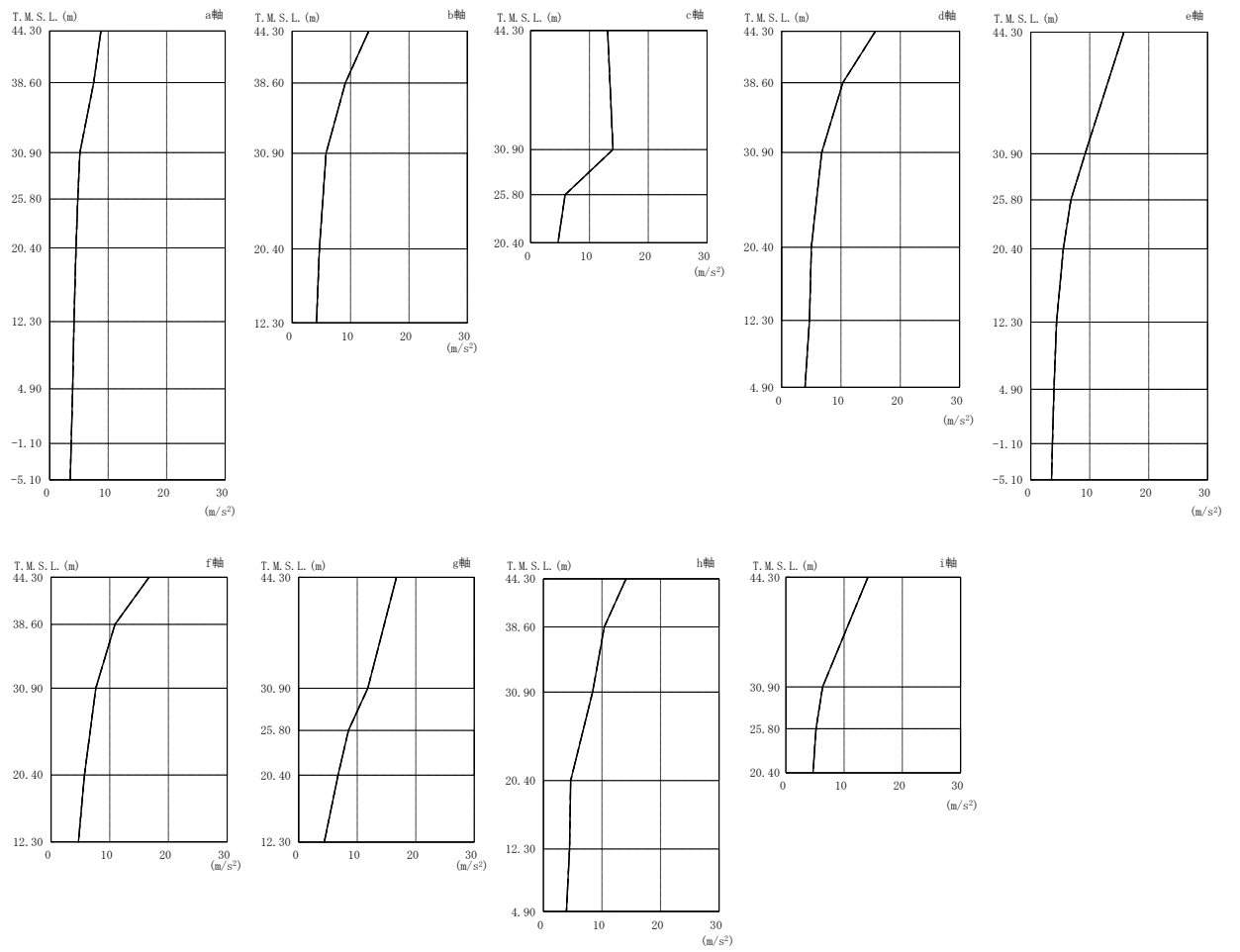
図 4-20 最大応答加速度（弾性設計用地震動 S d，EW 方向）
