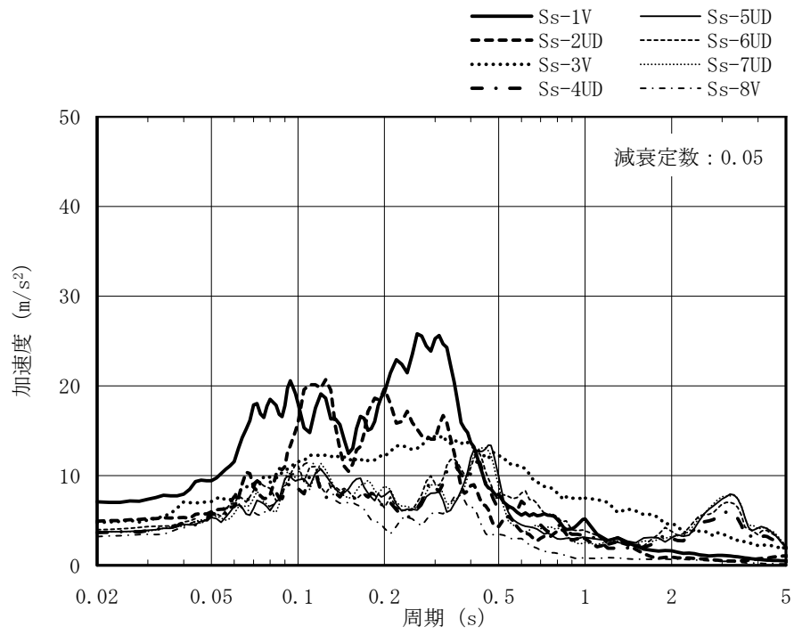
図 3-18 入力地震動の加速度応答スペクトル (基準地震動 S s , 鉛直方向, T.M.S.L. -7.9m)
