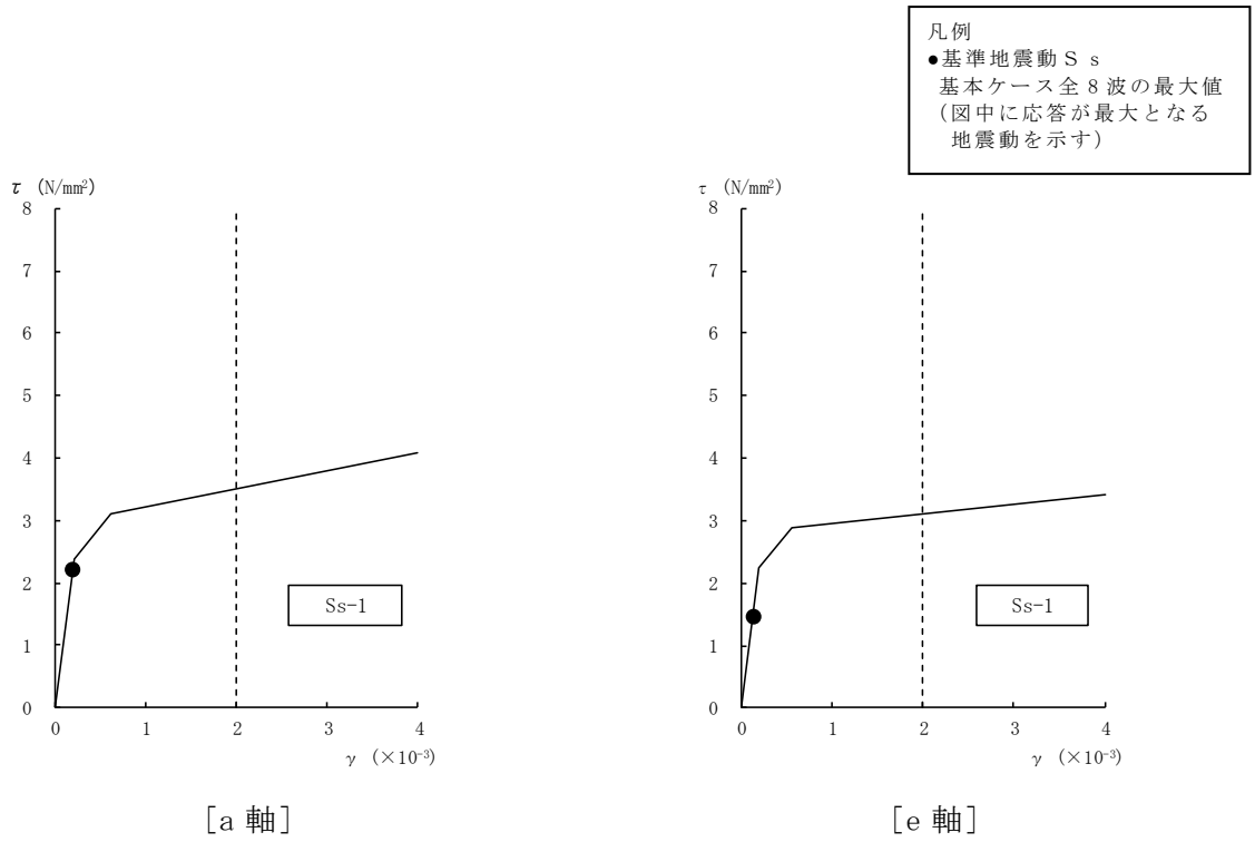
図 4-15 せん断スケルトン曲線上の最大応答値 (基準地震動 S s , EW 方向, MB2F)
