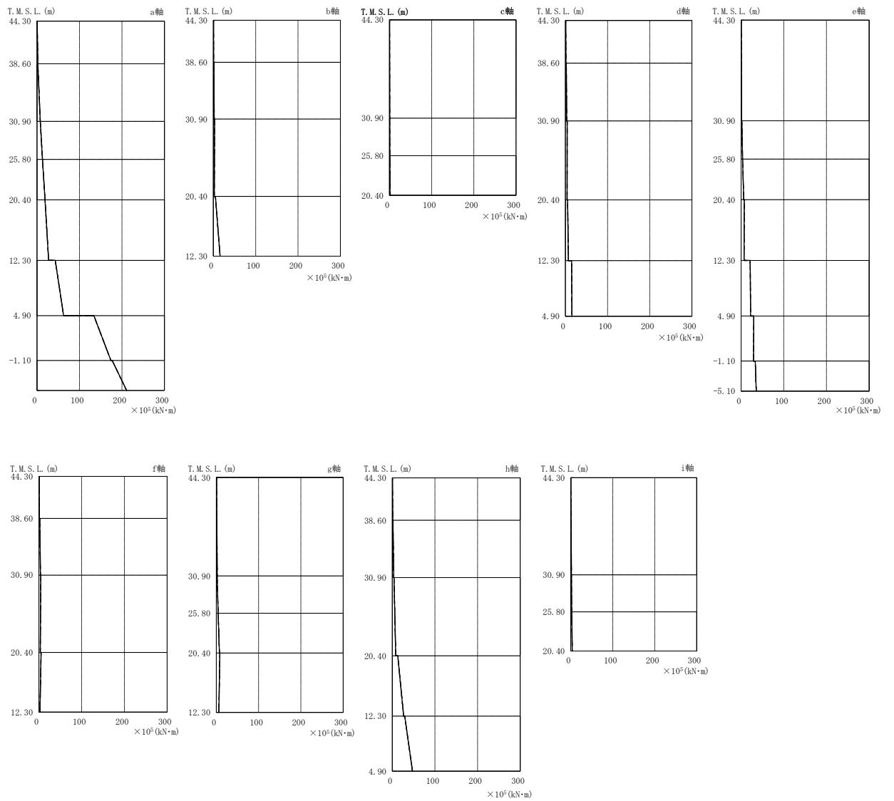
図 4-10 最大応答曲げモーメント（基準地震動 S s ，EW 方向）
