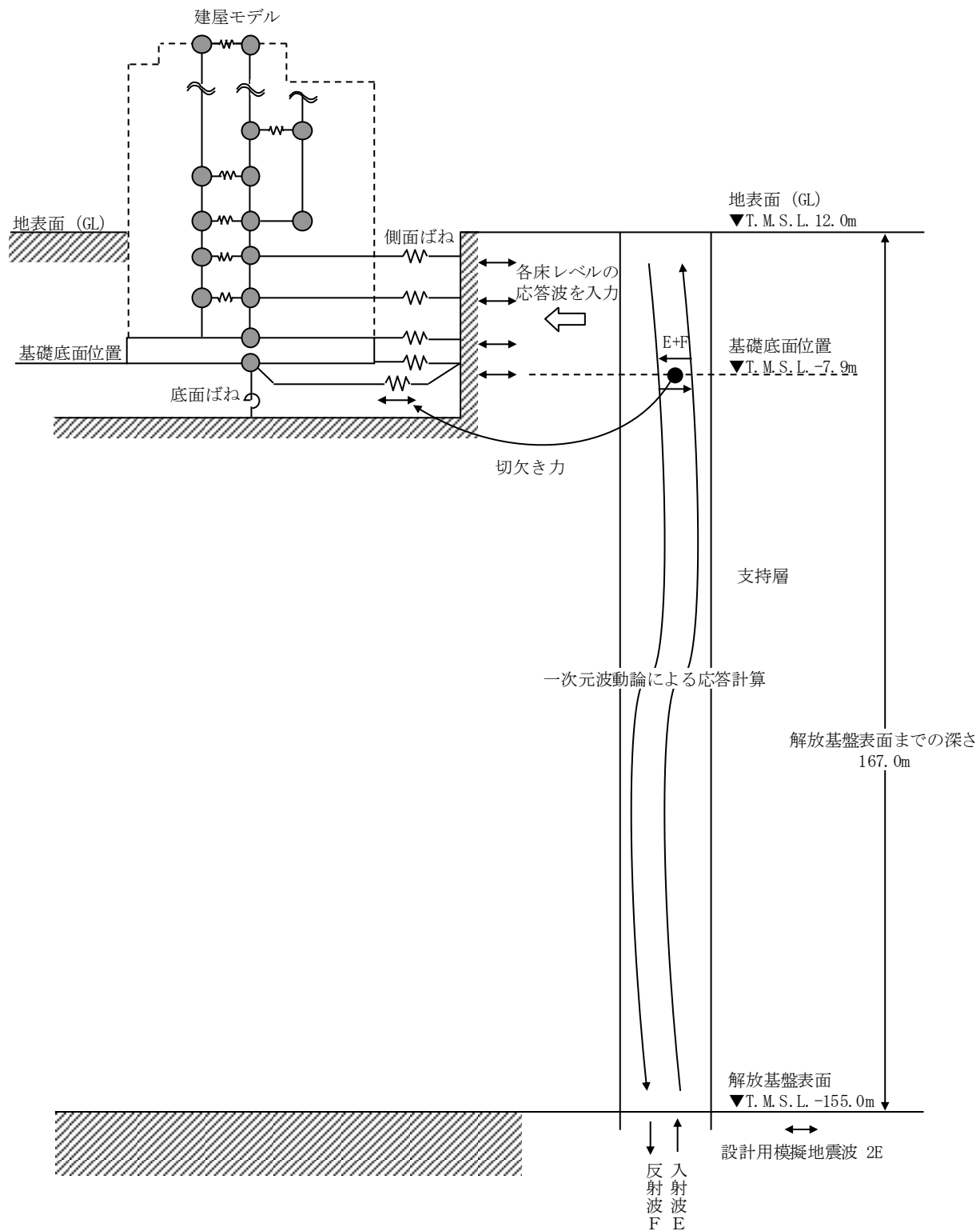
図 3-12 地震応答解析モデルに入力する地震動の概念図 (水平方向)
