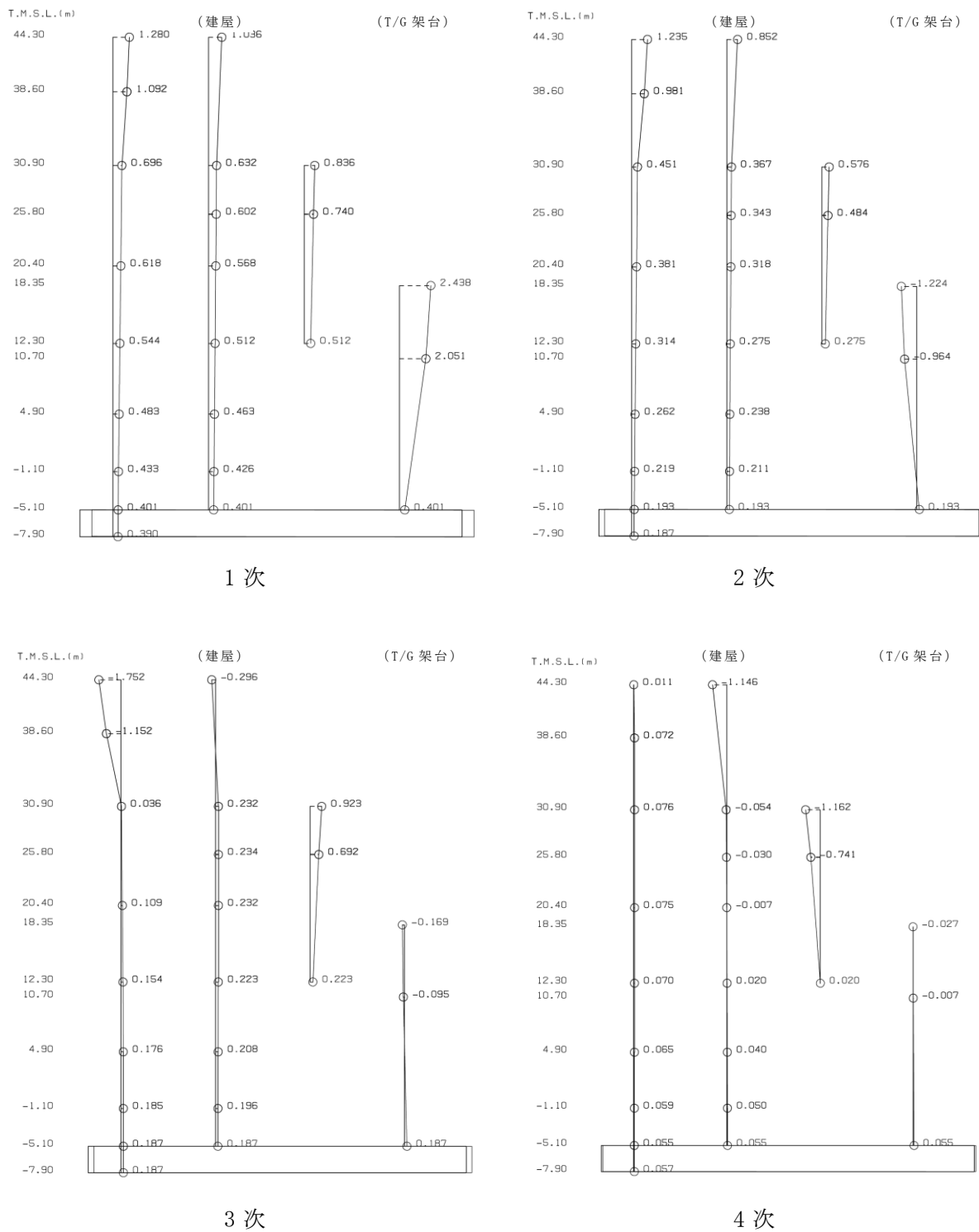
図 4-2 刺激関数図 (Sd-1, NS 方向) (1/4)
