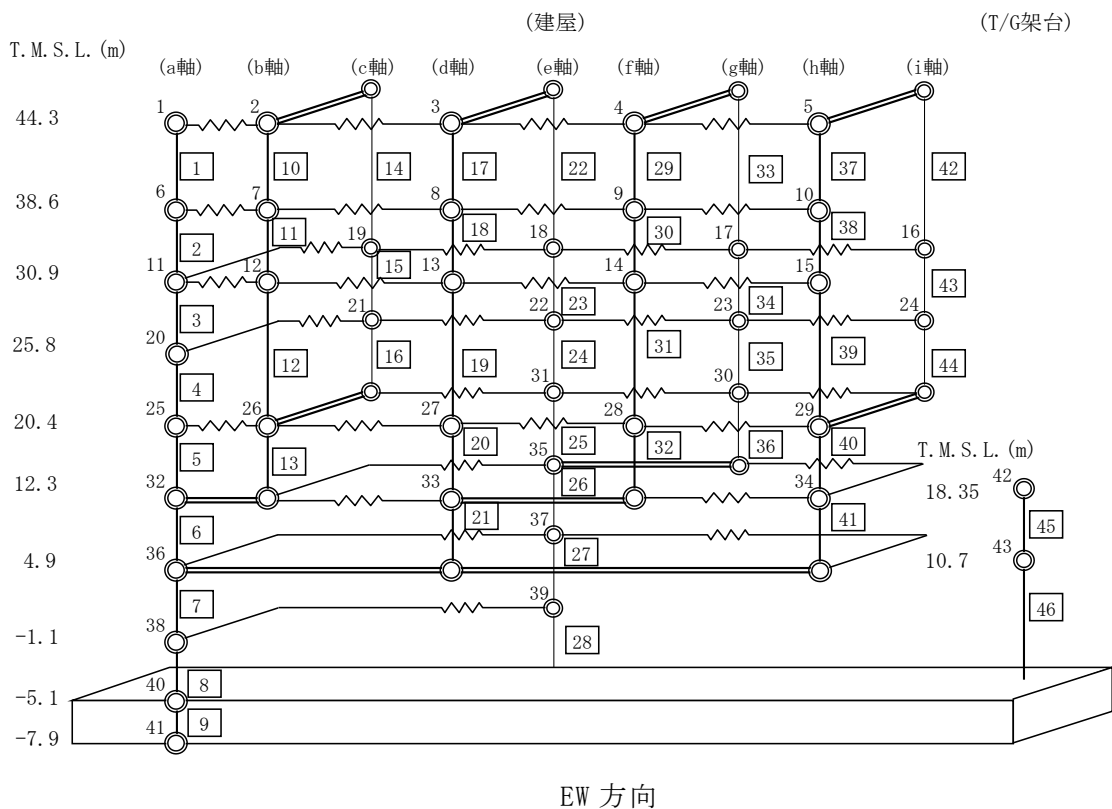
図 3-11 地震応答解析モデル (水平方向)
