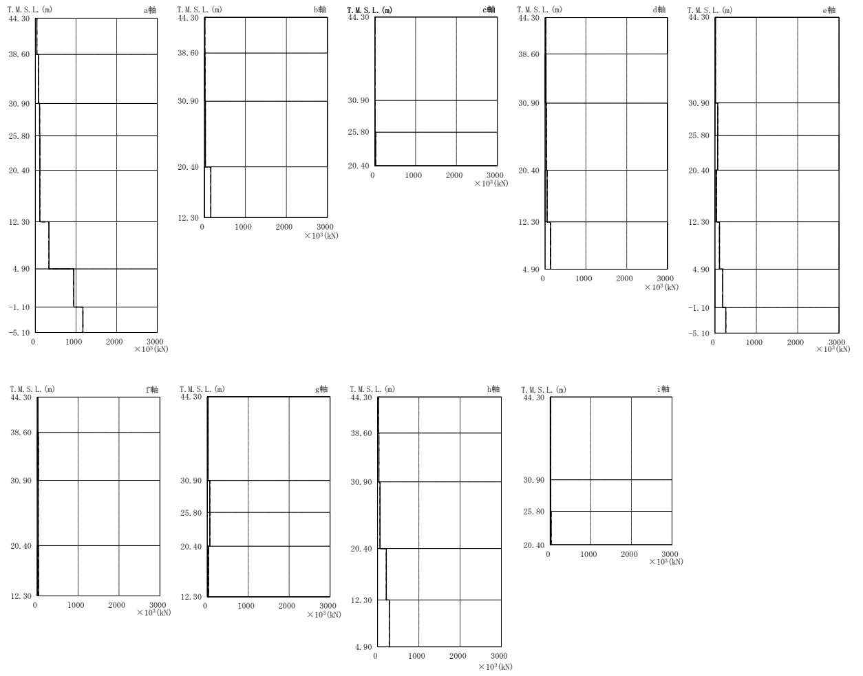
図 4-9 最大応答せん断力（基準地震動 S s ， EW 方向）
