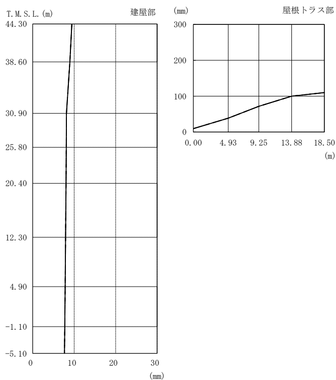
図 4-12 最大応答変位（基準地震動 S s ，鉛直方向）
