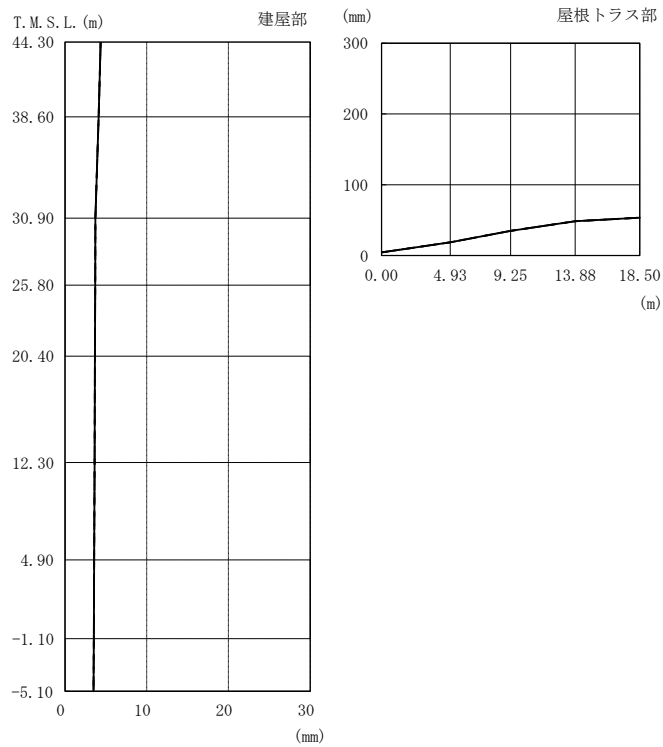
図 4-25 最大応答変位（弾性設計用地震動 S d，鉛直方向）
