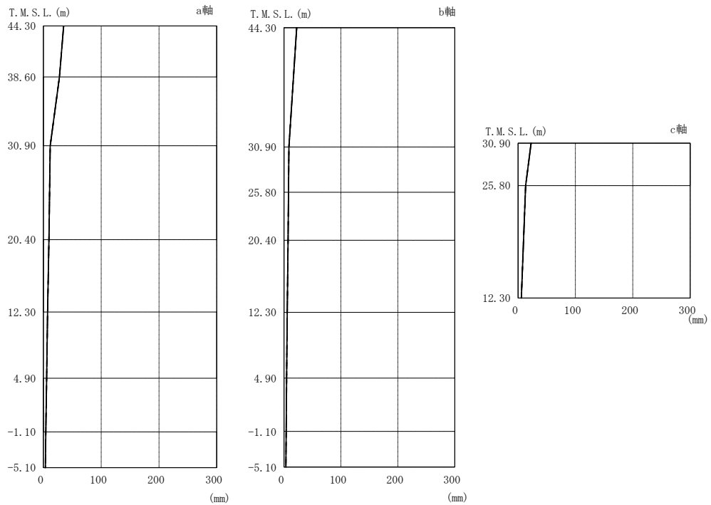
図 4-17 最大応答変位（弾性設計用地震動 S d，NS 方向）
