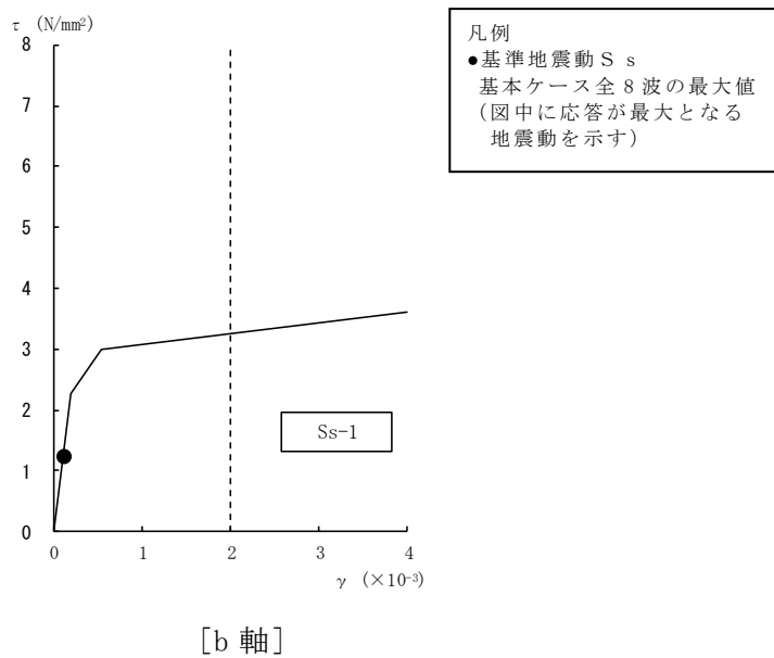
図 4-14 せん断スケルトン曲線上の最大応答値 (基準地震動 S s , NS 方向, 1F) (1/4)
