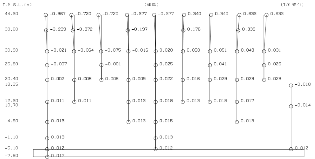
图 4-2 刺激関数図 (Sd-1, EW 方向) (3/4)
