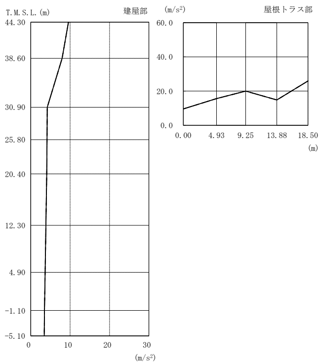
図 4-24 最大応答加速度（弾性設計用地震動 S d，鉛直方向）
