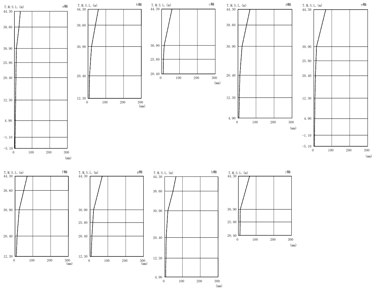
図 4-21 最大応答変位（弾性設計用地震動 S d，EW 方向）
