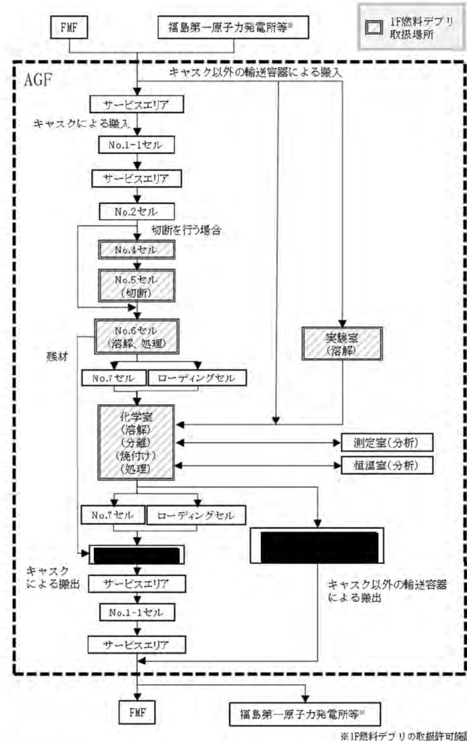
図-1 1F 燃料デブリ分析に関するフロー
