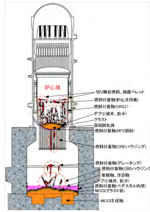
1Fで想定されるPCV内の状態
