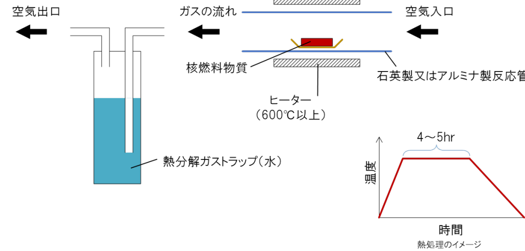
図-10 核燃料物質の安定化処理（酸化処理）
