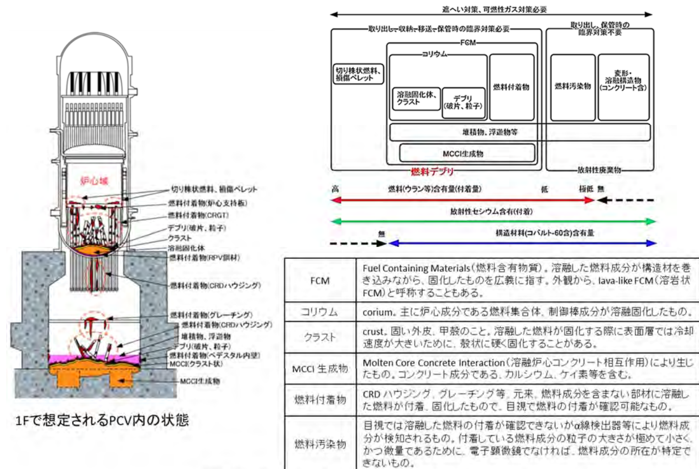
図-1 1F 燃料デブリの状態及び分類
