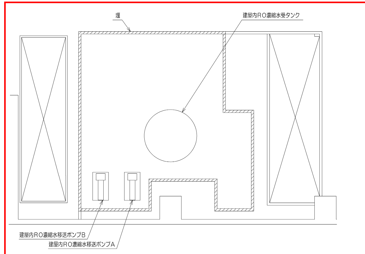
図-2 建屋内RO濃縮水受タンクの漏えい拡大防止 堰配置図
