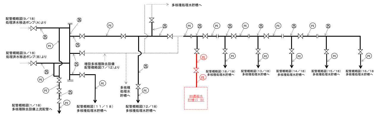
図-1 配管概略図 (10/18)
