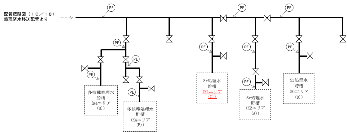
図-1 配管概略図 (10/18)
