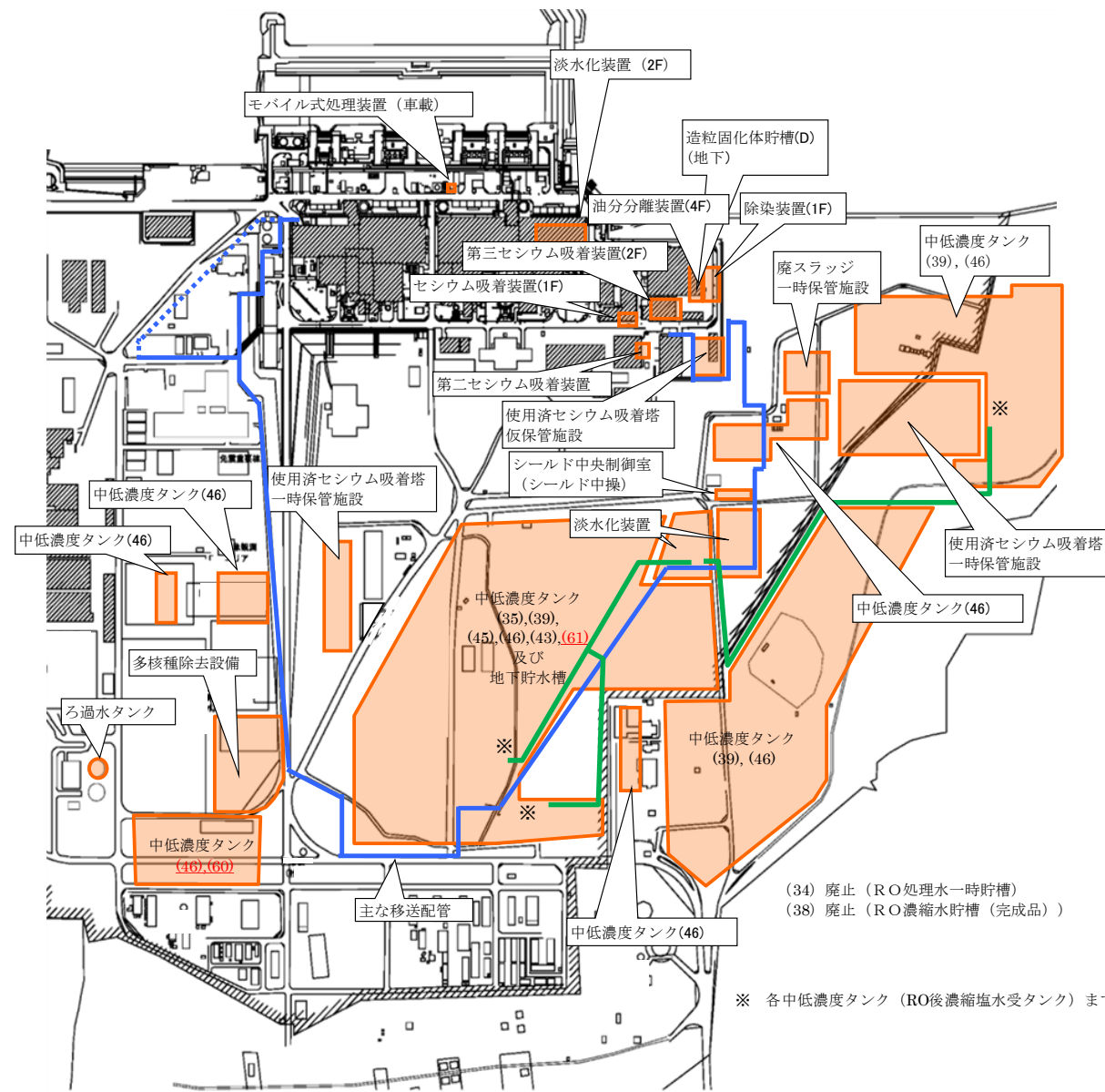
(b) 配置概要
