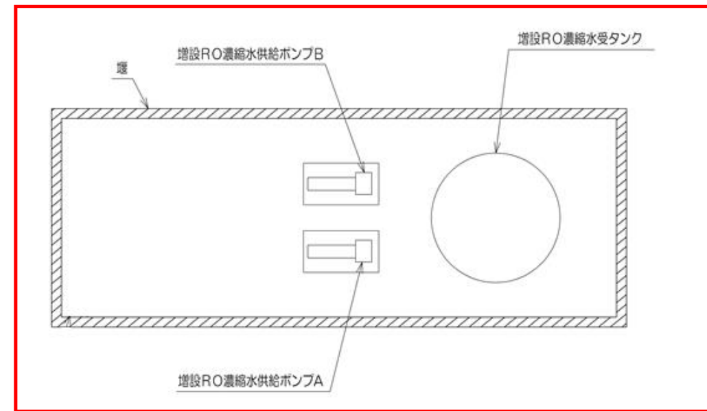
図-3 増設RO濃縮水受タンクの漏えい拡大防止 堰配置図
