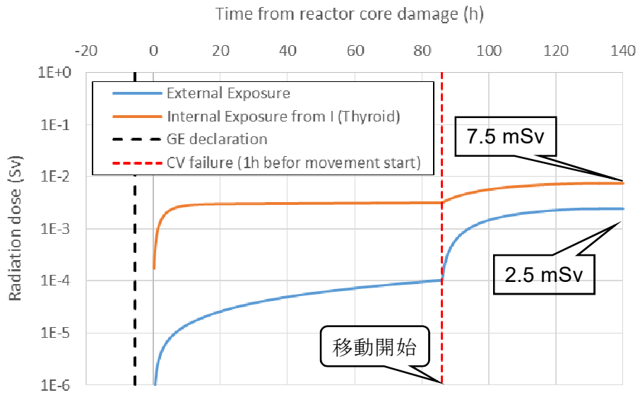
図 2.1.14 PWR 小破断 LOCA(SL-δ)時に格納容器破損後に移動開始した場合の被ばく線量の経時変化
