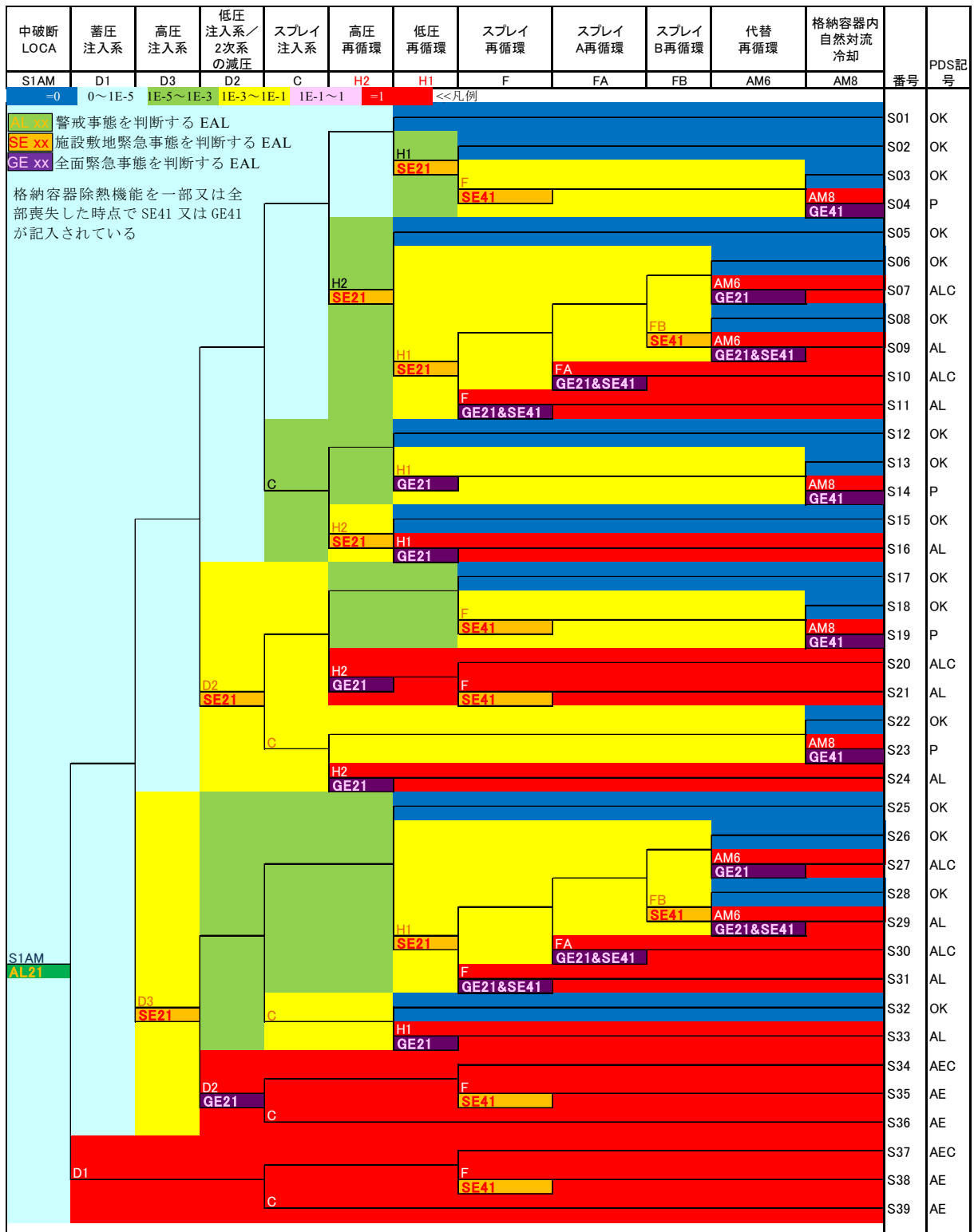
図 2.1.2 CCDP と EAL の ET へのマッピング例 (PWR 中破断 LOCA) Fig. 2.1.2 Example of CCDP and EAL mapping on event tree
