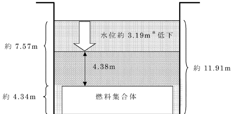
使用済燃料ピット水位概要図
