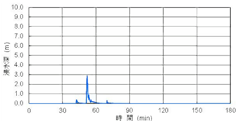
第 3.1.4.2.2.12 図 3，4号機建屋周辺エリアの津波水位変化
