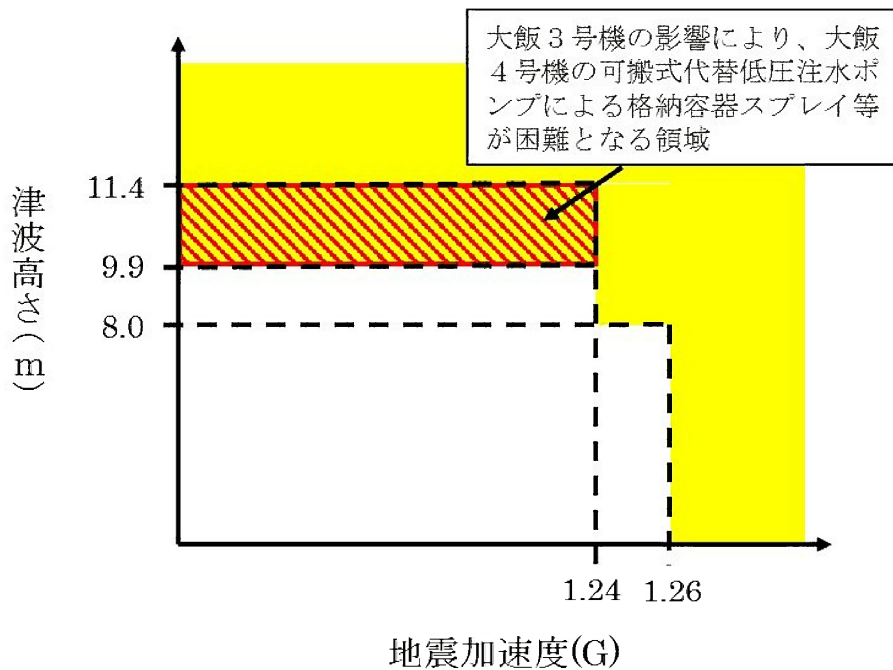
第 3.1.4.4.1.4 図 大飯 3 号機からの影響を考慮した大飯 4 号機の地震と津波の重畳に関するクリフエッジ評価結果（格納容器損傷）
