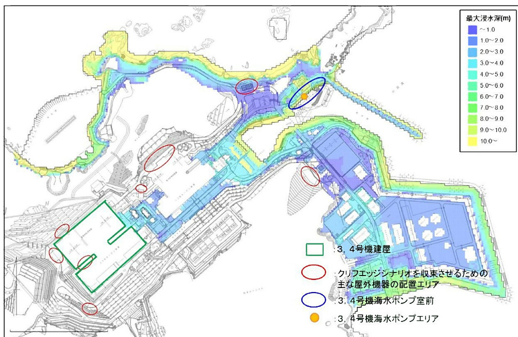
第 3.1.4.2.2.8 図 最大浸水深分布 (3, 4号機海水ポンプ室前潮位 : E.L.+11.4m)
