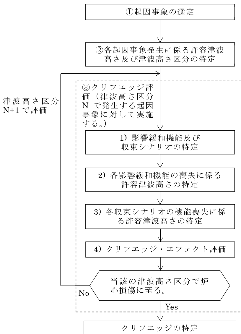
第 3.1.4.2.2.2 図 クリフエッジの特定に係るフロー図 (津波：運転停止時炉心損傷)
