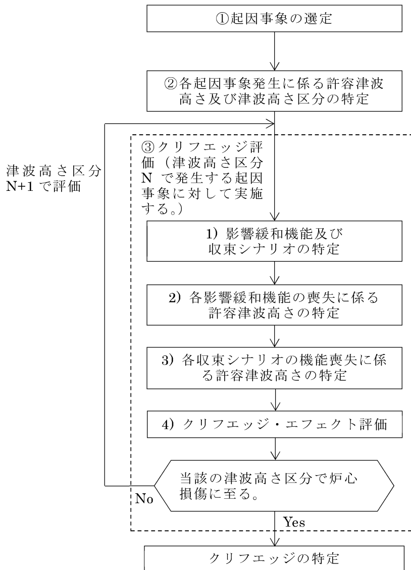
第 3.1.4.2.2.1 図 クリフエッジの特定に係るフロー図 (津波：出力運転時炉心損傷)
