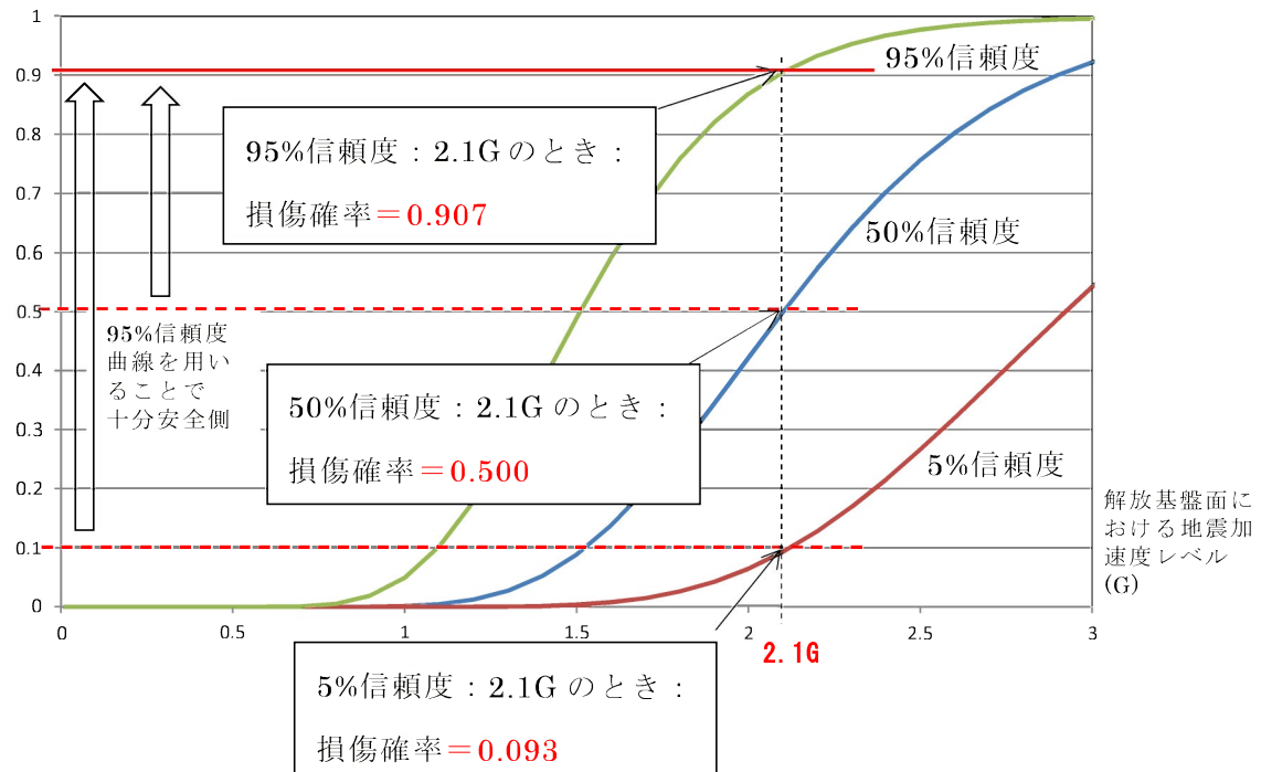
第 3.1.4.1.2.2 図 各信頼度における fragility 曲線 注)
