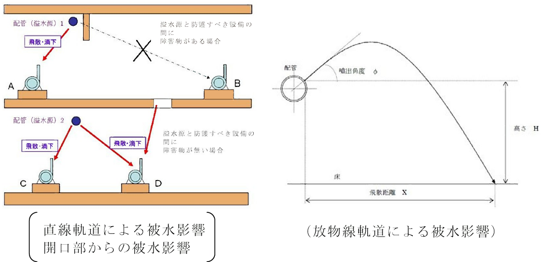
第 3.1.4.2.1.5 図 被水影響範囲の考え方
