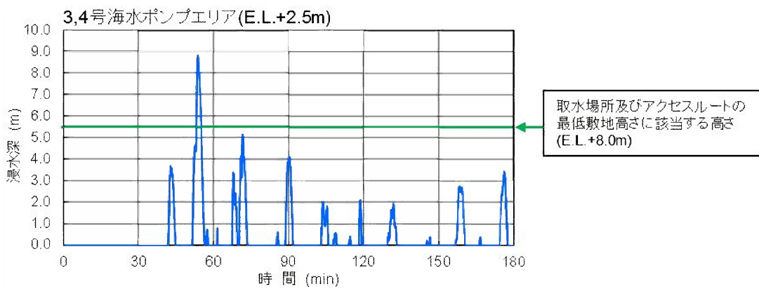
第 3.1.4.2.2.10 図 3, 4号機海水ポンプエリア(E.L.+2.5m) の津波水位変化
