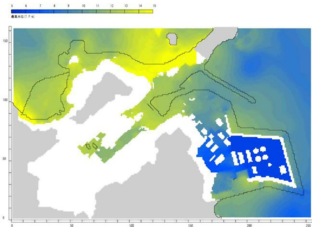
第 3.1.4.2.2.7 図 最高水位分布 (3, 4号機海水ポンプ室前潮位 : E.L.+11.4m)
