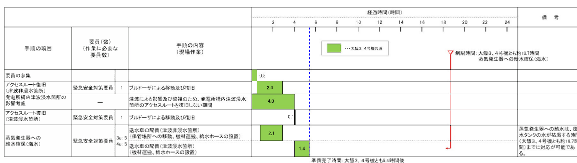
第 3.1.4.3.1.3 図 2 次系冷却継続のための海水の復水ピット補給の 対応手順と所要時間
