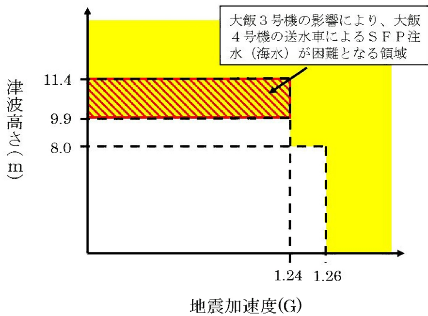
第 3.1.4.4.1.5 図 大飯3号機からの影響を考慮した大飯4号機の地震と津波の重畳に関するクリフエッジ評価結果 (SFP燃料損傷)
