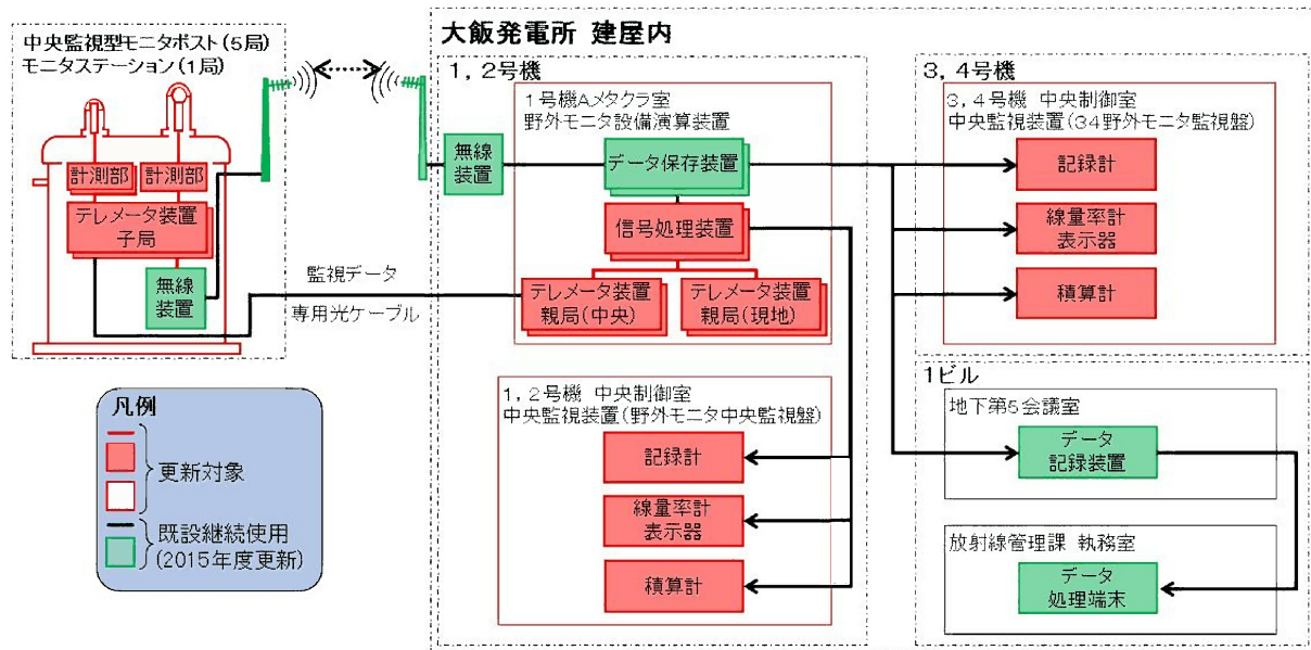
第 2.4.6 図 野外モニタ装置取替の説明図
