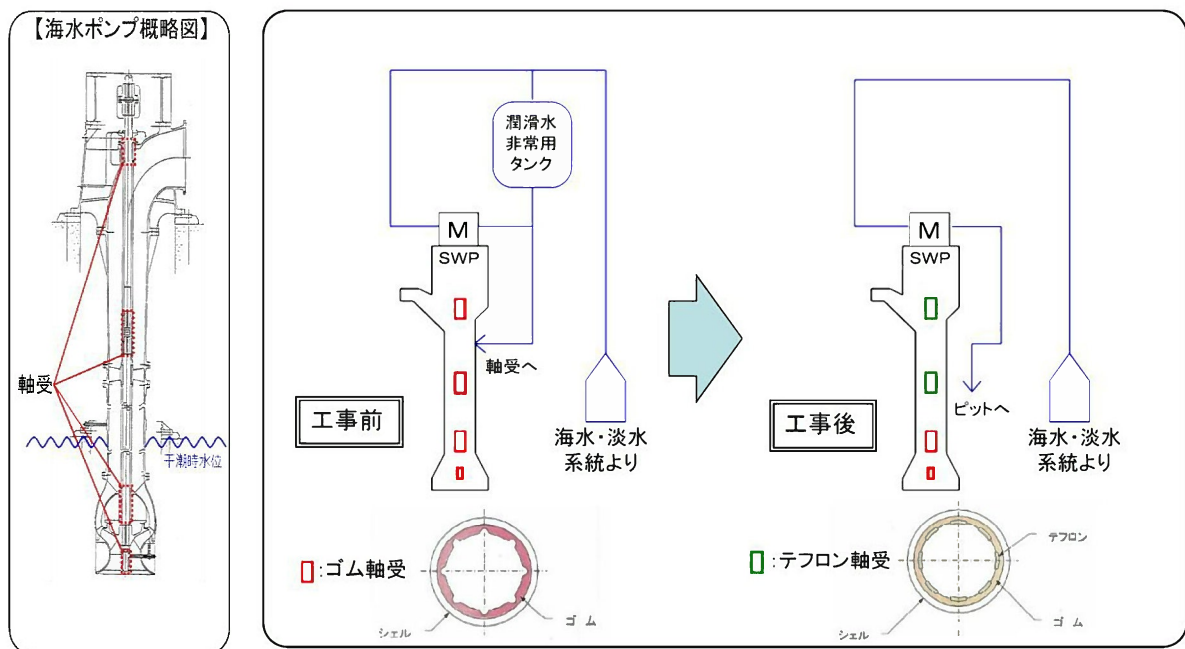
第 2.4.2 図 海水ポンプ（SWP）軸受取替の説明図
