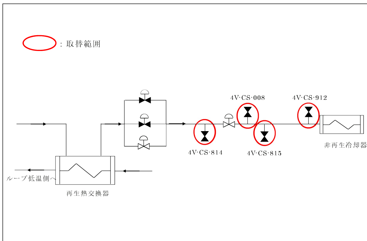
第 2.4.3 図 O 2 SCC 配管取替の説明図
