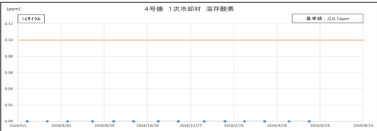
第 2.2.1.2.13 図 水質データの推移 (1 / 2)
