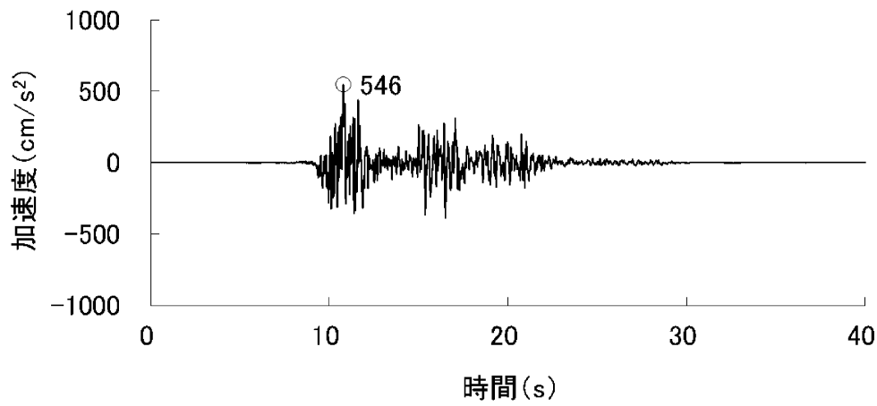
加速度（水平方向：S s -4 H (NS)）
