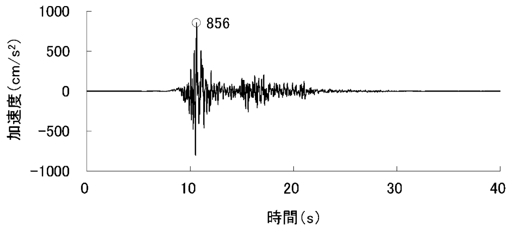
加速度（水平方向：S s -4 H (EW)）
