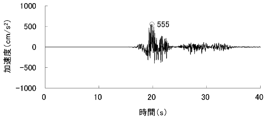
加速度（水平方向：S s -8 H (EW)）
