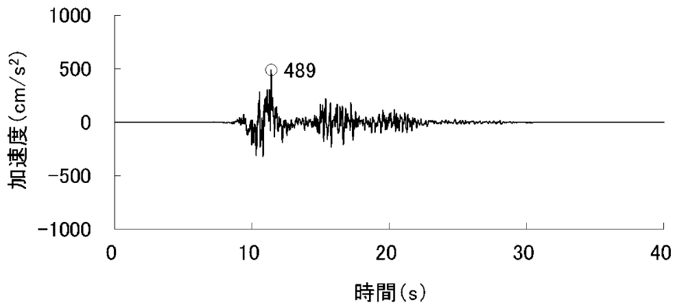
加速度（水平方向：S S -9 H (NS)）
