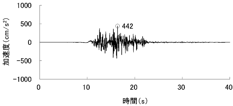
加速度（水平方向：S s -7 H (NS)）
