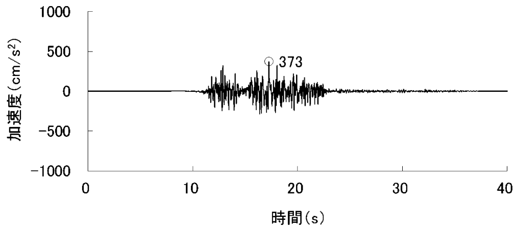
加速度（鉛直方向：S s -7 V ）
