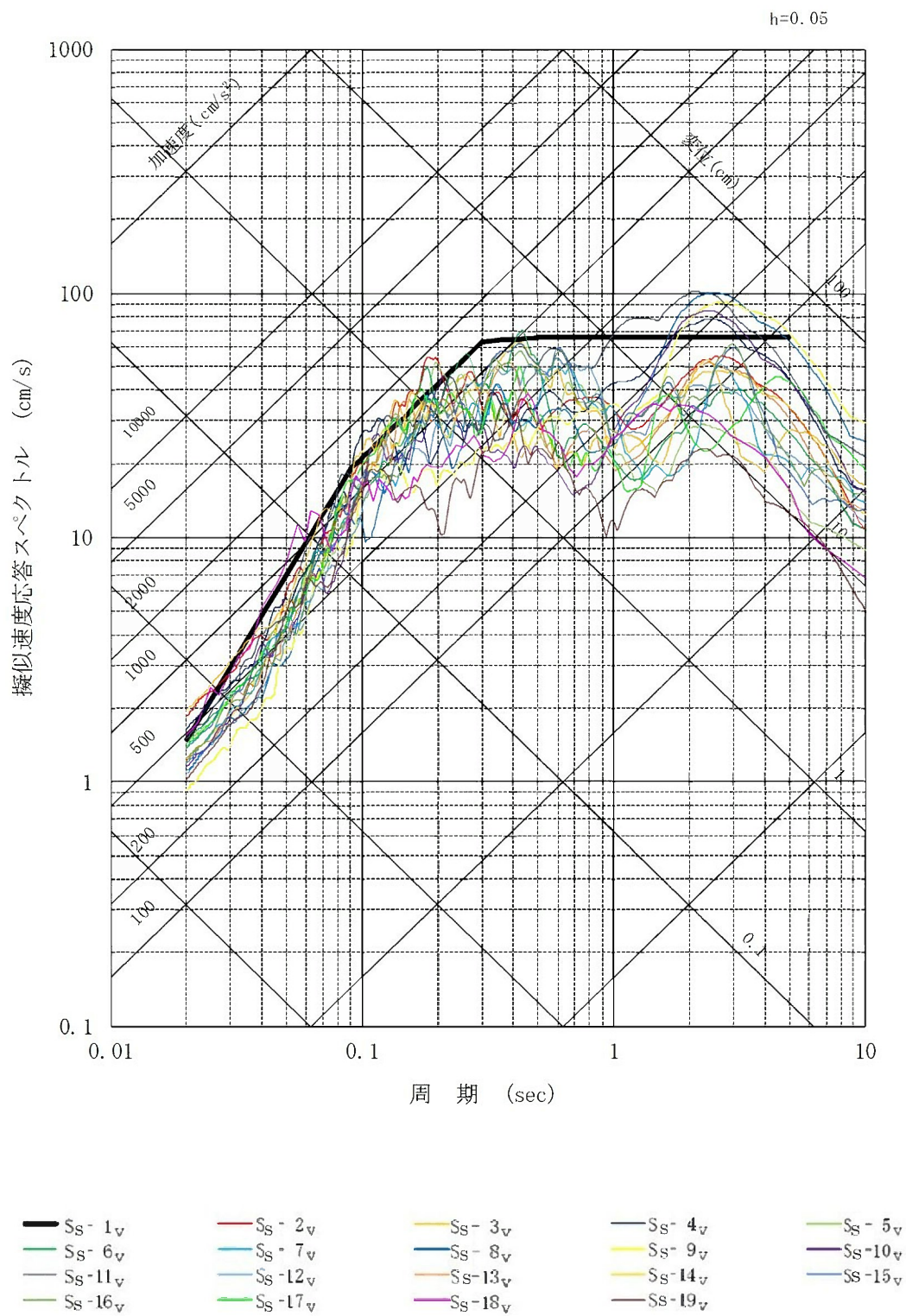
第 1.3.2.2 図 基準地震動 S S の応答スペクトル (鉛直方向)
