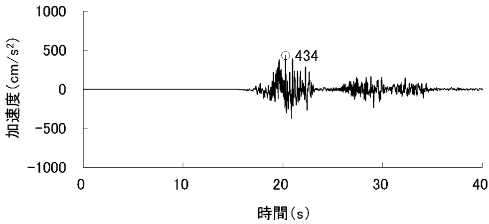
加速度（水平方向：S s -8 H (NS)）
