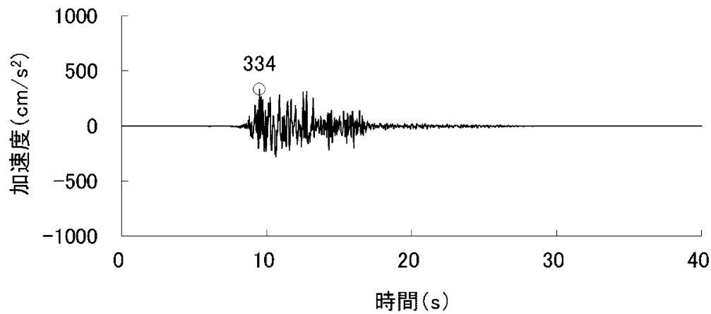
加速度（鉛直方向：Ss-12 V ）
