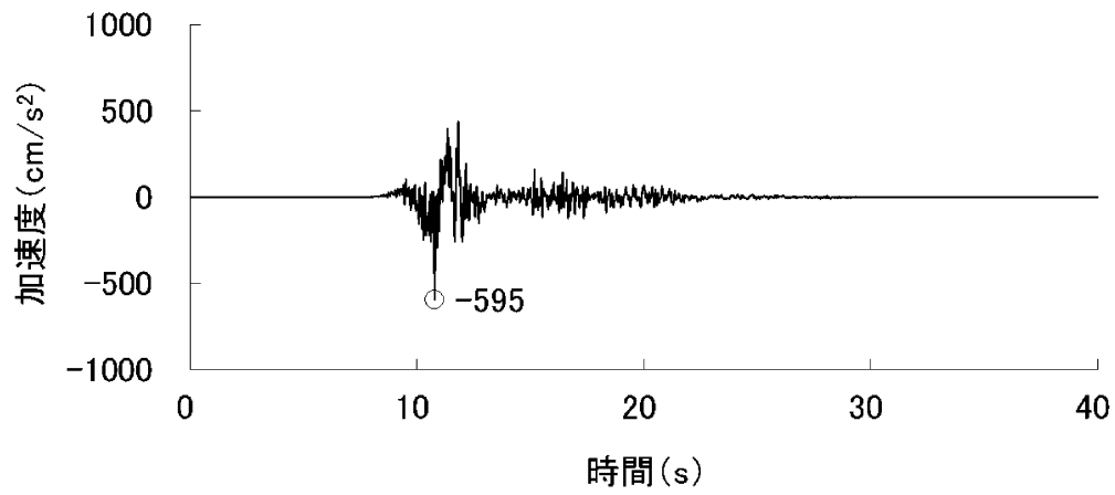
加速度（水平方向：S S -9 H (EW)）
