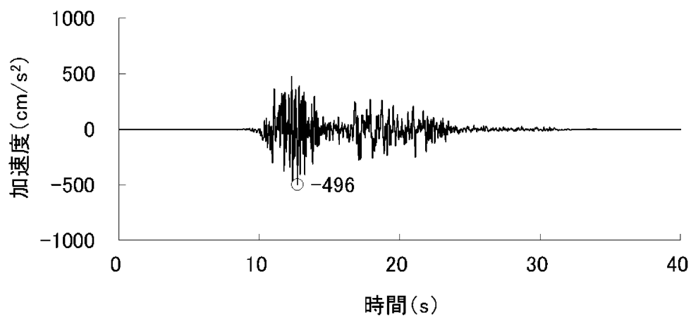
加速度 (水平方向 : S s -3 H (NS))
