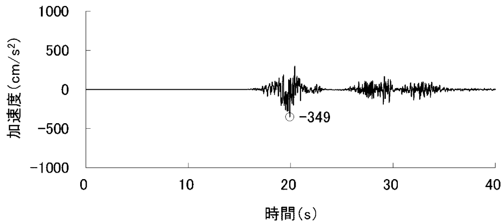
加速度（鉛直方向：S s -8 V ）
