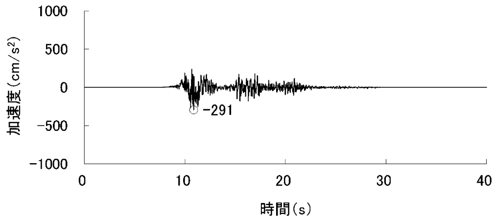
加速度（鉛直方向：S S -9 V ）
