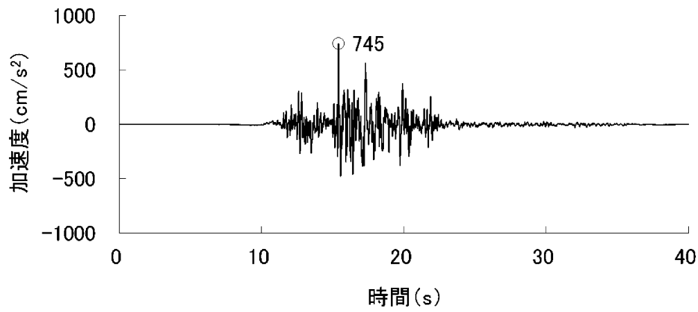
加速度（水平方向：S s -7 H (EW)）
