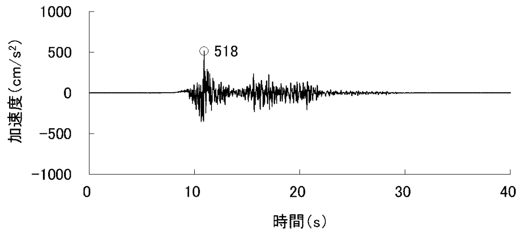
加速度（鉛直方向：S s -4 V ）
