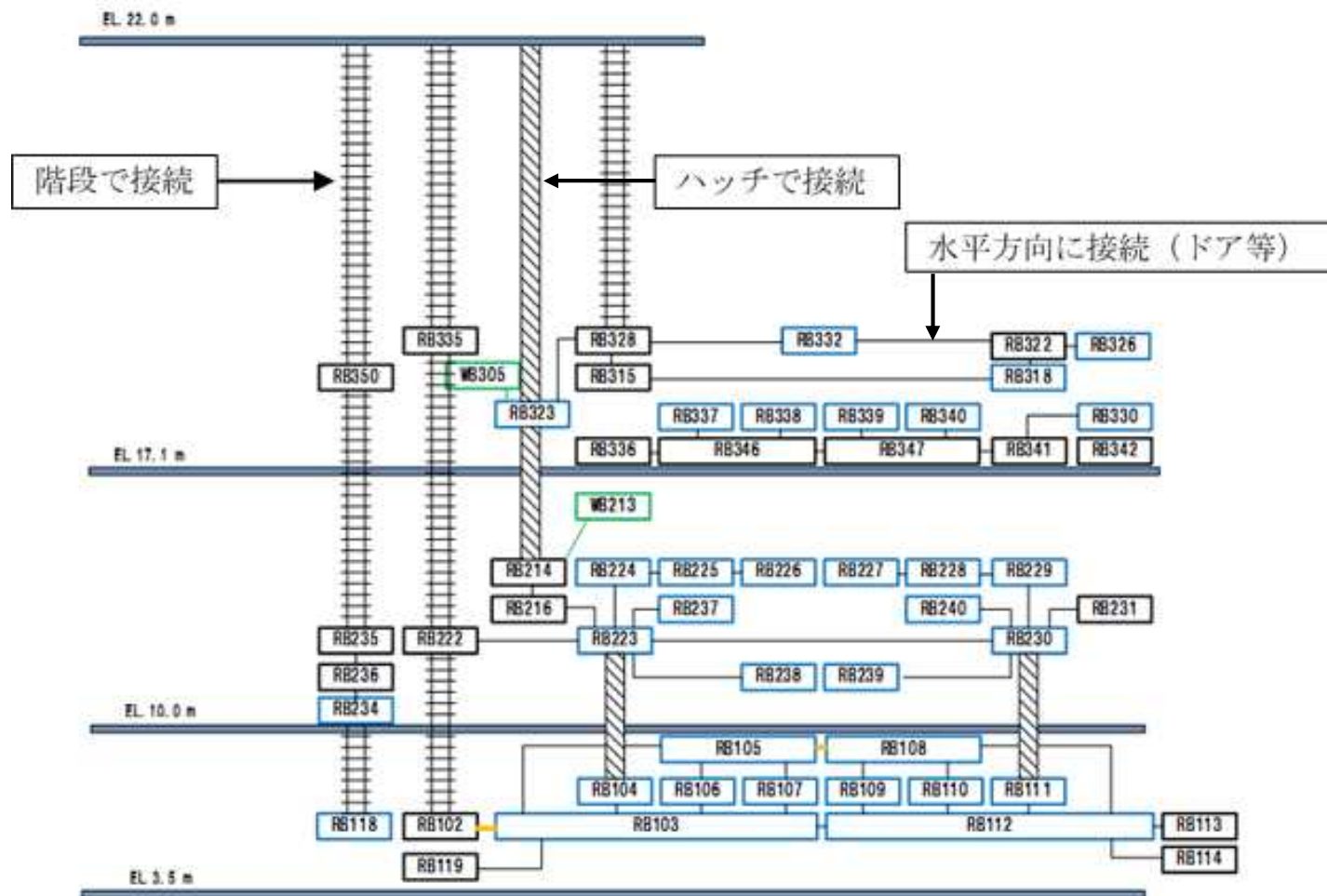
図2 浸水解析コードのモデルの階層概念図
