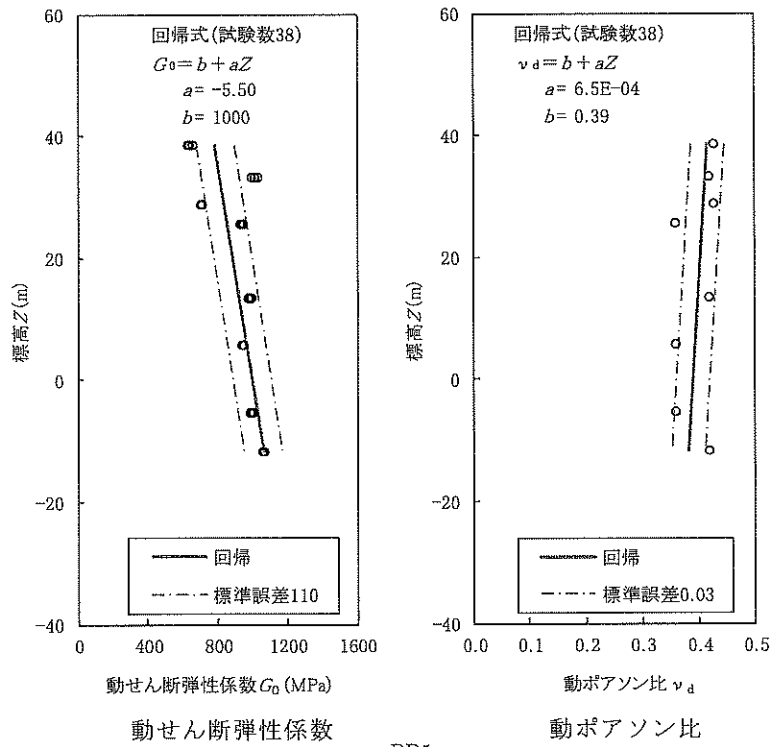
第 4.5-16 図(5) 動的変形特性
