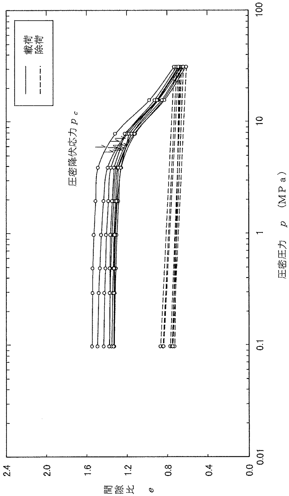
第 4.5-11 図(3) 圧密試験による間隙比—圧密圧力曲線 (鷹架層上部層)
