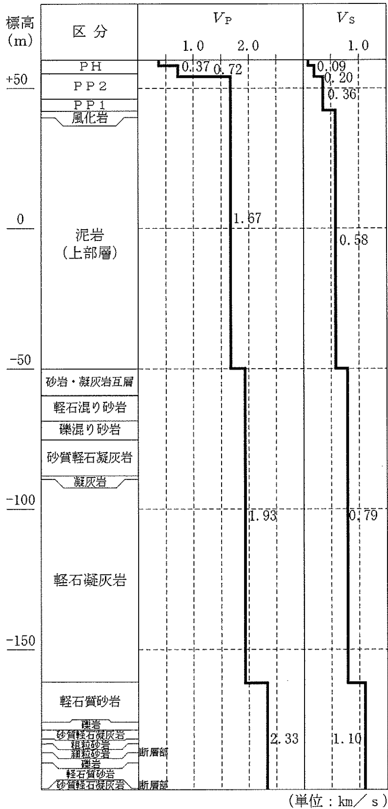
第 4.5-15 図(8) P S 檢層結果 (J-T 孔)
