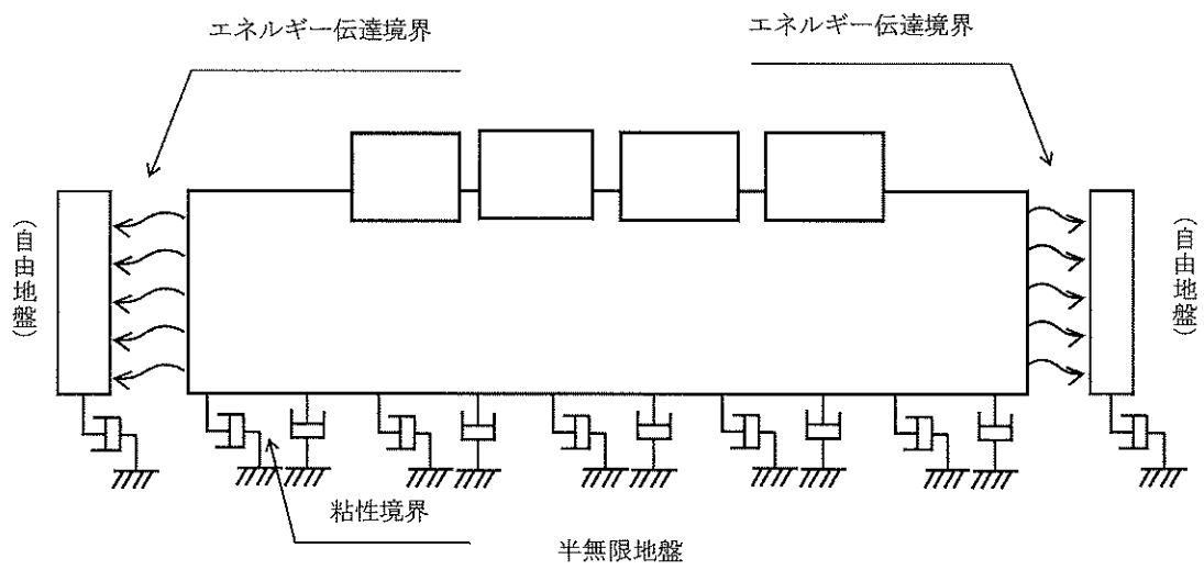
地震時解析
