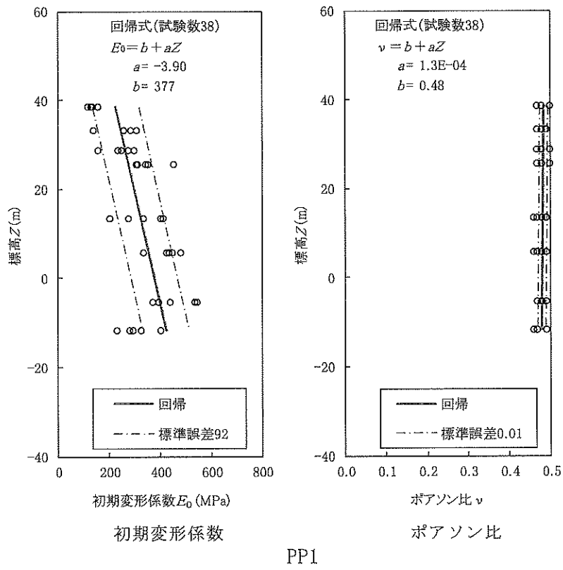
第 4.5-10 図(7) 静的変形特性 (初期変形係数及びポアソン比と標高の関係)
