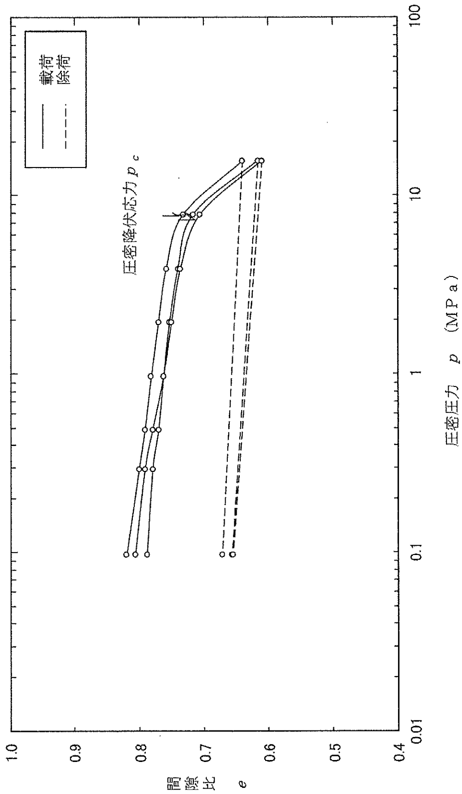
第 4.5-11 図(1) 圧密試験による空隙比-圧密圧力曲線 (鷹架層下部層)
