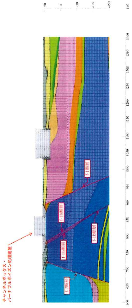
第 4.6-2 図(19) 解析用要素分割図(P-P断面)
