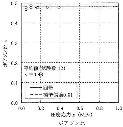
埋戻し土
