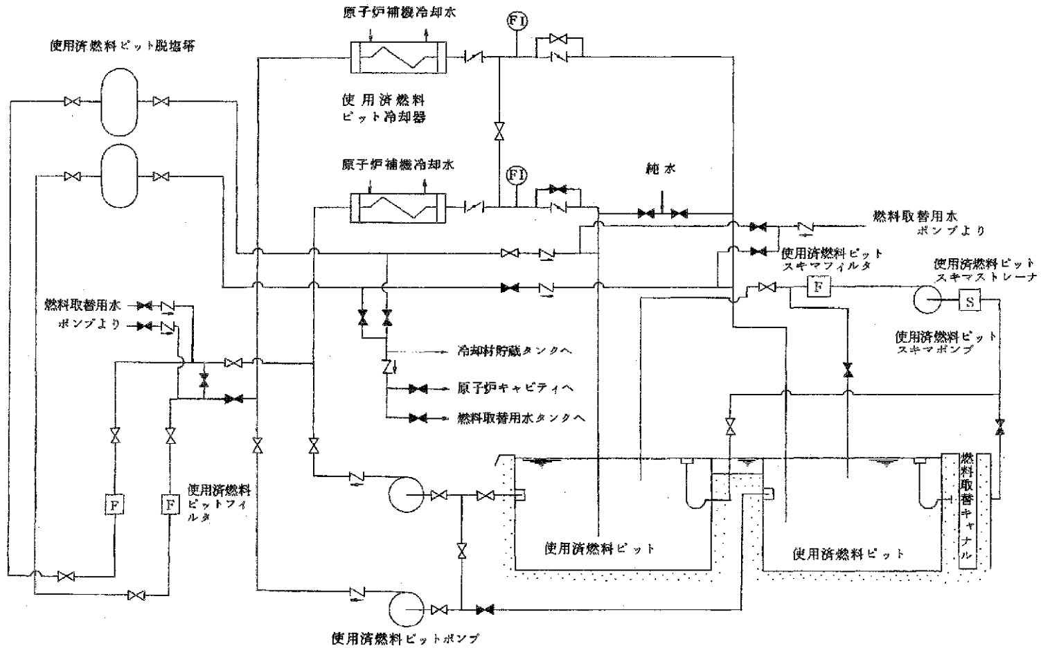
第1.9-3図 使用済燃料ピット水浄化冷却設備系統説明図(3号機)
