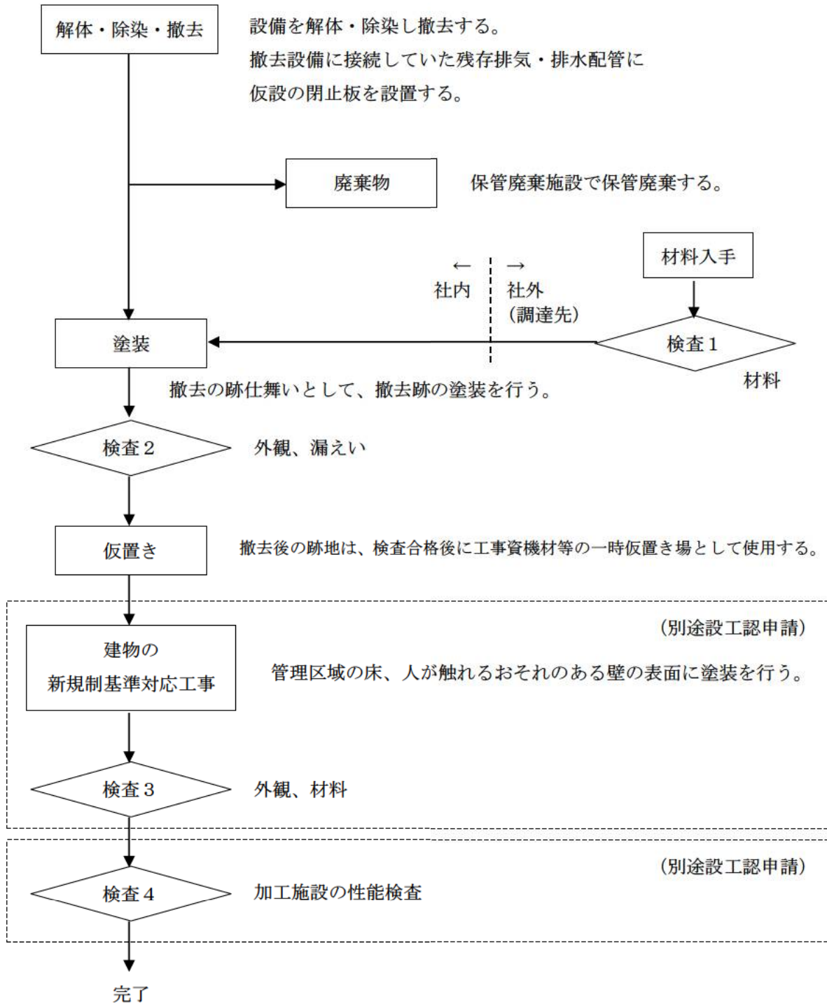
図リー-1 洗濯室の洗濯機の工事フロー
