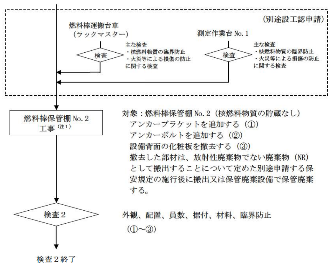
図へー1 燃料棒保管棚 No. 1, No. 2 の工事フロー (1 / 3)
