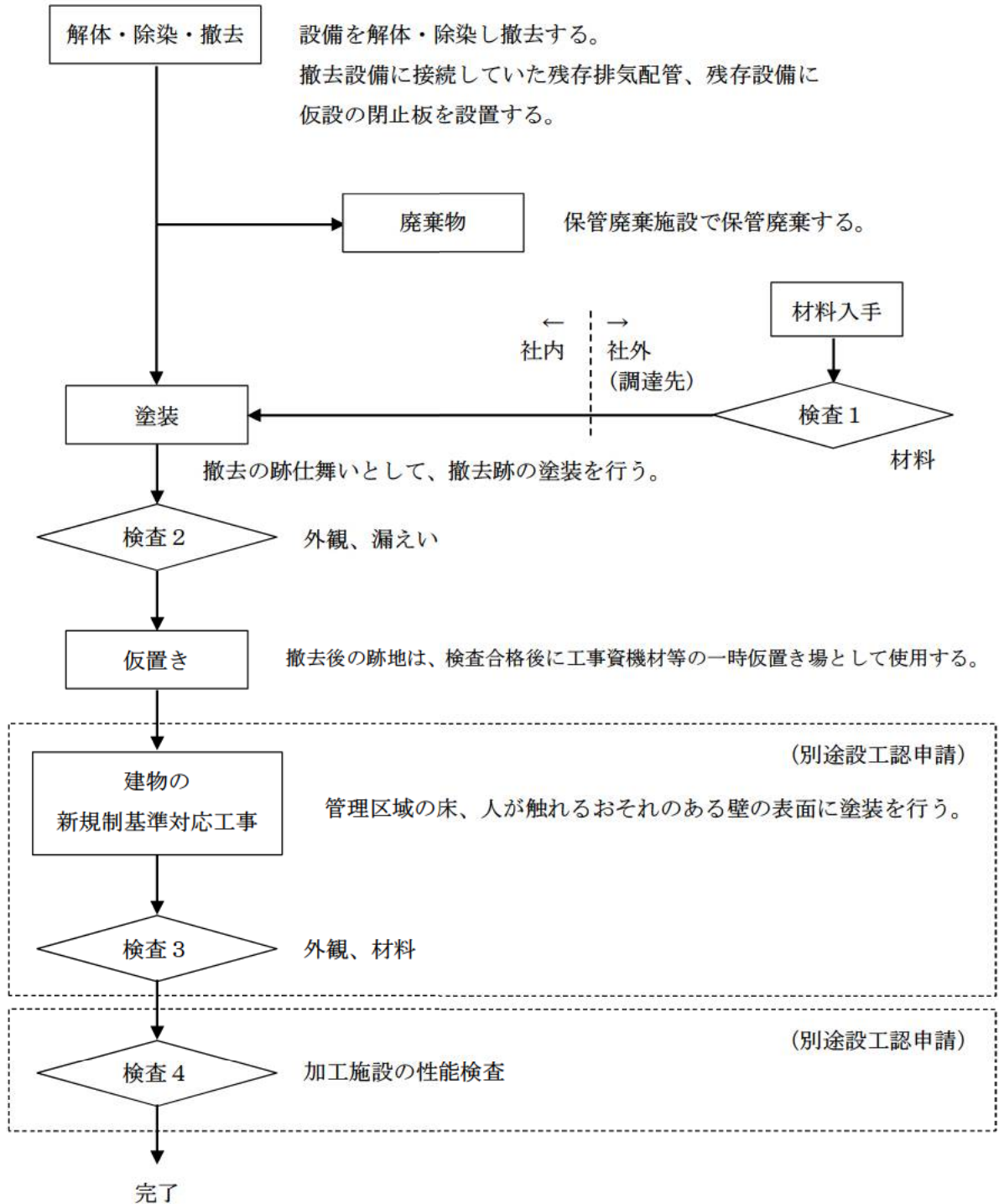
図ハー1 粉末調整室及びペレット加工室RI内の成型施設の工事フロー
