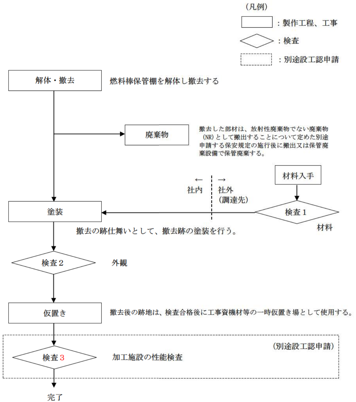
図へー4 燃料棒保管棚の工事フロー
