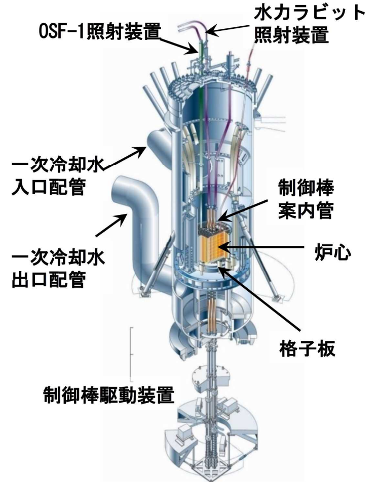
原子炉容器概要図
