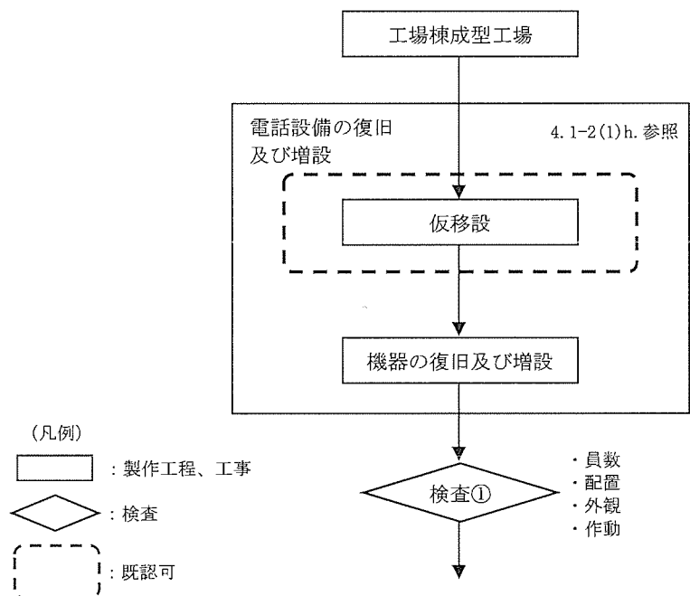
(図ハ1-1 工事の手順フロー図へ)
