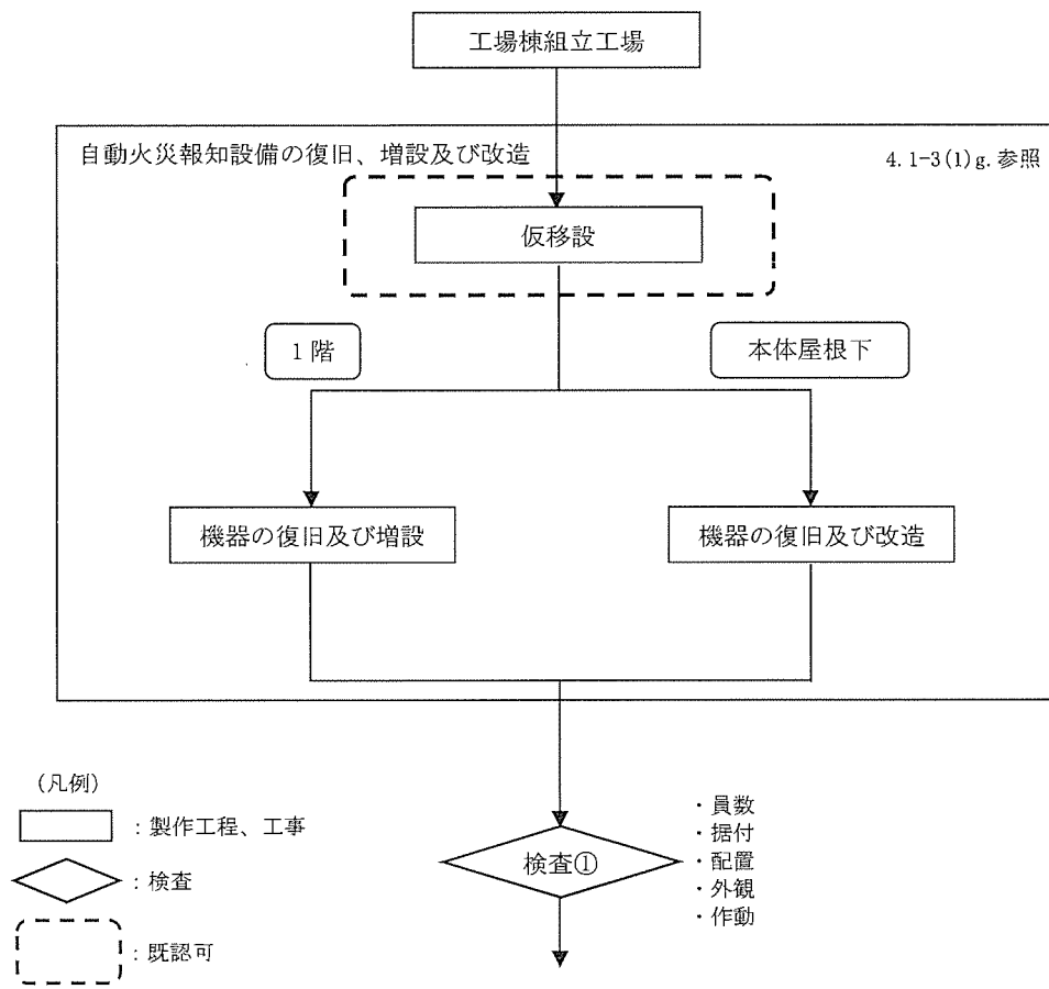
(図ホ 1-1 工事の手順フロー図へ)
