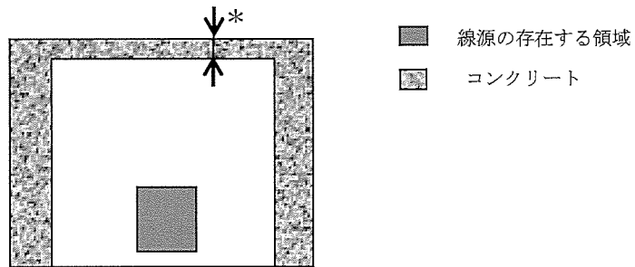
(建物断面方向の計算概念図)
