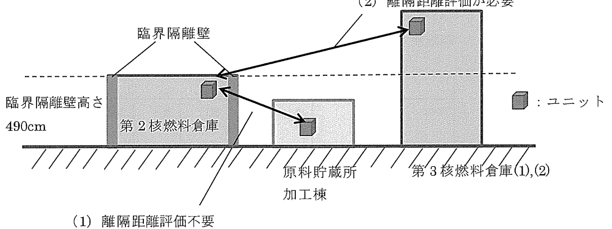
添説建 8-3 図 第2核燃料倉庫領域と原料貯蔵所、加工棟、第3核燃料倉庫(1),(2)の領域の相互干渉評価(模式図)
