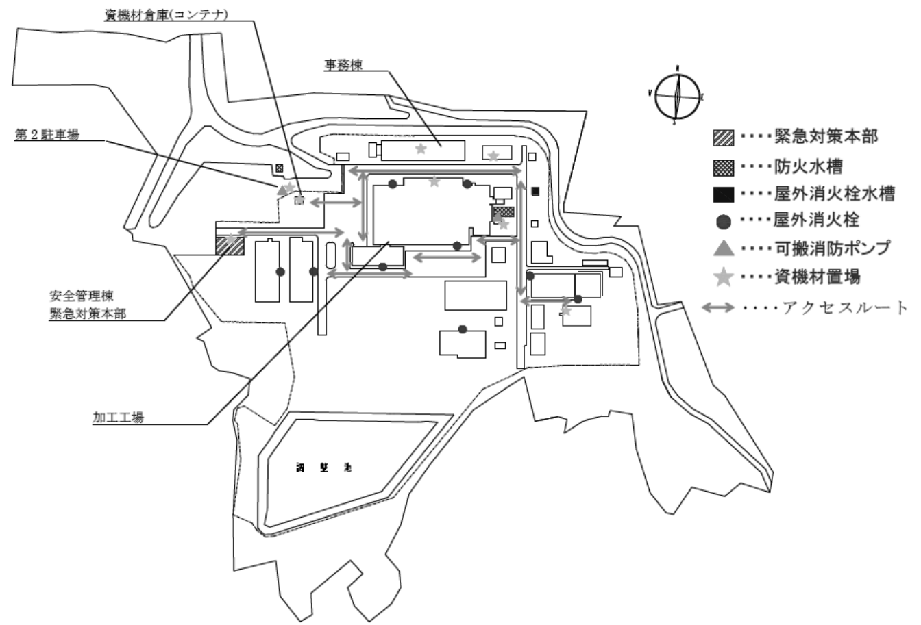
添2の図2 資機材保管場所とアクセスルート
