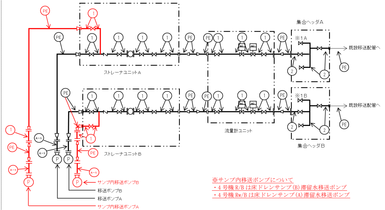
図-1 配管概略図 (9/11) (4号機 R/B,Rw/B)
