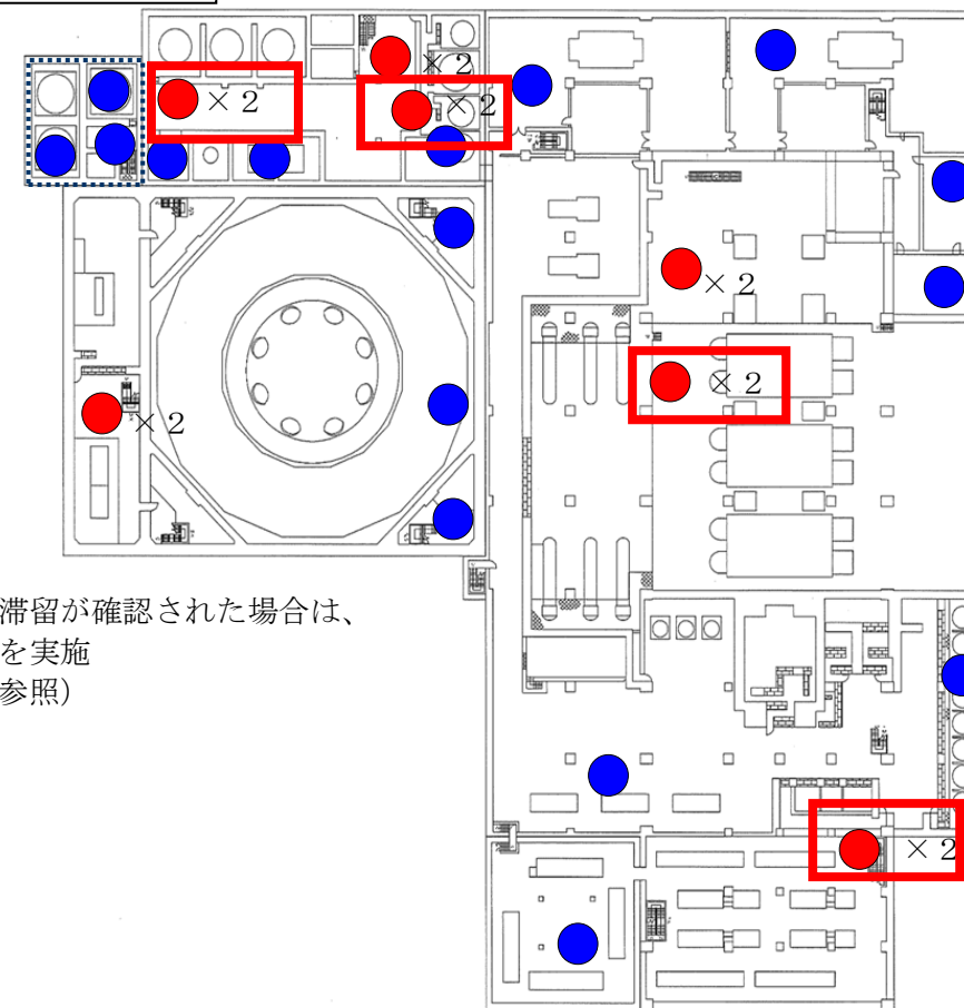
図5 3号機水位計設置位置図
