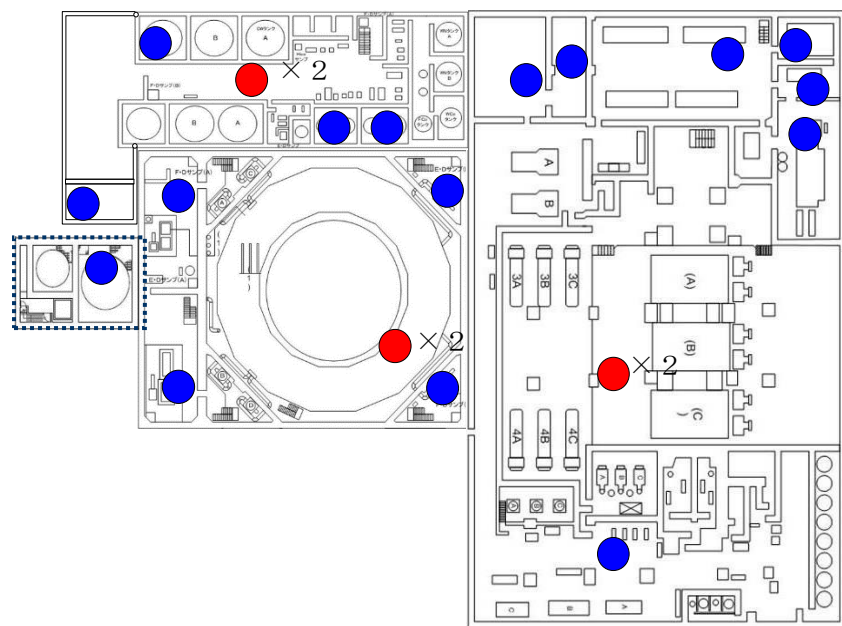
図6 4号機水位計設置位置図
