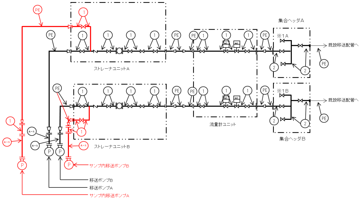
図-1 配管概略図 (8/11) (4号機 I/B)
