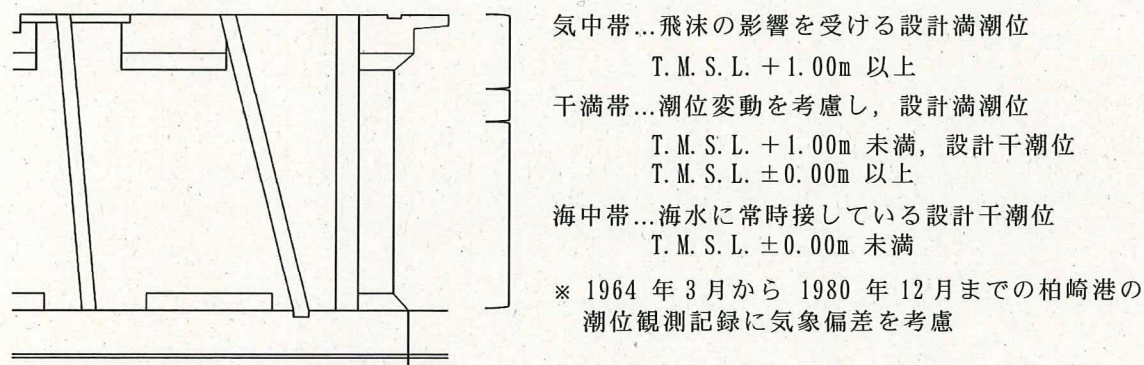
図 5 取水構造物の概要
