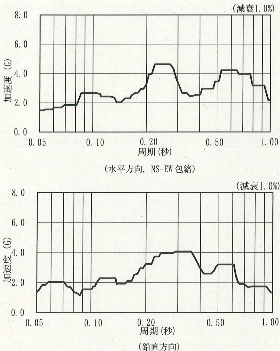
図2 基準地震動 S_s の加速度スペクトル比較図（原子炉基礎版上）
