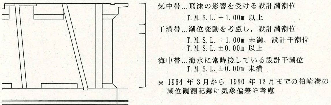
図 7 取水構造物の概要
