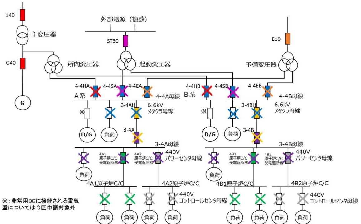
第2-1図 アーク放電発生箇所とアーク放電を遮断する遮断器 (非常用ディーゼル発電機給電時以外)
