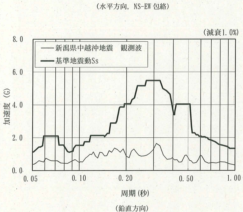
図4 基準地震動 S_s と新潟県中越沖地震観測波の加速度スペクトル比較図 (原子炉基礎版上)
