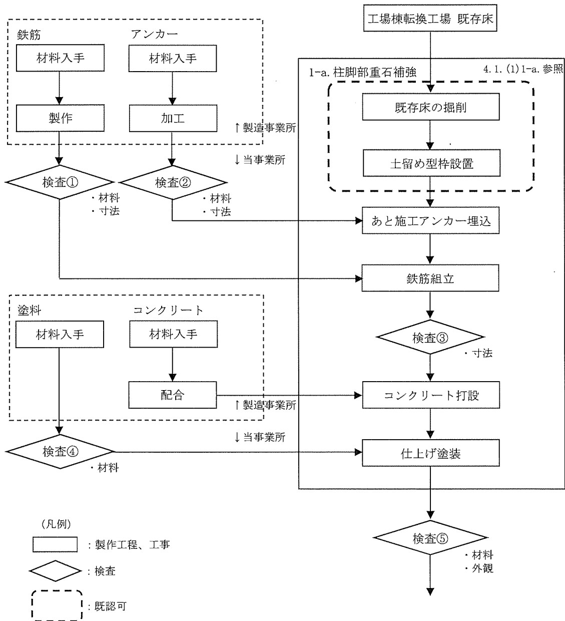
(図イ 1-1 工事の手順フロー図へ)
