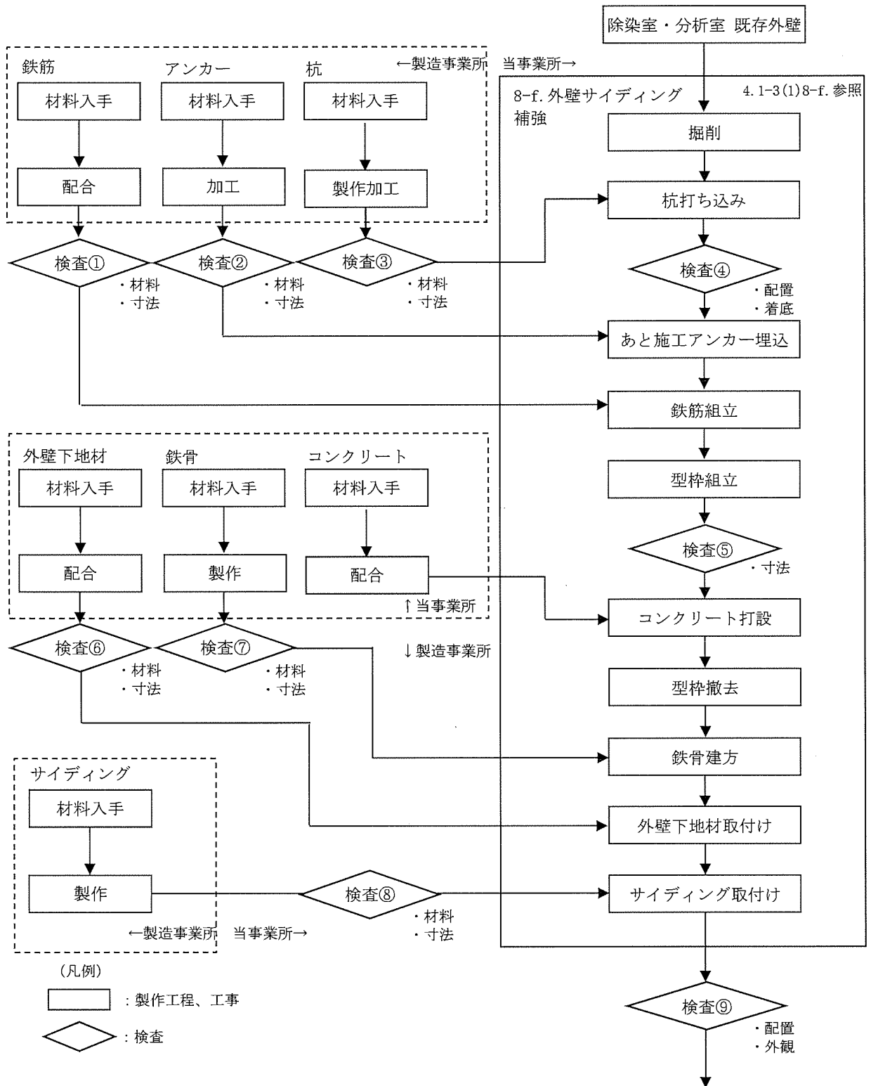
(図ト 1-3 工事の手順フロー図へ)
