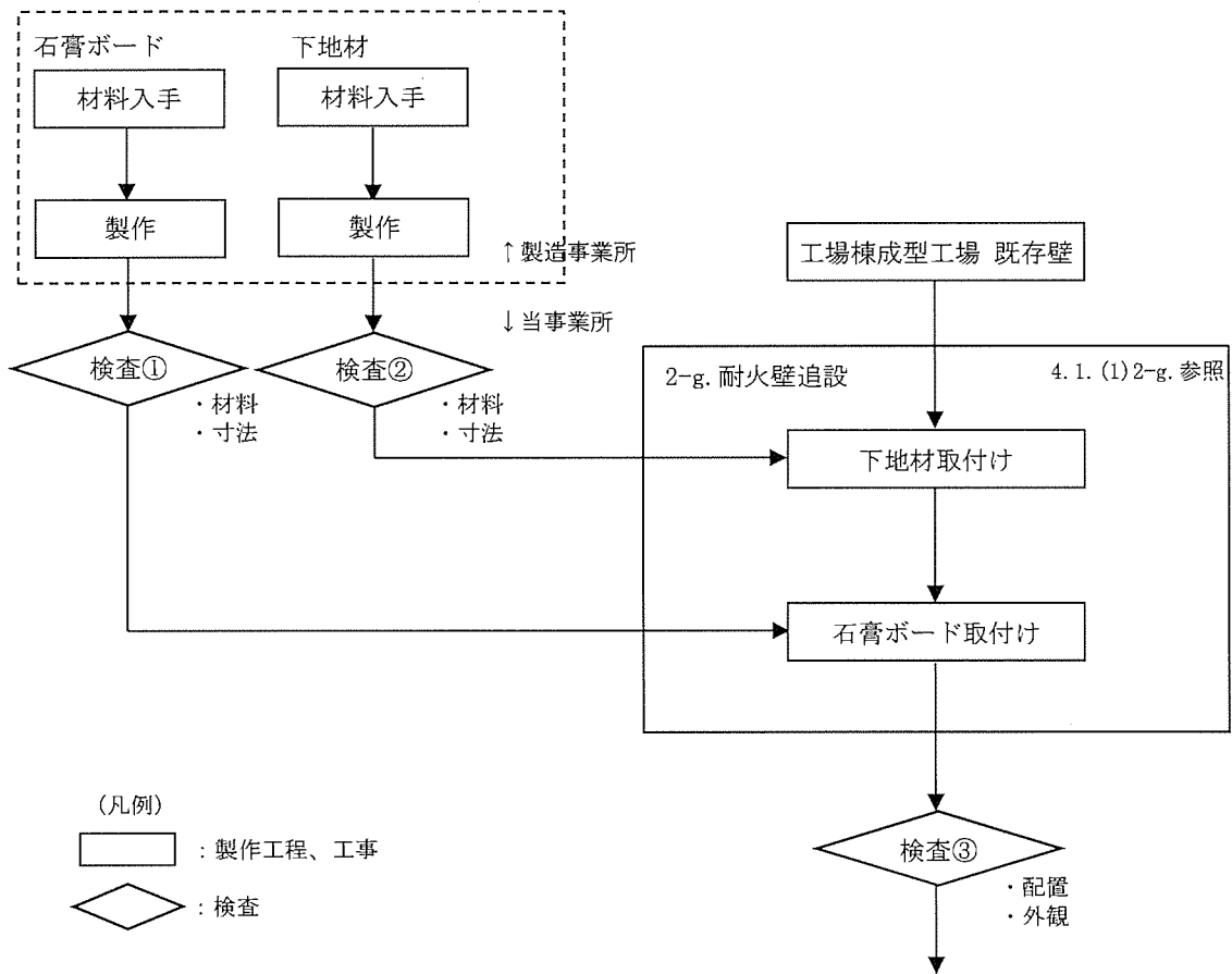
(図ハ 1-1 工事の手順フロー図へ)
