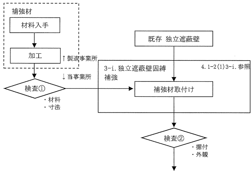
(図ホ 1-1 工事の手順フロー図へ)
