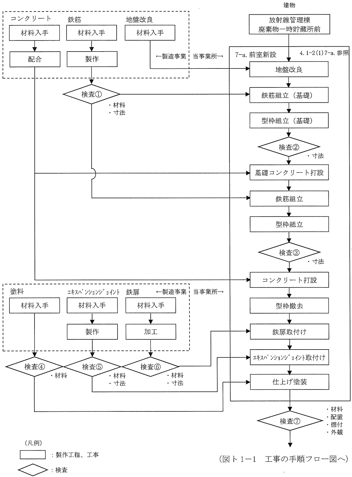
図ト 7-a. 放射線管理棟前室新設の手順フロー図
