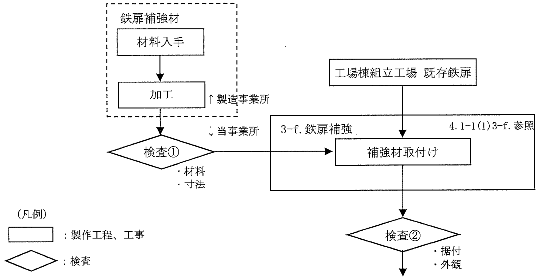
(図ホ 1-1 工事の手順フロー図へ)
