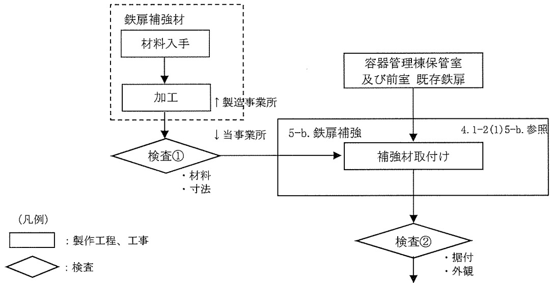
(図へ1-2 工事の手順フロー図へ)
