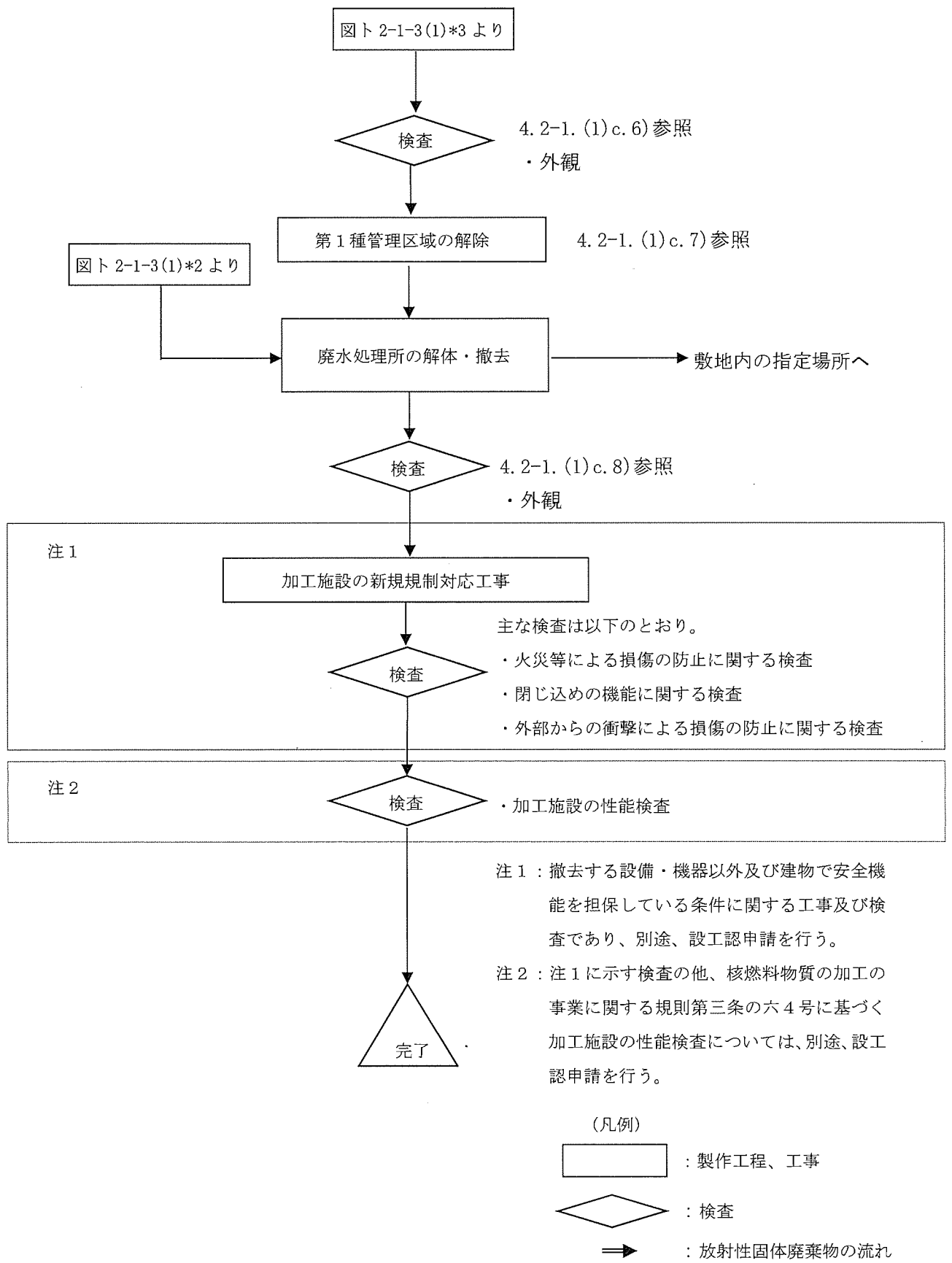
図ト 2-1-3(2) 工事の手順フロー図 (廃水処理所 (廃液処理設備(2))の撤去工事)
