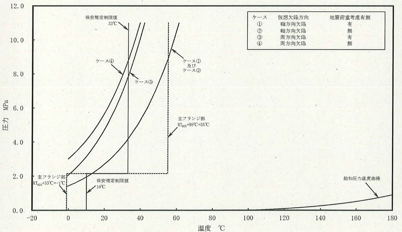
図4 原子炉压力容器の圧力-温度制限図（平成30年3月31日時点） （炉心領域円筒筒、炉心臨界時）
