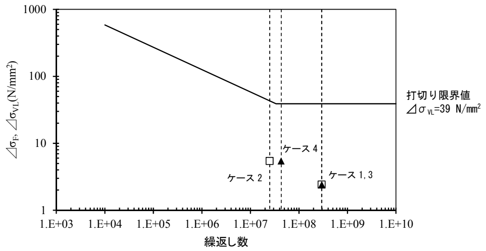
図-別紙 2-1 垂直応力範囲の繰返しによる疲労設計曲線（鉄塔（支柱材））
