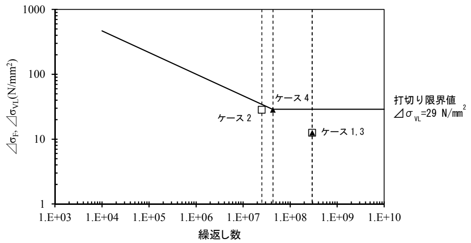
図-別紙 2-2 垂直応力範囲の繰返しによる疲労設計曲線（筒身）
