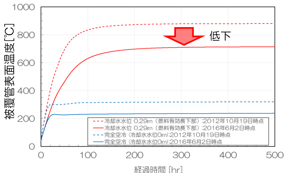
図 3号機使用済燃料プール冷却水喪失時評価
