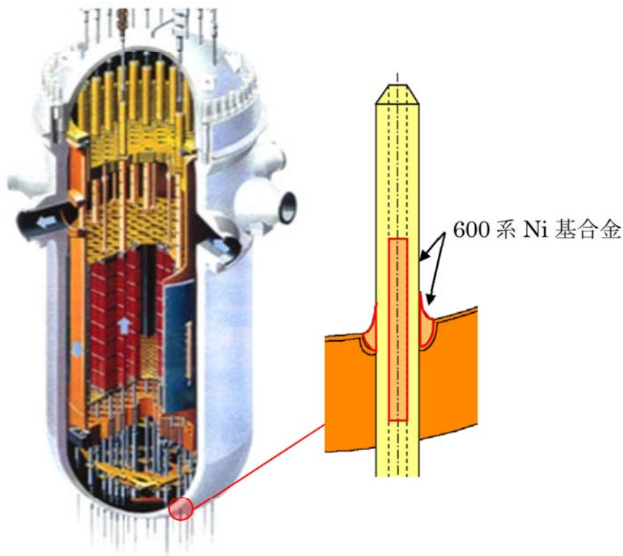
図 3.3.1.2 試験対象 (BMI)
