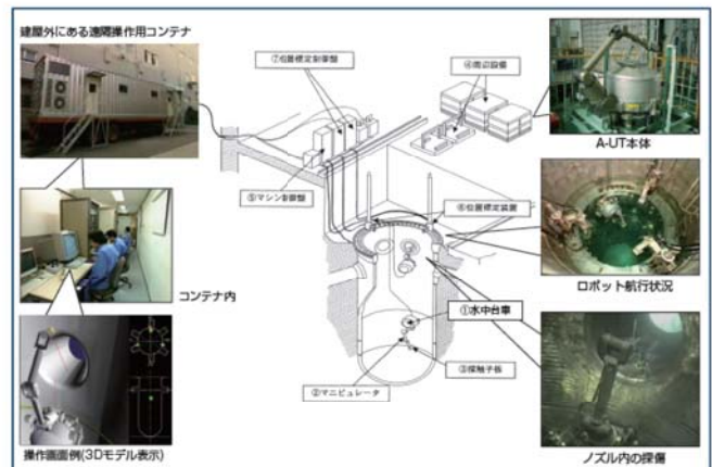
図 3.1.2.2 原子炉容器超音波探傷試験装置
