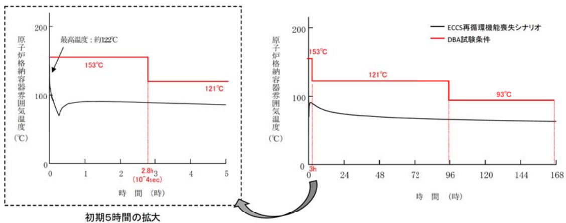
CV内温度推移
