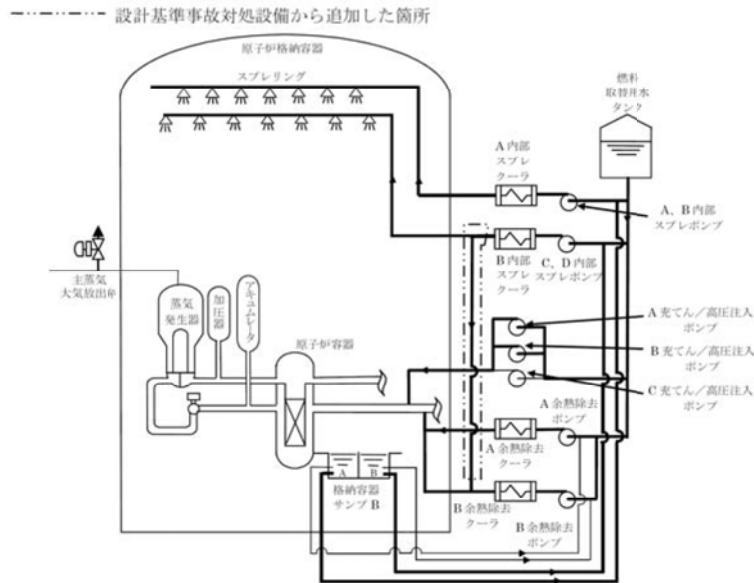
概略系統図
