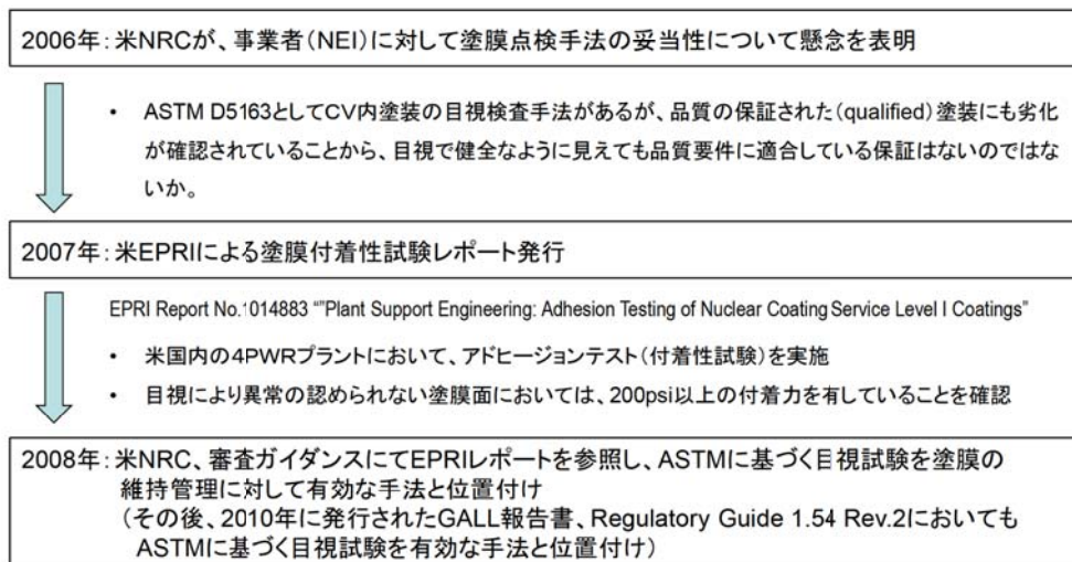
図 米国におけるCV塗装点検に係る議論経緯
