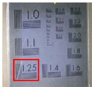
グレーカード（18%中性灰色カード） の幅0.8mmの黒線部（1.25=1/0.8） 識別を確認しながら点検を実施
