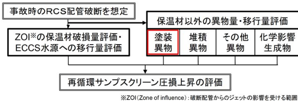
図 事故時の格納容器再循環サンプスクリーン性能評価概要
