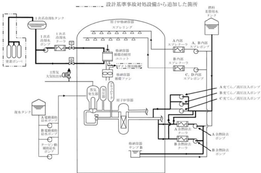
概略系統図
