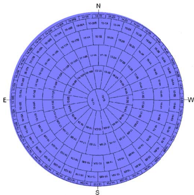
図 3. 8 高浜 1 号炉 半球部内面
