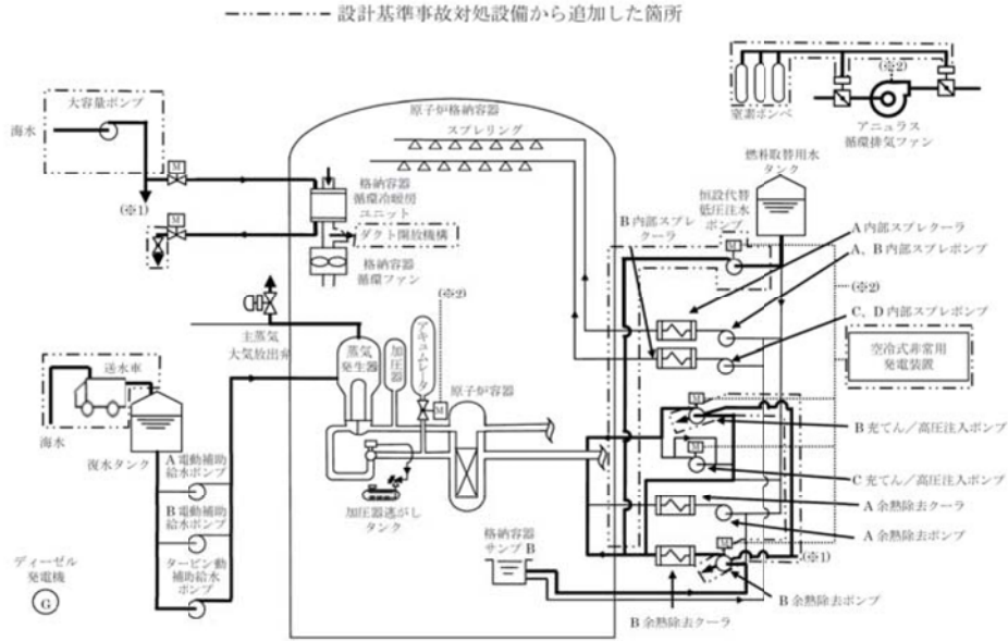
概略系統図
