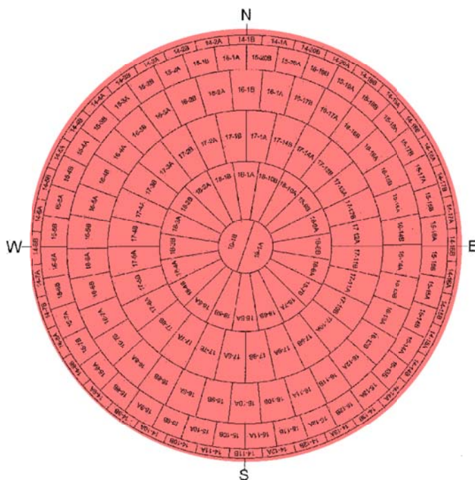
図 3. 9 高浜 1 号炉 半球部外面
