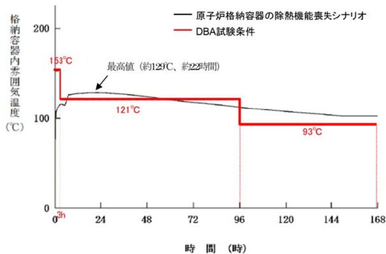
図 「原子炉格納容器の除熱機能喪失」シナリオの CV 内温度推移
