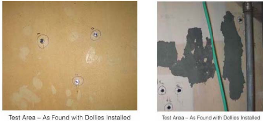
図 健全な塗膜（左）及び劣化箇所付近の塗膜（右）に対する試験片貼り付けの様子 (Waterford Unit3)
