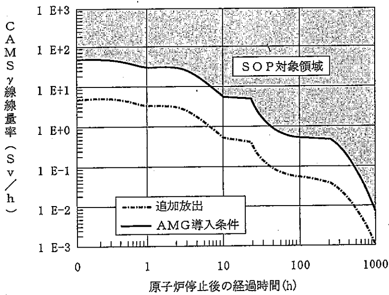
(2) サプレッションチェンバー領域のγ線線量率
