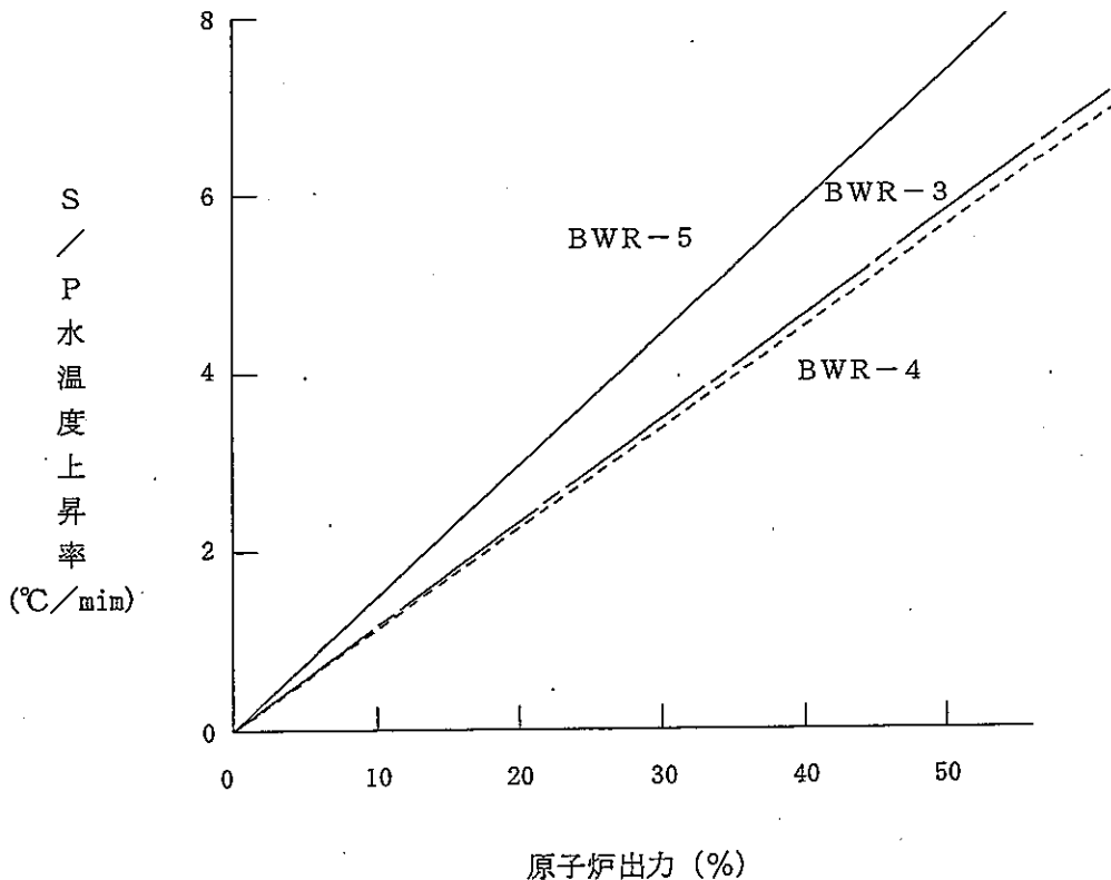
原子炉隔離状態における原子炉出力とS/P水温度上昇率の関係
