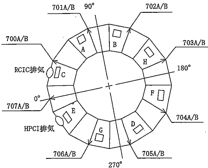
参考4 図1 1F-3 各SRV吹出し位置及び TE 700A/B~707A/B設置場所
