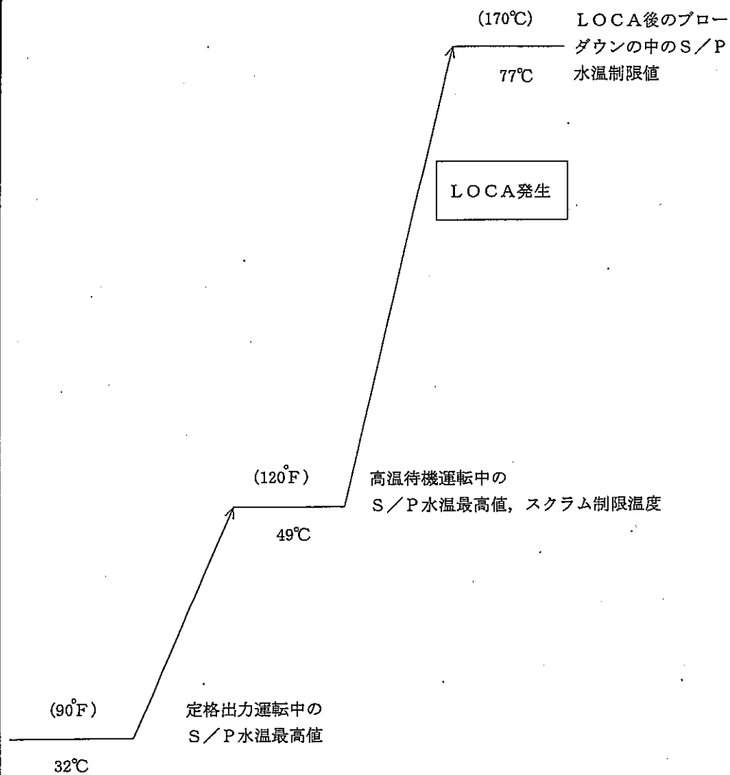
参考3 図1 S/P水温度制限条件概要図
