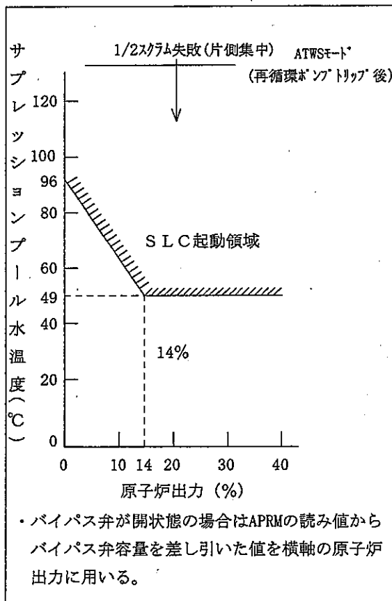
制限図 図C-1 原子炉出力-S/P水温度相関曲線 (BWR 4)
