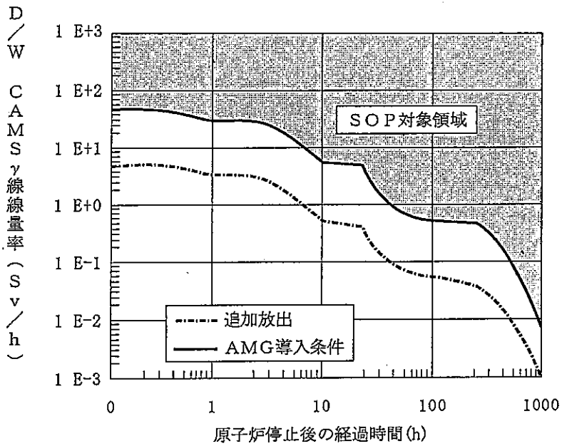
(1) ドライウェル領域のγ線線量率
