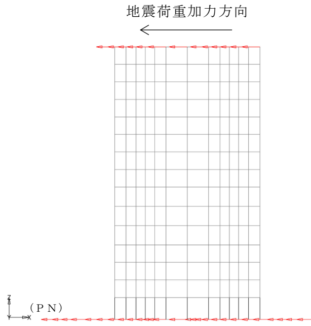
(a) 断面荷重図
