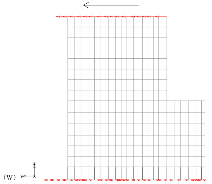
(a) 断面荷重図
