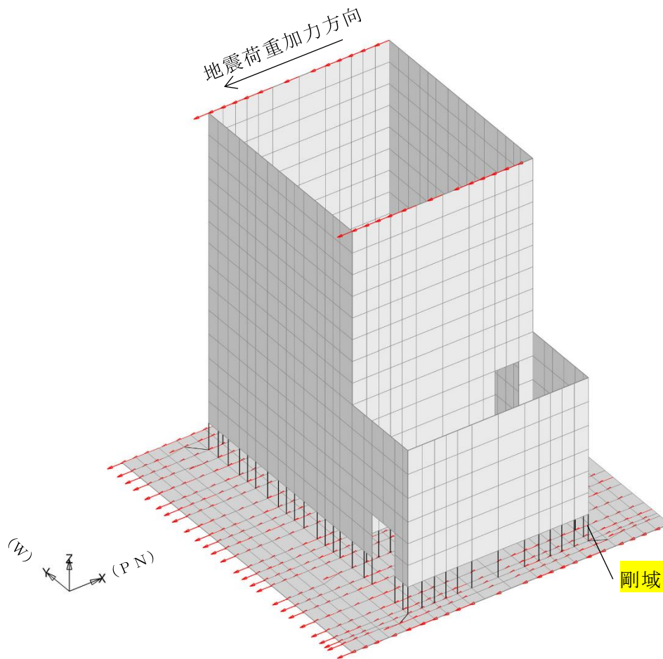
(b) 鳥瞰荷重図
