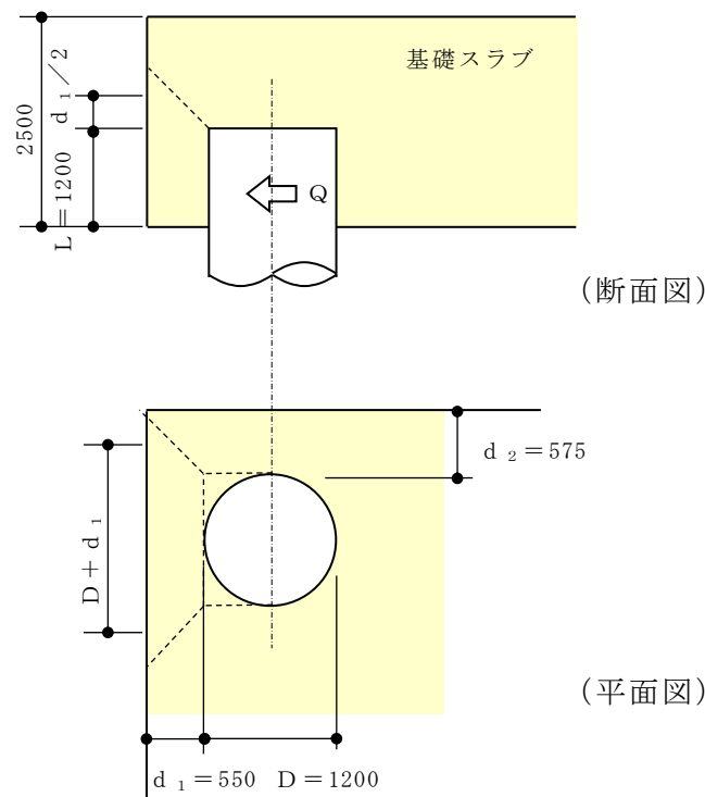
図4-1 杭の水平押抜きせん断の概要 (単位 : mm)
