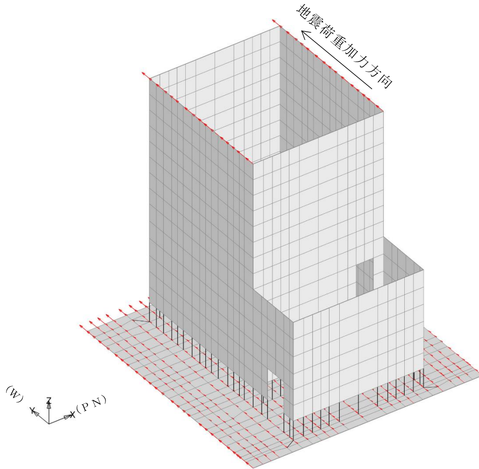
(b) 鳥瞰荷重図
