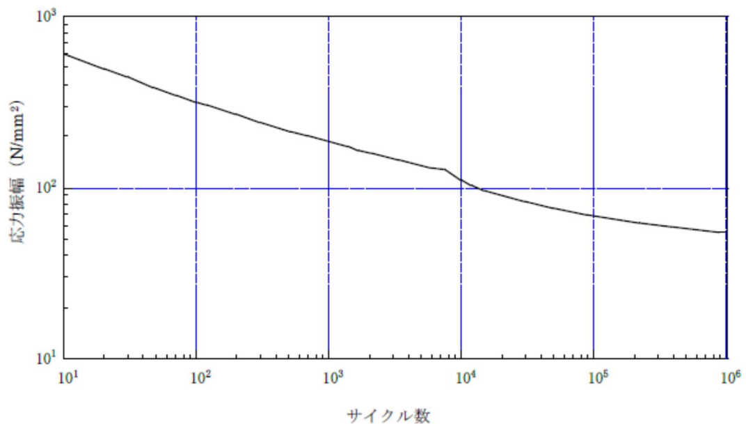
図 1 ジルカロイ設計疲労曲線
