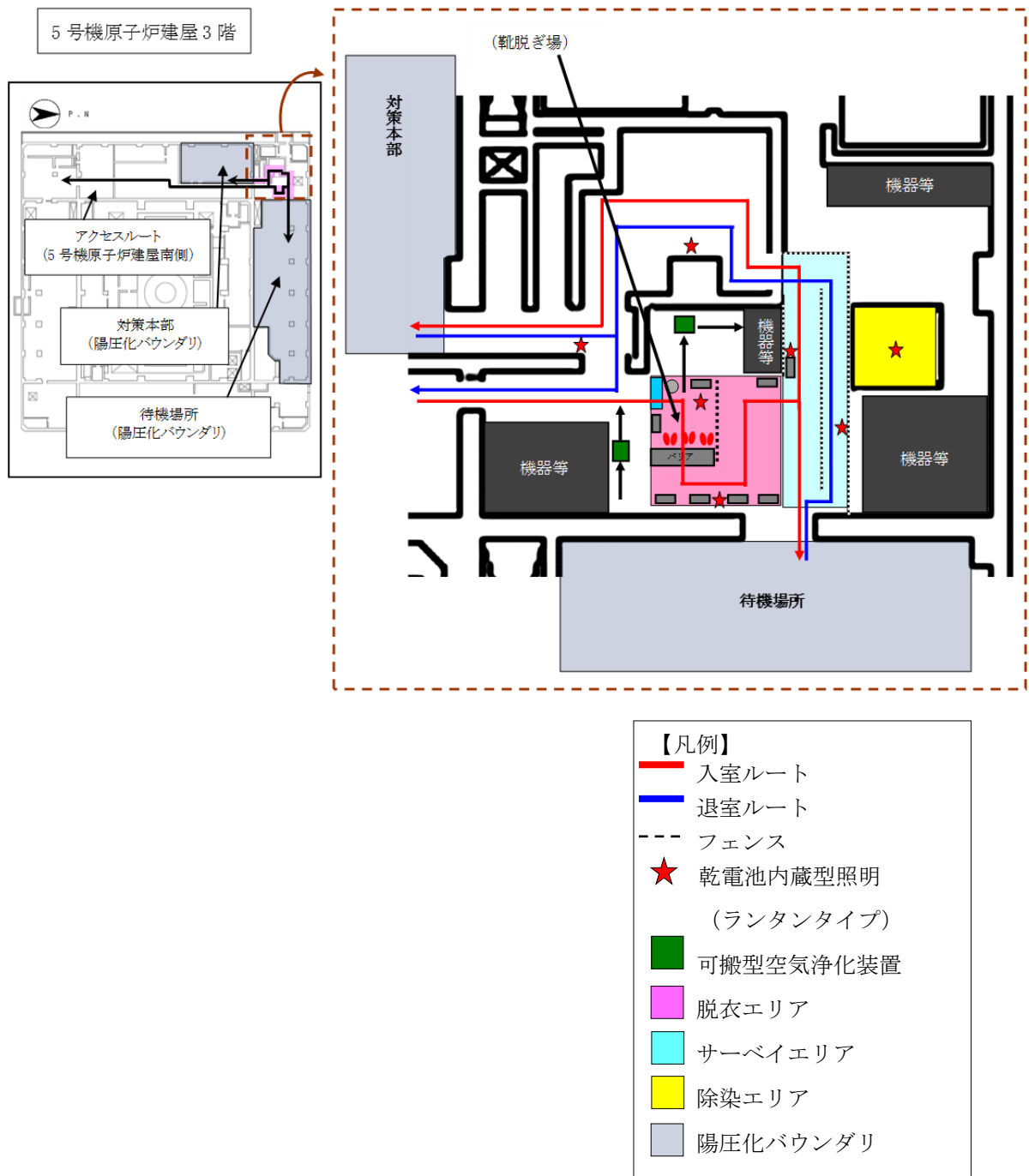
図 3-8 緊急時対策所チェンジングエリアのレイアウト (1/2)
