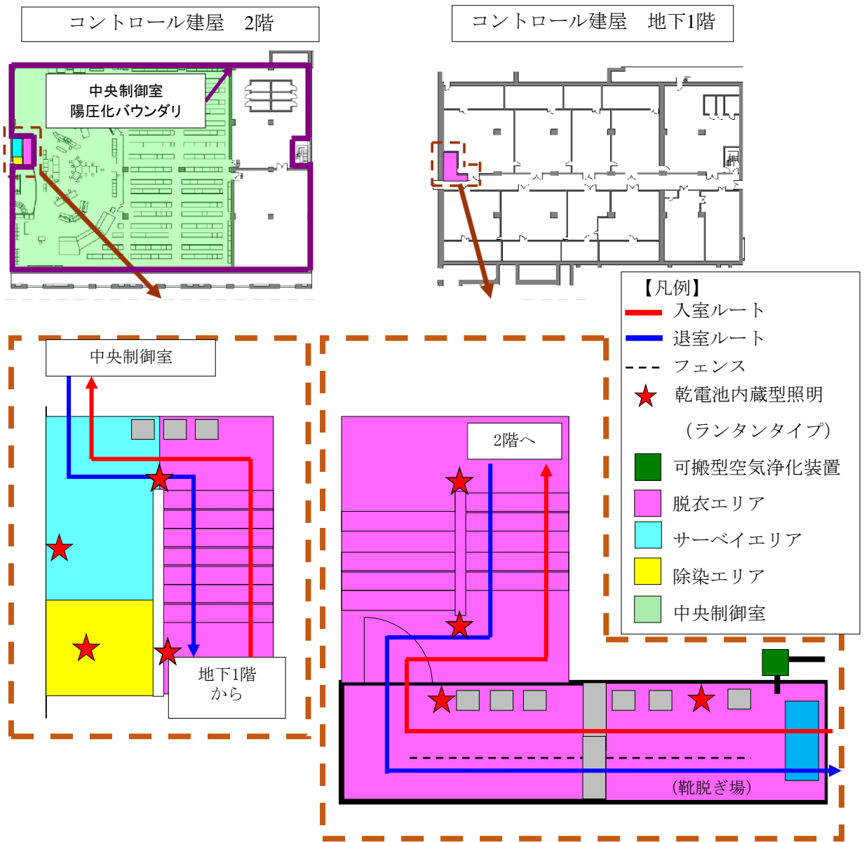
図3-1 中央制御室チェンジングエリア設置場所及び配置
