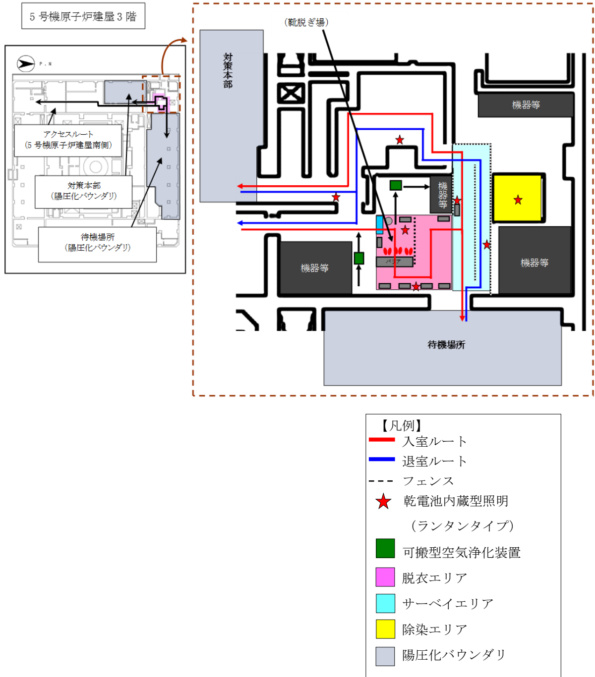
図3-2 緊急時対策所チェンジングエリア設置場所及び配置(1/2)
