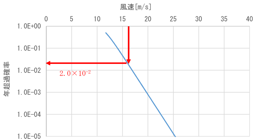
図 1 柏崎市の最大風速ハザード曲線（Gumbel 分布）
