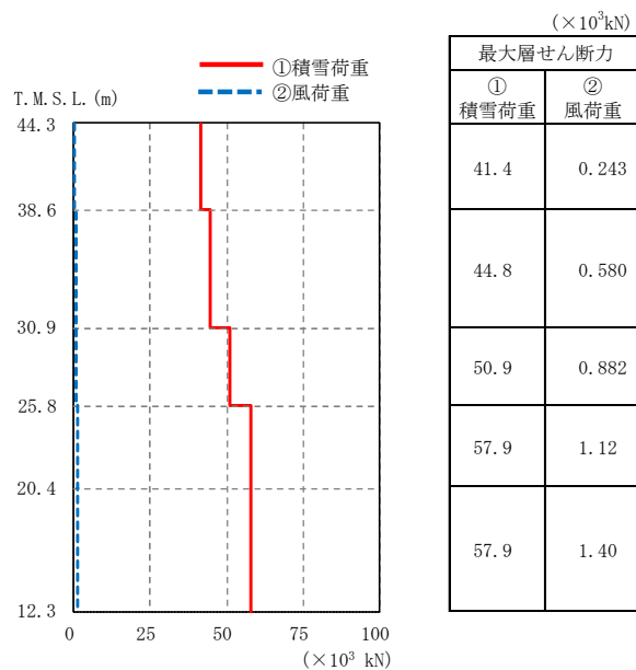
図 3 風荷重と積雪荷重の比較
