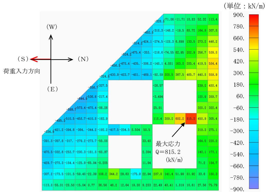
1 方向入力せん断力 (荷重ケース : 1.0(N→S 入力) - 0.4UD 入力)
