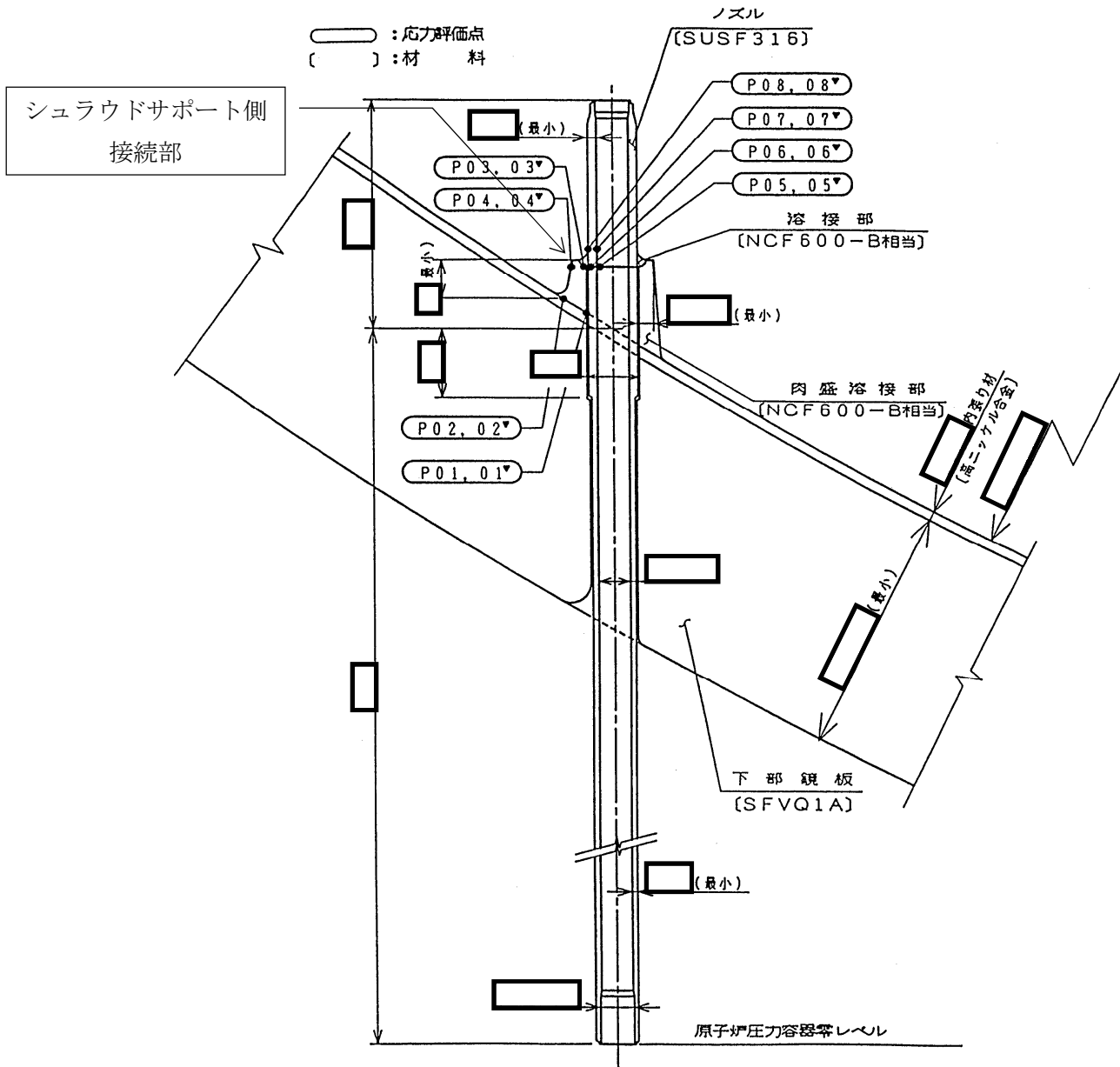
図1 原子炉冷却材再循環ポンプ差圧検出ノズル (N9) 構造図
