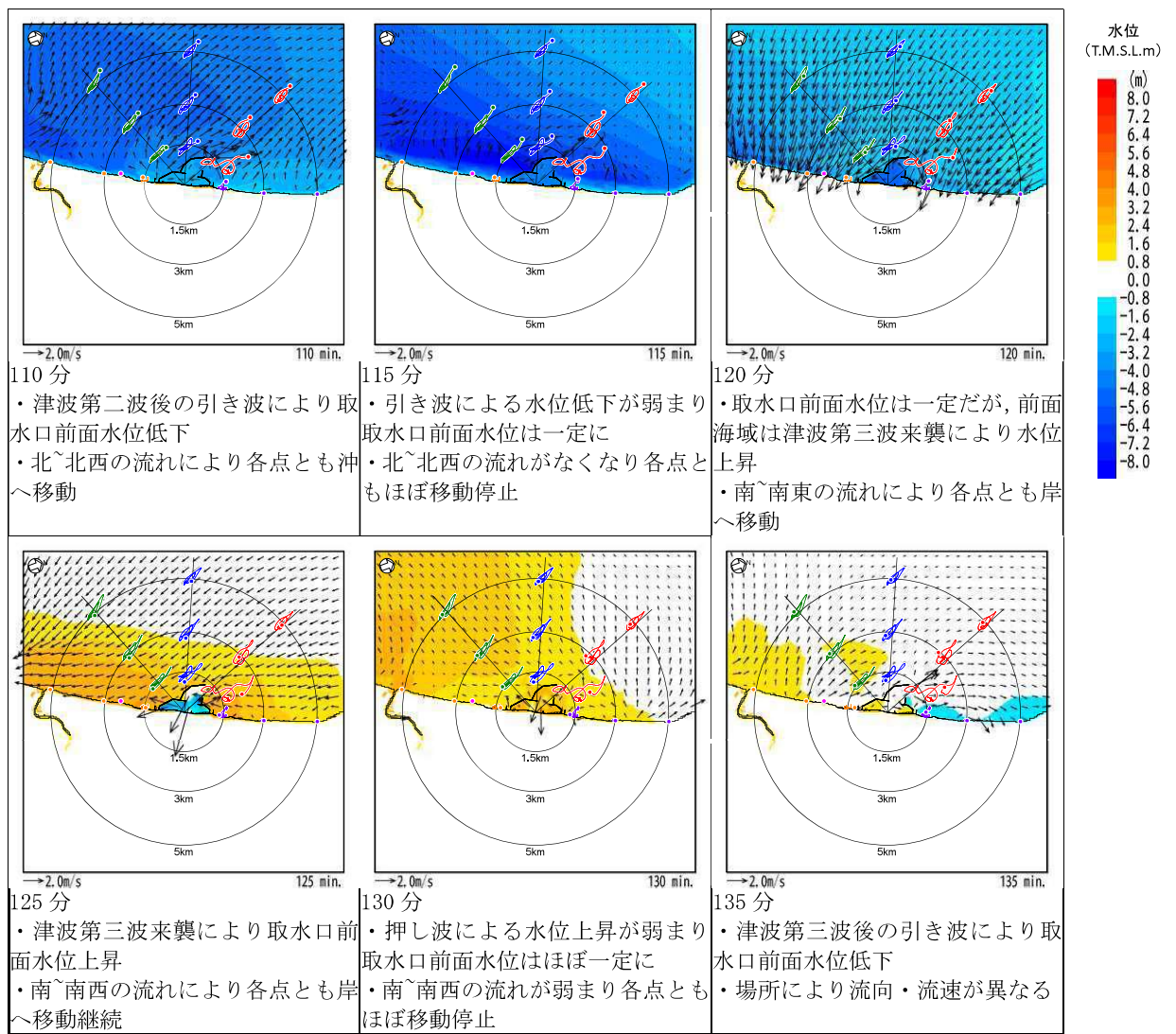
図 4.7-添 2(b)-7(2) 水位・流向・流速を用いた傾向分析結果 (基準津波 2 防波堤 1m 沈下 地震発生後 120 分頃)
