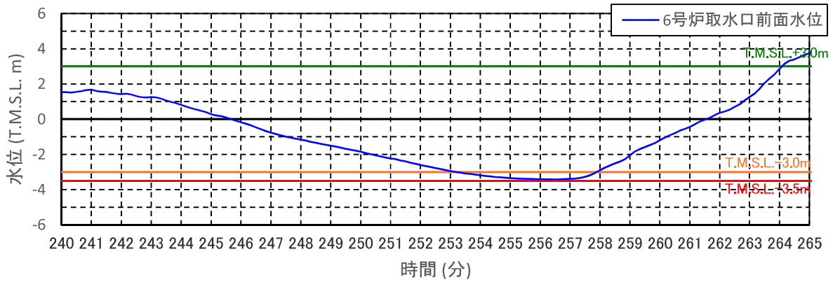
図 4.7-添 3-2(7) 6号機取水口前面水位と護岸部浸水深 (基準津波 2 防波堤健全・護岸部健全: ③)
