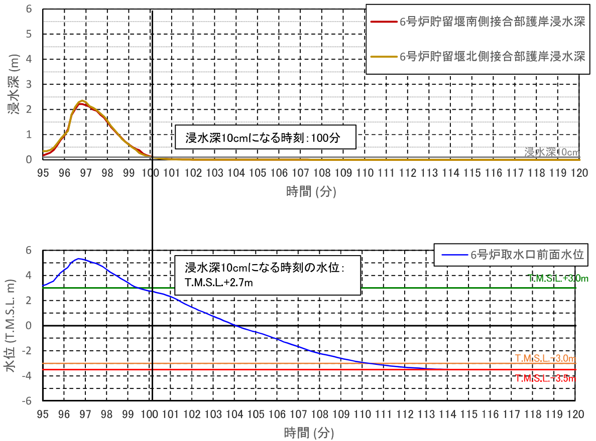
図 4.7-添 3-2(6) 6号機取水口前面水位と護岸部浸水深 (基準津波 2 防波堤健全・護岸部健全: ②)
