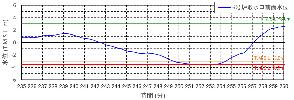
図 4.7-添 3-2(14) 6号機取水口前面水位と護岸部浸水深 (基準津波 2 防波堤なし・護岸部健全: ④)
