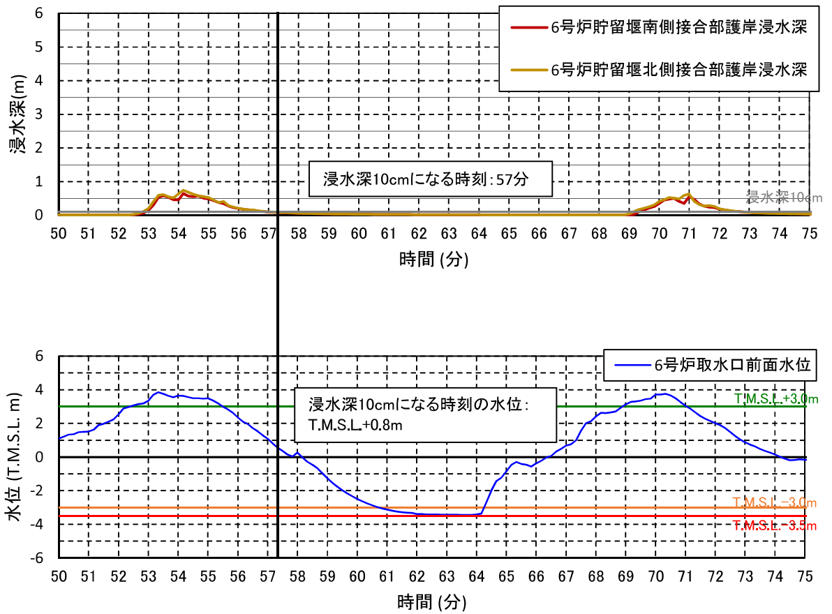
図 4.7-添 3-2(1) 6号機取水口前面水位と護岸部浸水深 (基準津波 1 防波堤なし・護岸部健全: ①)
