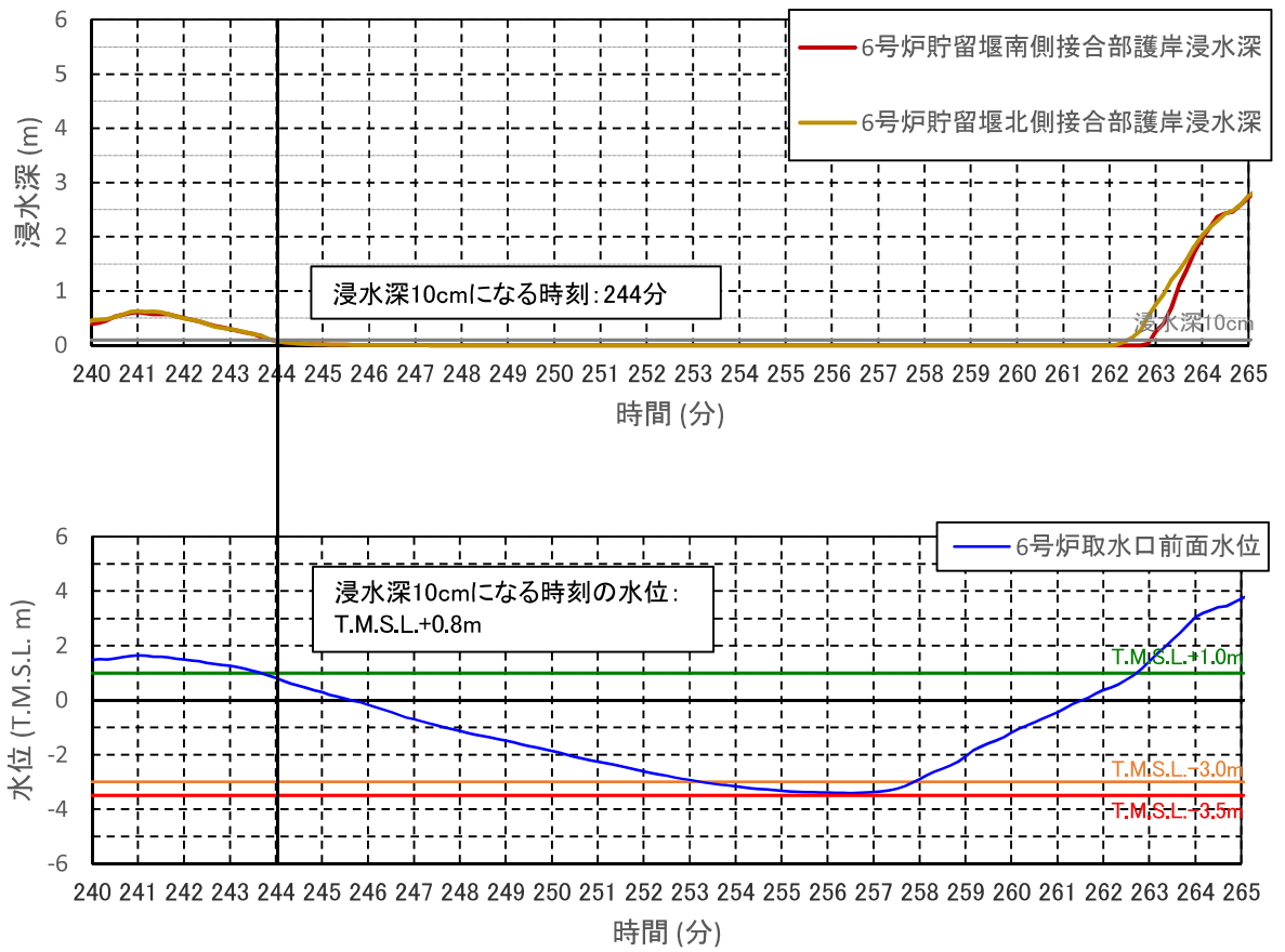
図 4.7-添 3-2(10) 6号機取水口前面水位と護岸部浸水深 (基準津波 2 防波堤健全・護岸部 2m 沈下: ③)
