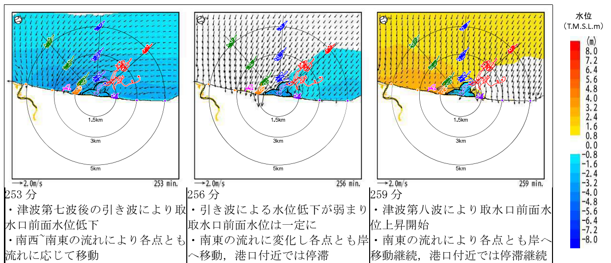
図 4.7-添 2(b)-6(3) 水位・流向・流速を用いた傾向分析結果 (基準津波 2 防波堤健全 地震発生後 255 分頃)
