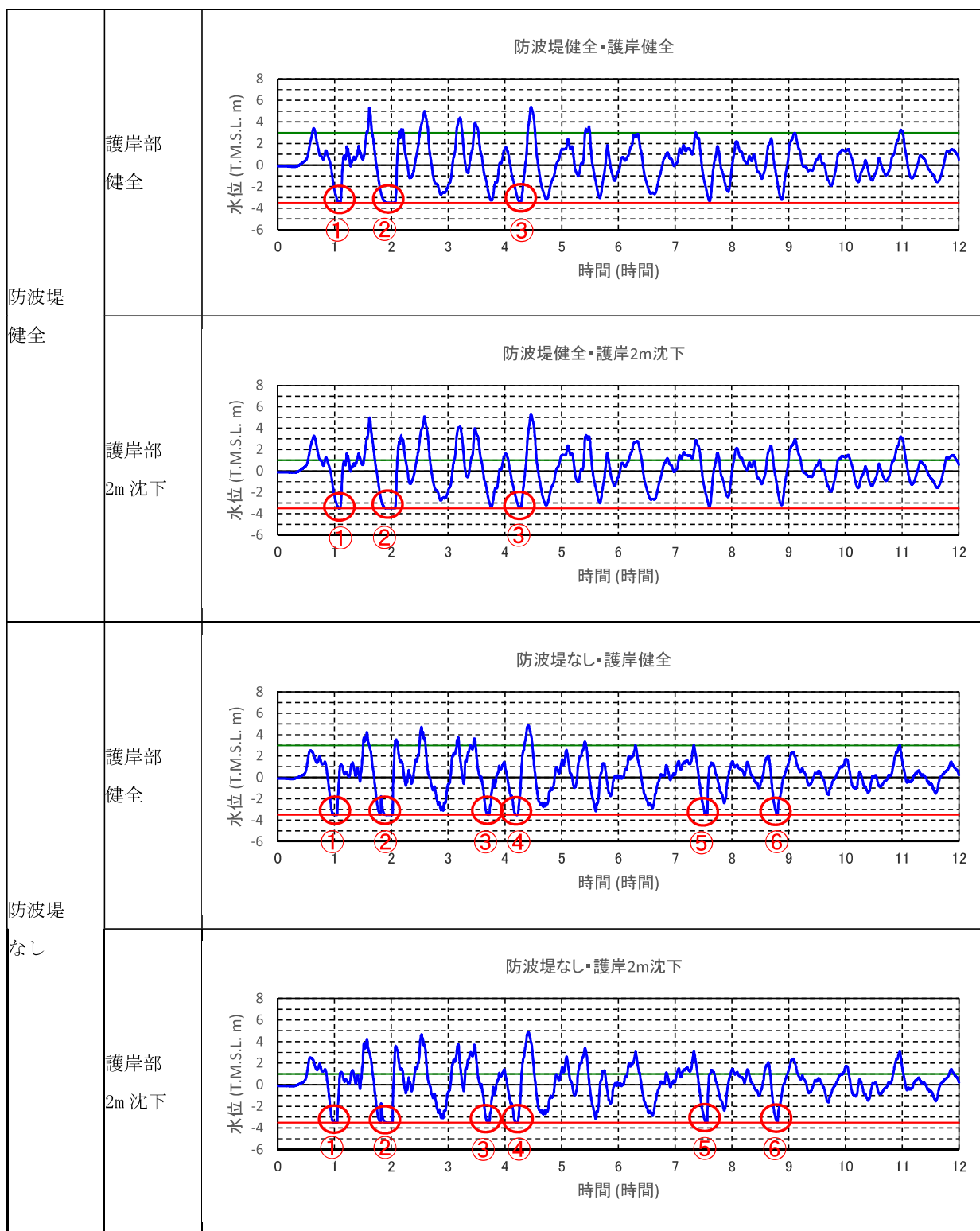
図 4.7-添 3-1(2) 6号機取水口前面水位の時刻歴波形 (基準津波 2)
