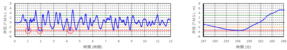
6号機取水口前面水位
