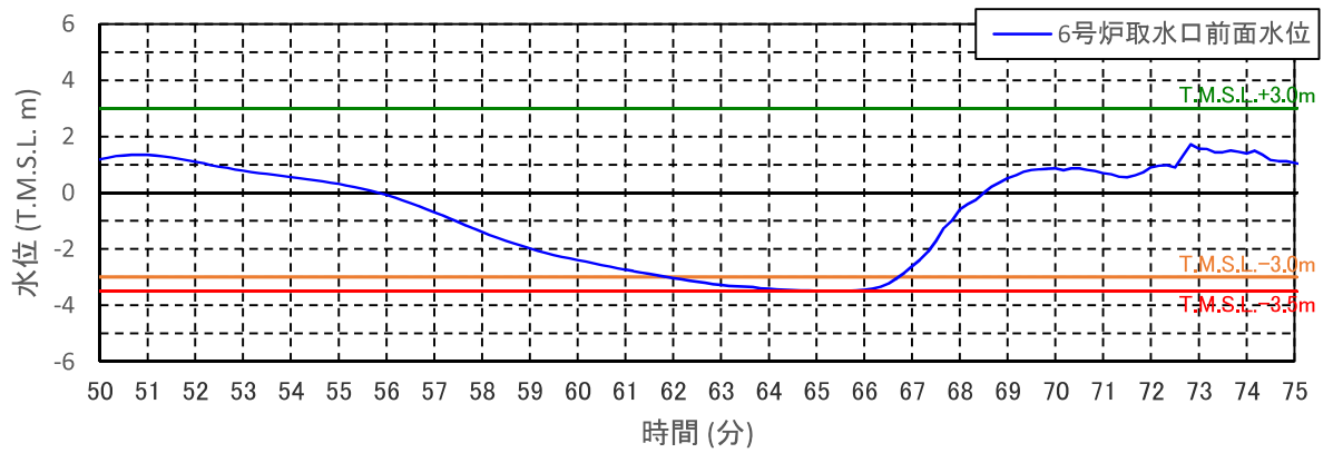
図 4.7-添 3-2(5) 6号機取水口前面水位と護岸部浸水深 (基準津波 2 防波堤健全・護岸部健全: ①)
