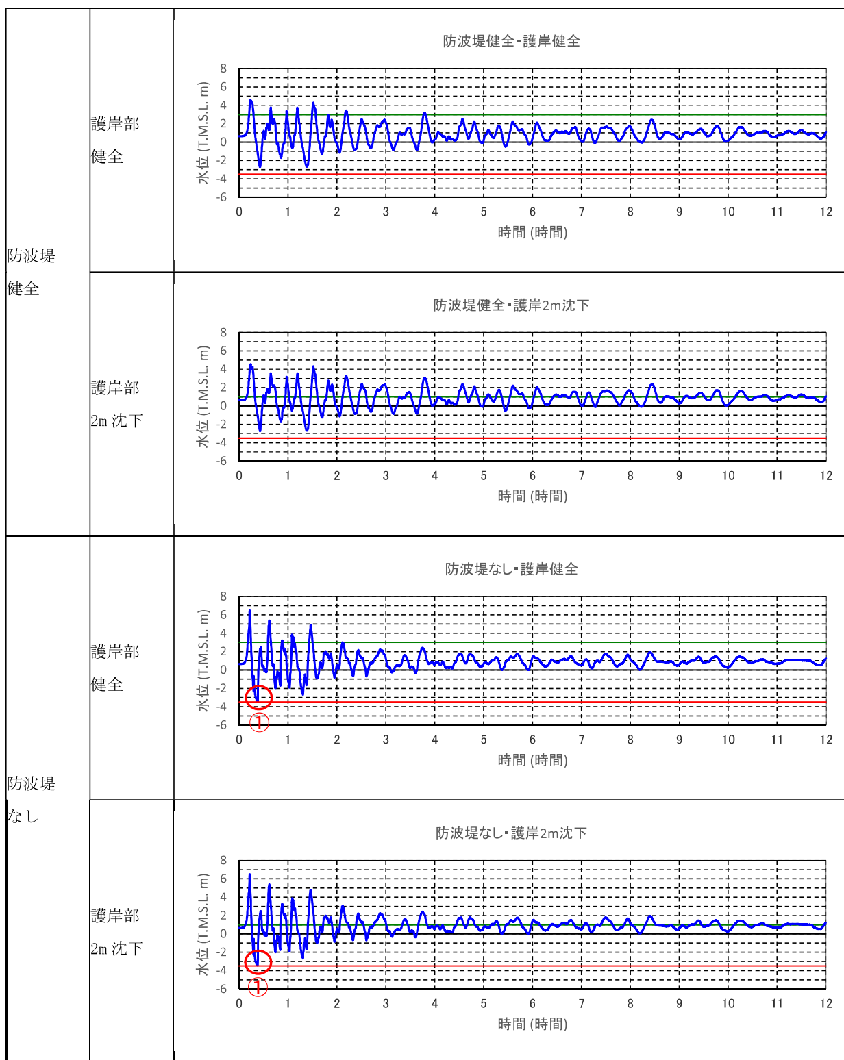
図 4.7-添 3-1(3) 6号機取水口前面水位の時刻歴波形 (基準津波 3)
