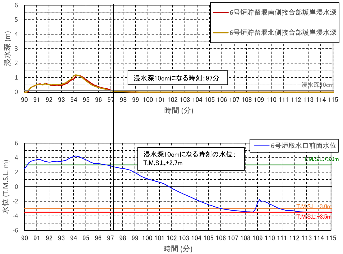
図 4.7-添 3-2(12) 6号機取水口前面水位と護岸部浸水深 (基準津波 2 防波堤なし・護岸部健全: ②)
