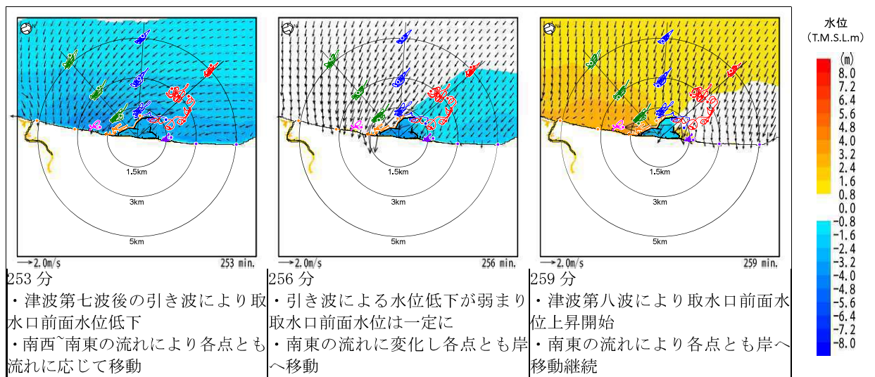
図 4.7-添 2(b)-7(3) 水位・流向・流速を用いた傾向分析結果 (基準津波 2 防波堤 1m 沈下 地震発生後 255 分頃)
