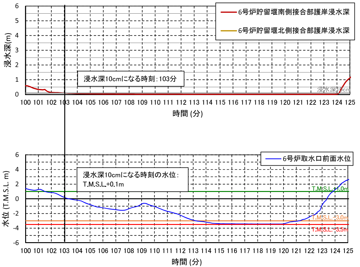
図 4.7-添 3-2(4) 6号機取水口前面水位と護岸部浸水深 (基準津波 1 防波堤なし・護岸部 2m 沈下: ②)
