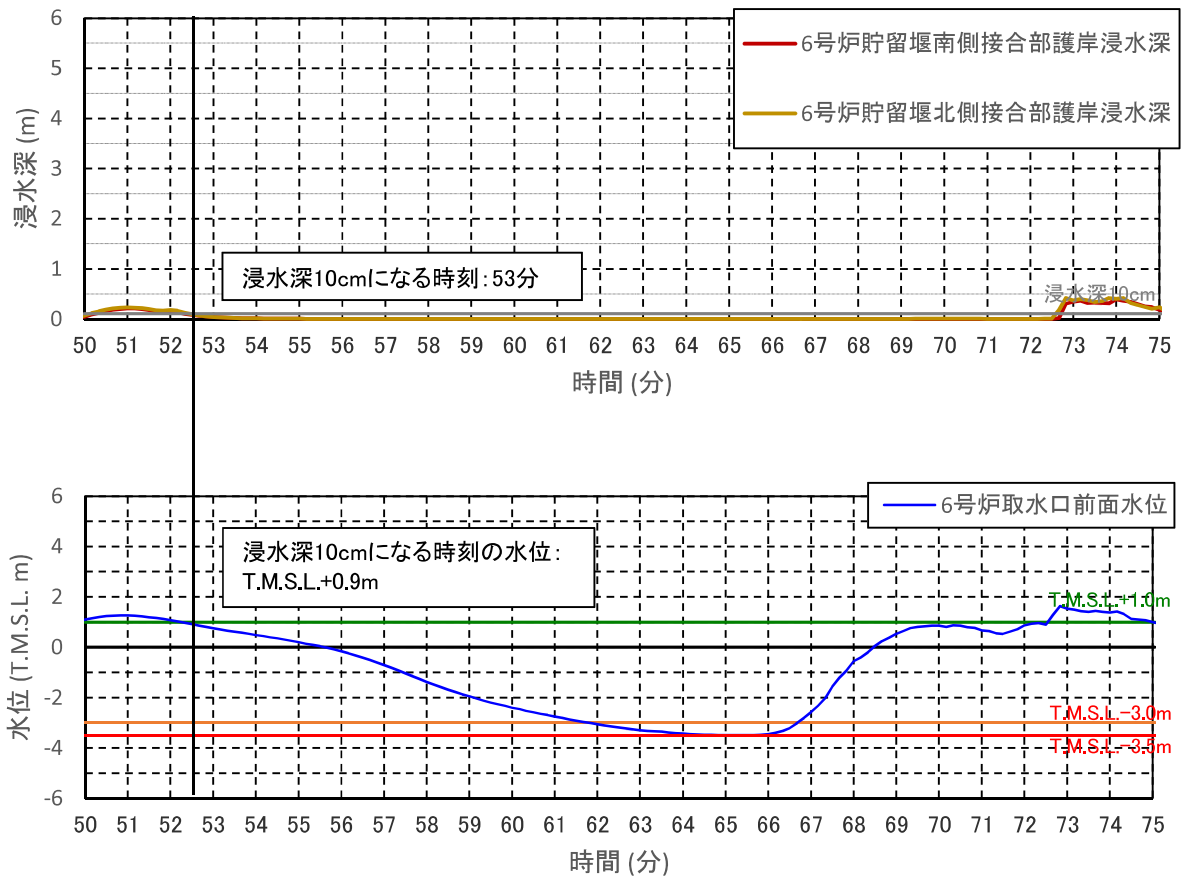
図 4.7-添 3-2(8) 6号機取水口前面水位と護岸部浸水深 (基準津波 2 防波堤健全・護岸部 2m 沈下: ①)
