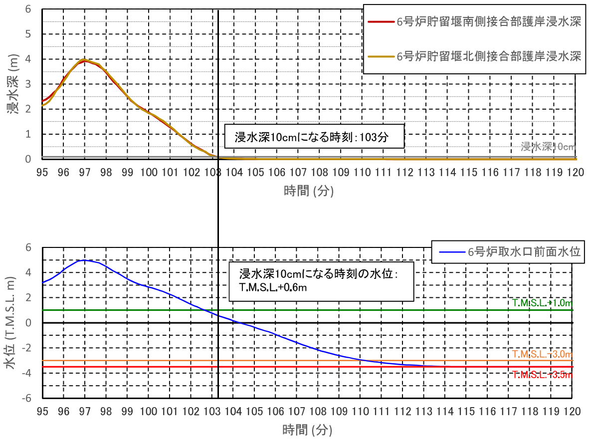
図 4.7-添 3-2(9) 6号機取水口前面水位と護岸部浸水深 (基準津波 2 防波堤健全・護岸部 2m 沈下: ②)
