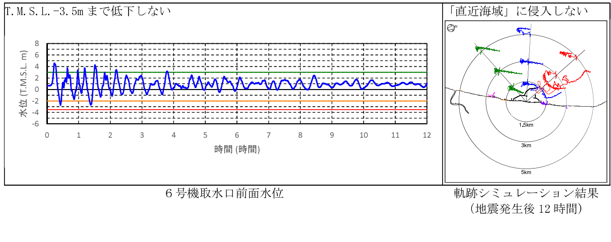
図 4.7-添 2(b)-10(1) 水位・流向・流速を用いた傾向分析結果（基準津波 3 防波堤健全）
