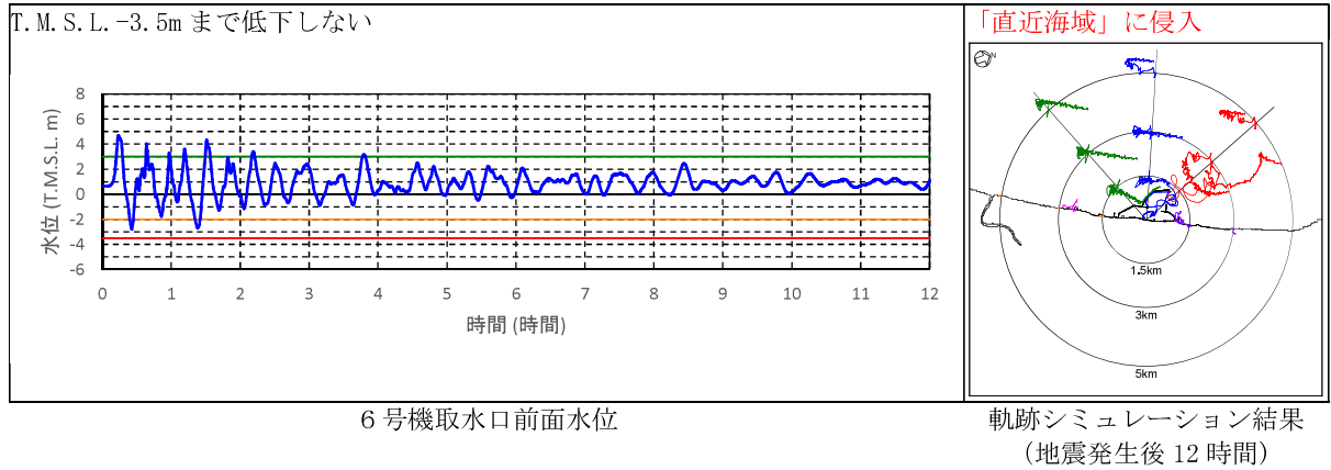
図 4.7-添 2(b)-11(1) 水位・流向・流速を用いた傾向分析結果 (基準津波 3 防波堤 1m 沈下)
