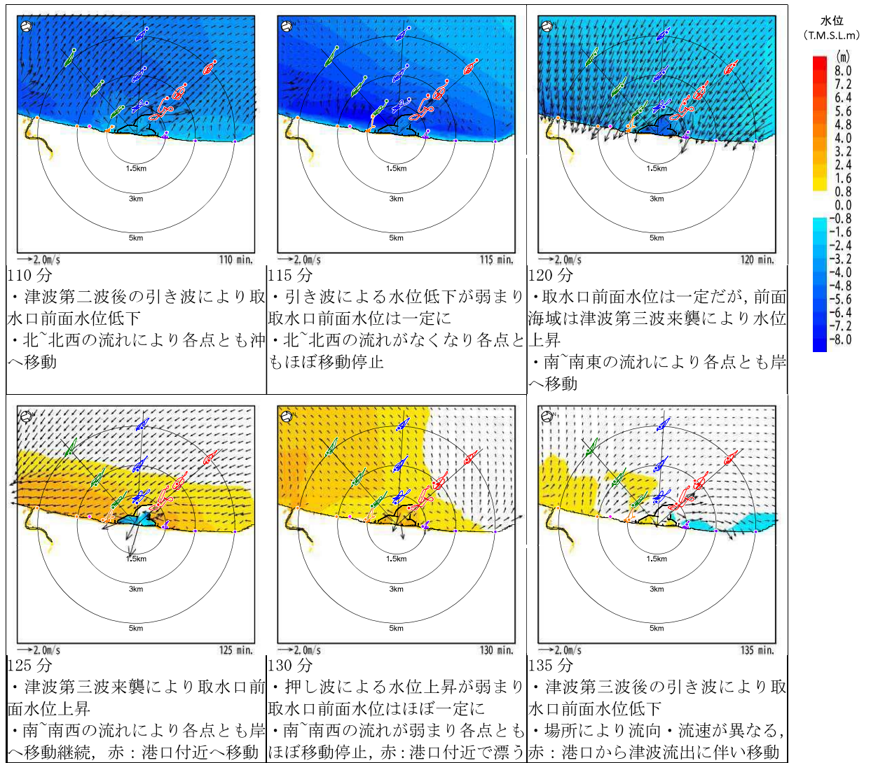
図 4.7-添 2(b)-6(2) 水位・流向・流速を用いた傾向分析結果 (基準津波 2 防波堤健全 地震発生後 120 分頃)
