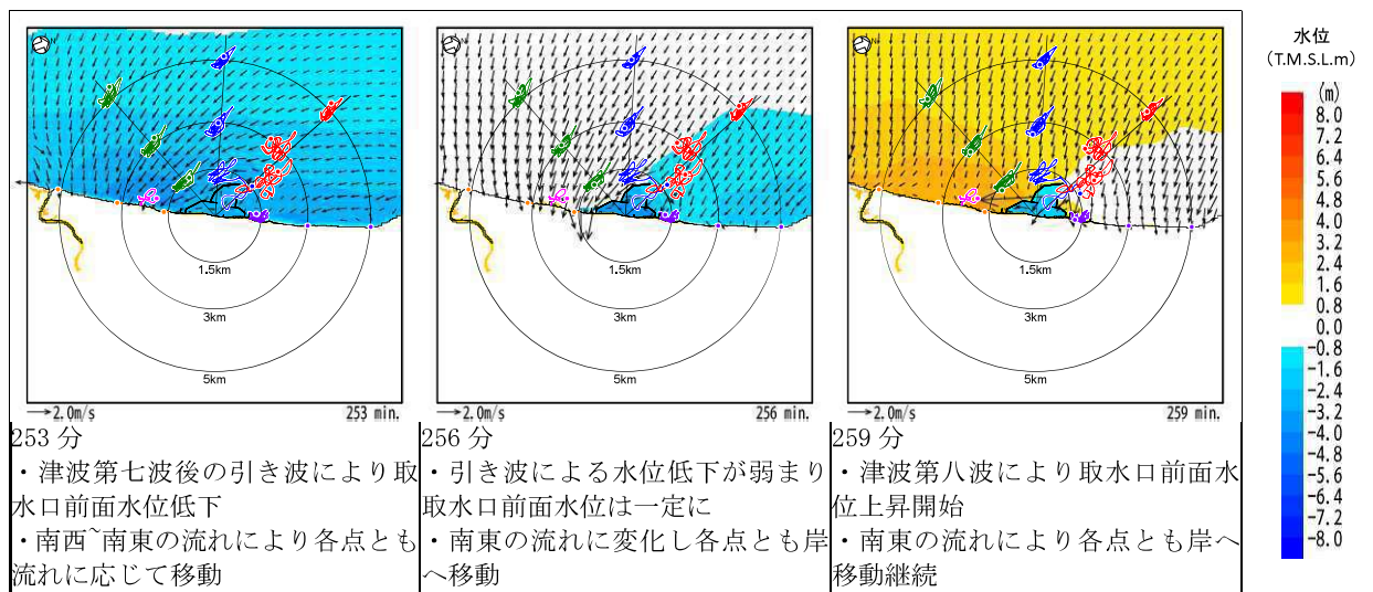
図 4.7-添 2(b)-8(3) 水位・流向・流速を用いた傾向分析結果 (基準津波 2 防波堤 2m 沈下 地震発生後 255 分頃)
