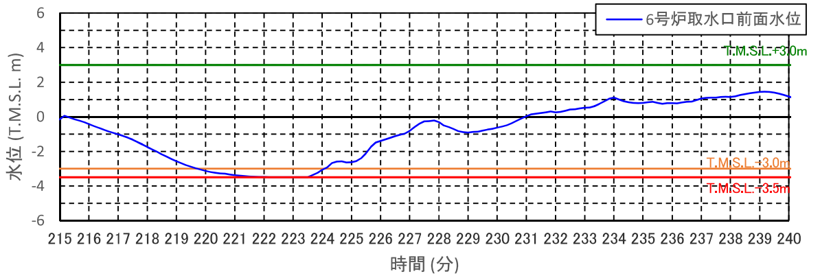
図 4.7-添 3-2(13) 6号機取水口前面水位と護岸部浸水深 (基準津波 2 防波堤なし・護岸部健全: ③)
