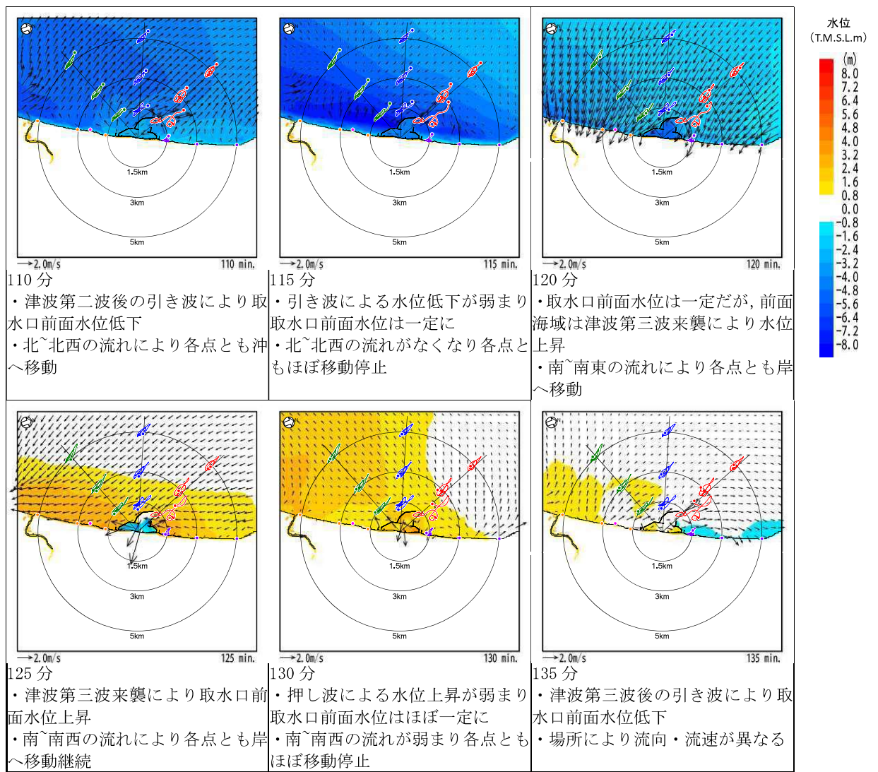
図 4.7-添 2(b)-8(2) 水位・流向・流速を用いた傾向分析結果 (基準津波 2 防波堤 2m 沈下 地震発生後 120 分頃)
