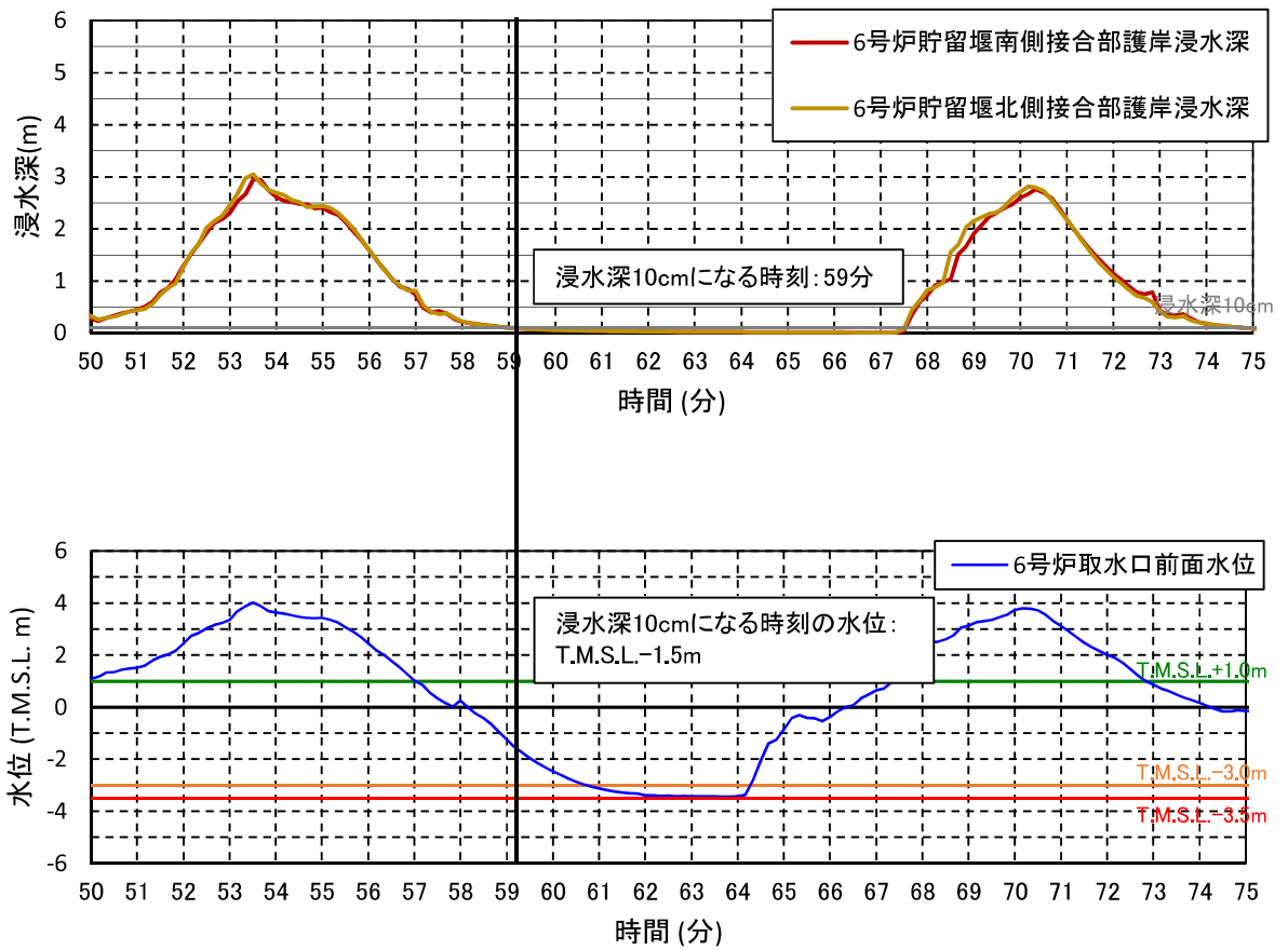
図 4.7-添 3-2(3) 6号機取水口前面水位と護岸部浸水深 (基準津波 1 防波堤なし・護岸部 2m 沈下: ①)
