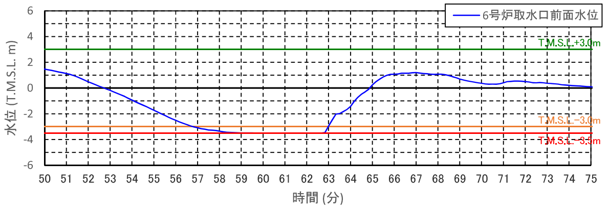
図 4.7-添 3-2(11) 6号機取水口前面水位と護岸部浸水深 (基準津波 2 防波堤なし・護岸部健全: ①)
