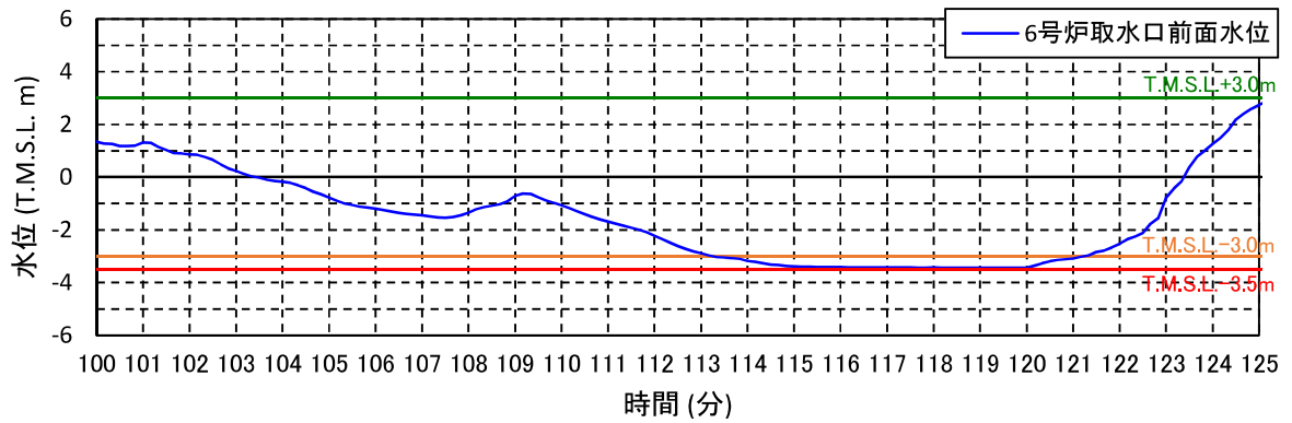
図 4.7-添 3-2(2) 6号機取水口前面水位と護岸部浸水深 (基準津波 1 防波堤なし・護岸部健全: ②)
