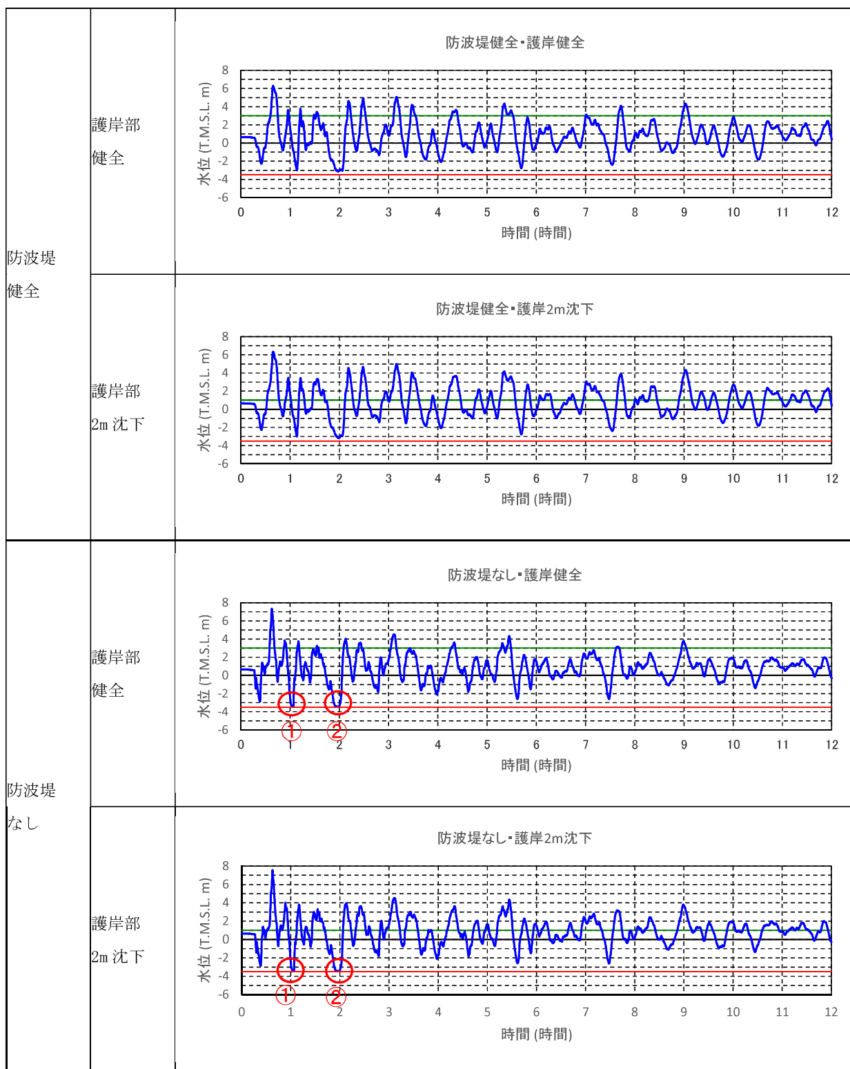
図 4.7-添 3-1(1) 6号機取水口前面水位の時刻歴波形 (基準津波 1)
