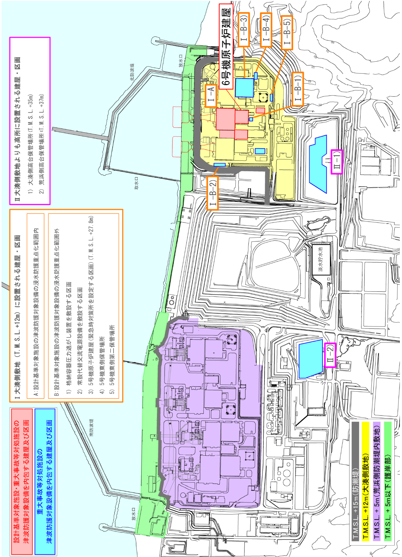
図 2-1 津波防護対象設備を内包する建屋及び区画 (発電所全体)
