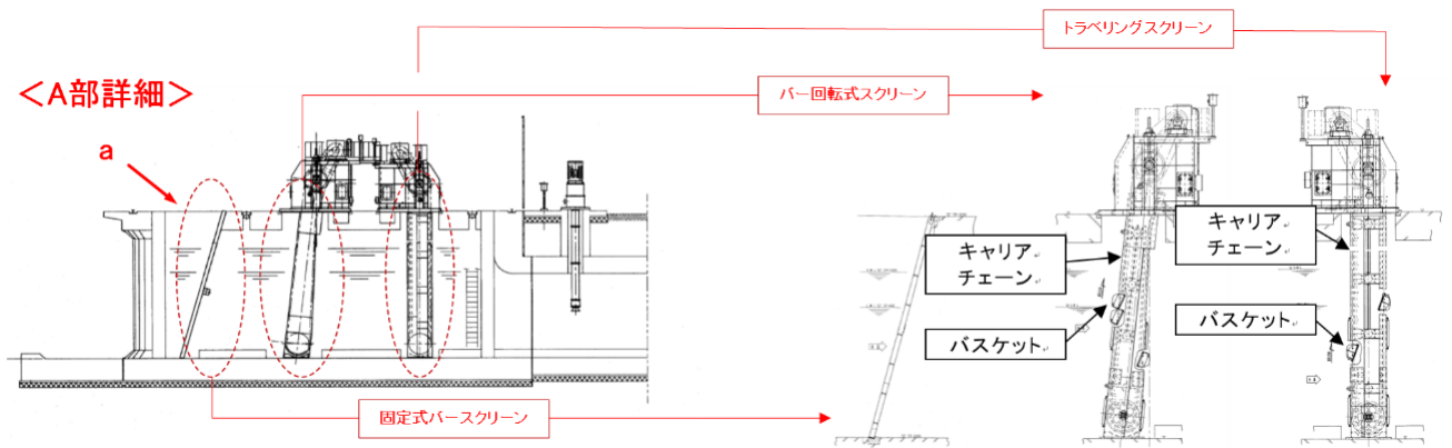
図 3-25 除塵装置の評価対象部位
