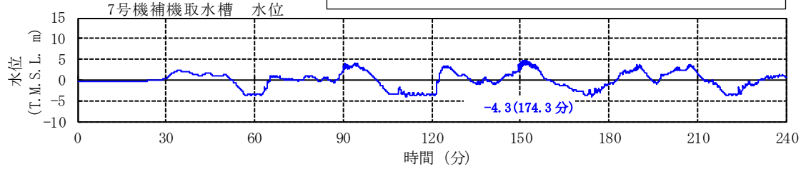
図 4-3(4) 経路からの津波の時刻歴波形
