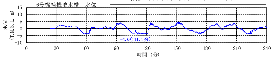
⑬6号機補機取水槽（下降側）
