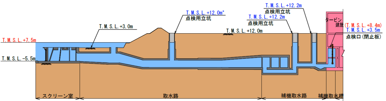
補機冷却海水系 (B-B断面)
