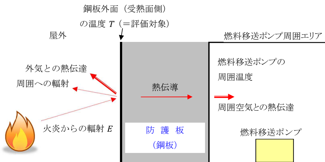
図 2-11 防護板（鋼板）温度評価体系図
