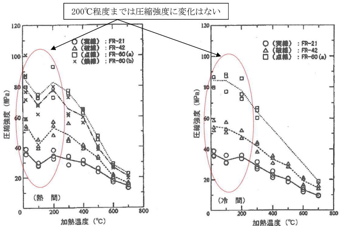
図2-6 コンクリートの強度と温度の関係 *2s
