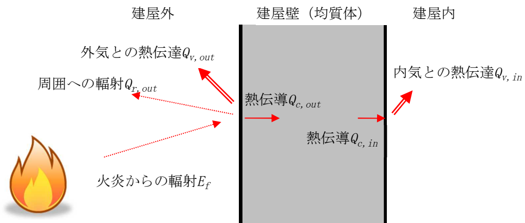
図 2-4 外壁面温度評価概念図
