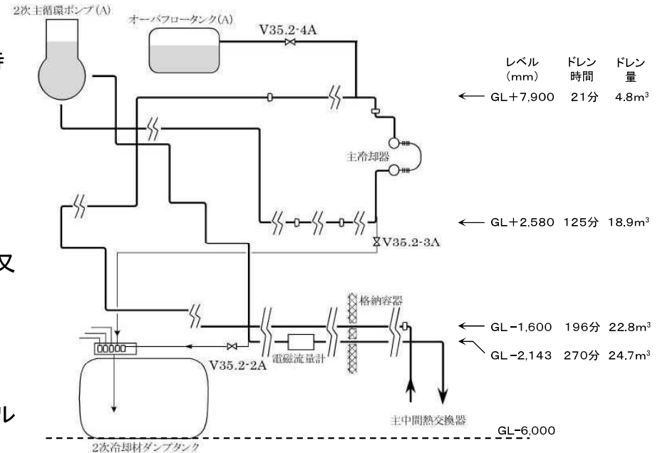
2次系の緊急ドレンに要する時間
