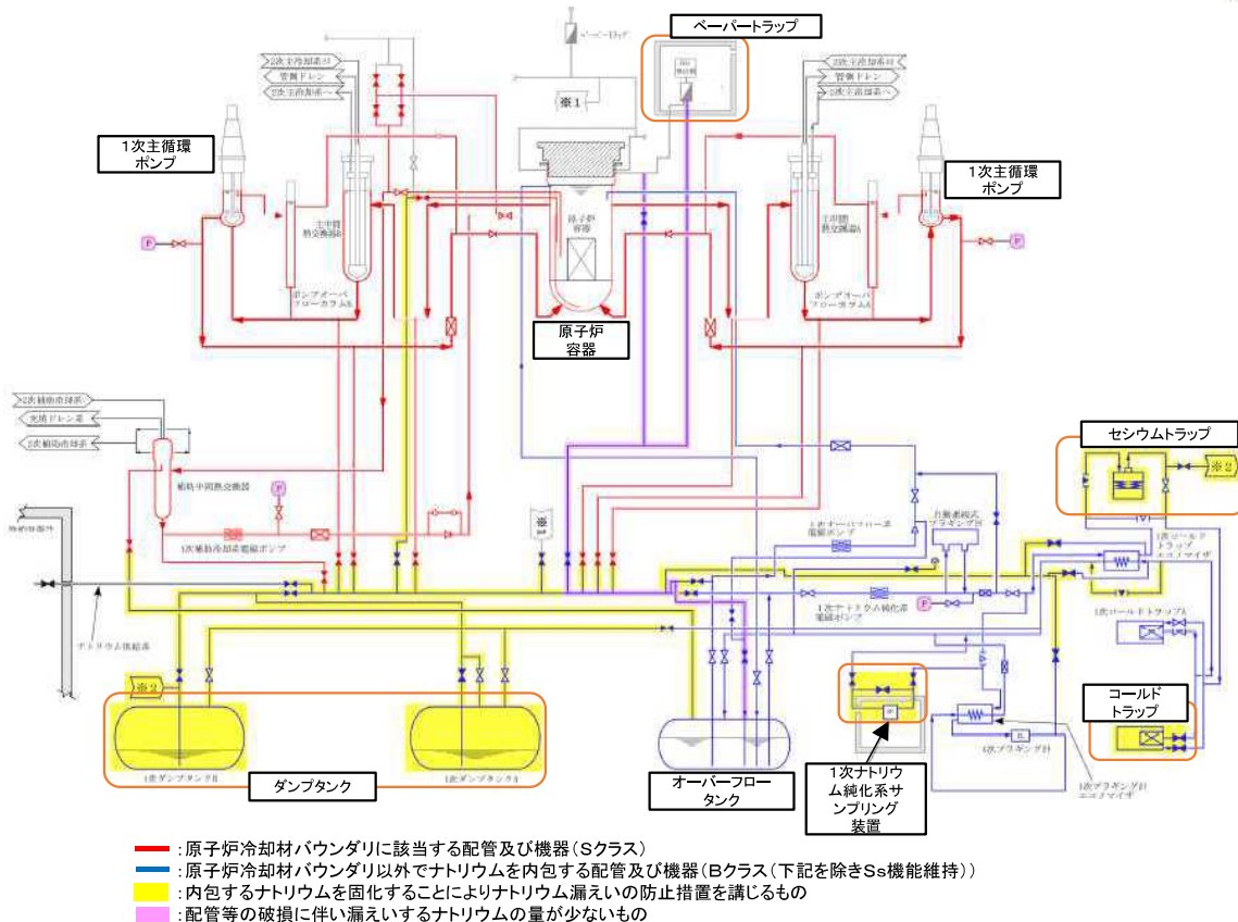
②の例：耐震設計の概念図(1次系)
