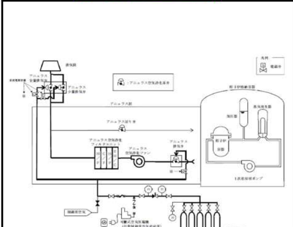
第1.16.5図 室兼ポンベ（代替制御用空気供給用）によるアンニュラス空気浄化設備の運転 概略系統
