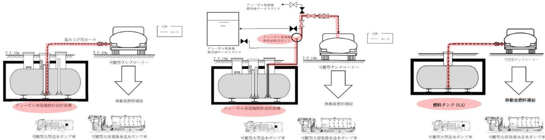
泊3号炉 ディーゼル発電機燃料油貯槽から各設備への補給 （直接汲み上げ時）
