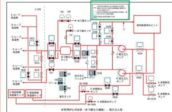
第1図 化学体積制御設備及び非常用炉心冷却系のほう酸注入機能の系統概要図
